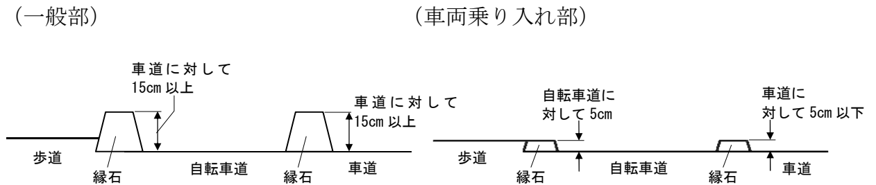
図 II-7 自転車道の断面構造の例
