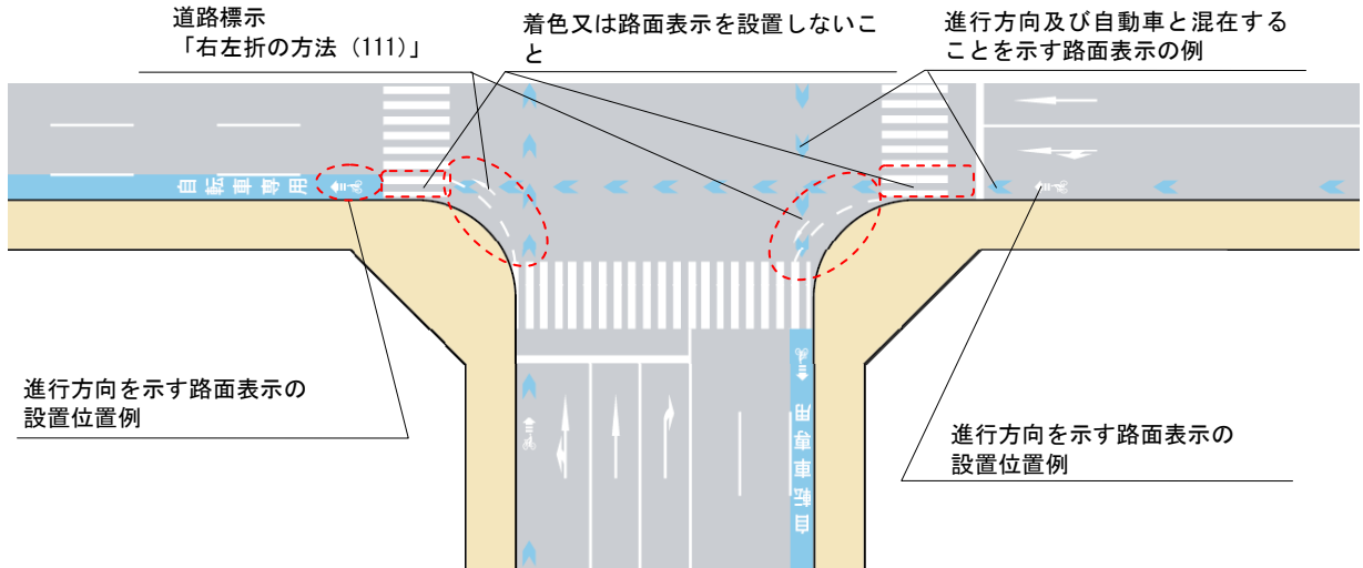
図 II-35 交差点隅角部の道路構造の例（自転車専用通行帯の場合）
