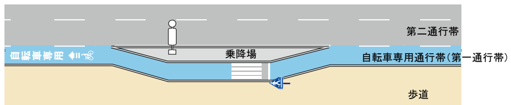
図Ⅱ-19 交通島を設置する例
