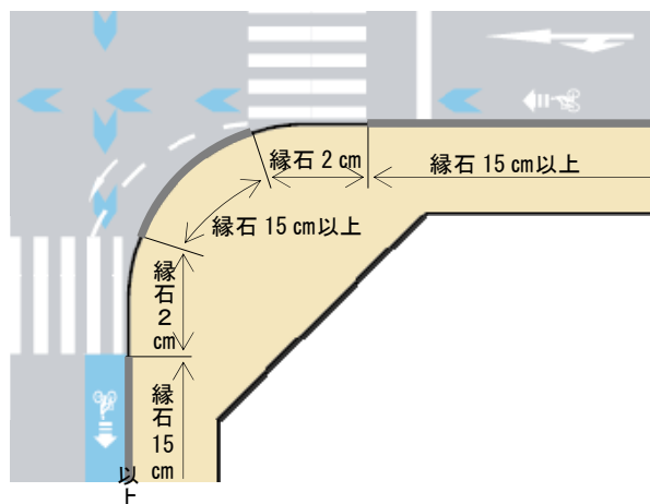
図II-31 交差点隅角部の縁石構造の例 (自転車専用通行帯の場合)
