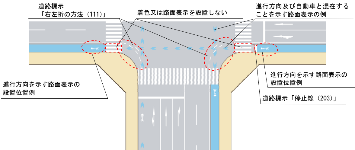
図 II-43 交差点隅角部の道路構造の例
