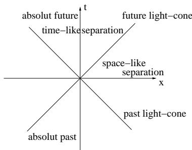
FIG. 3: The light cones.
