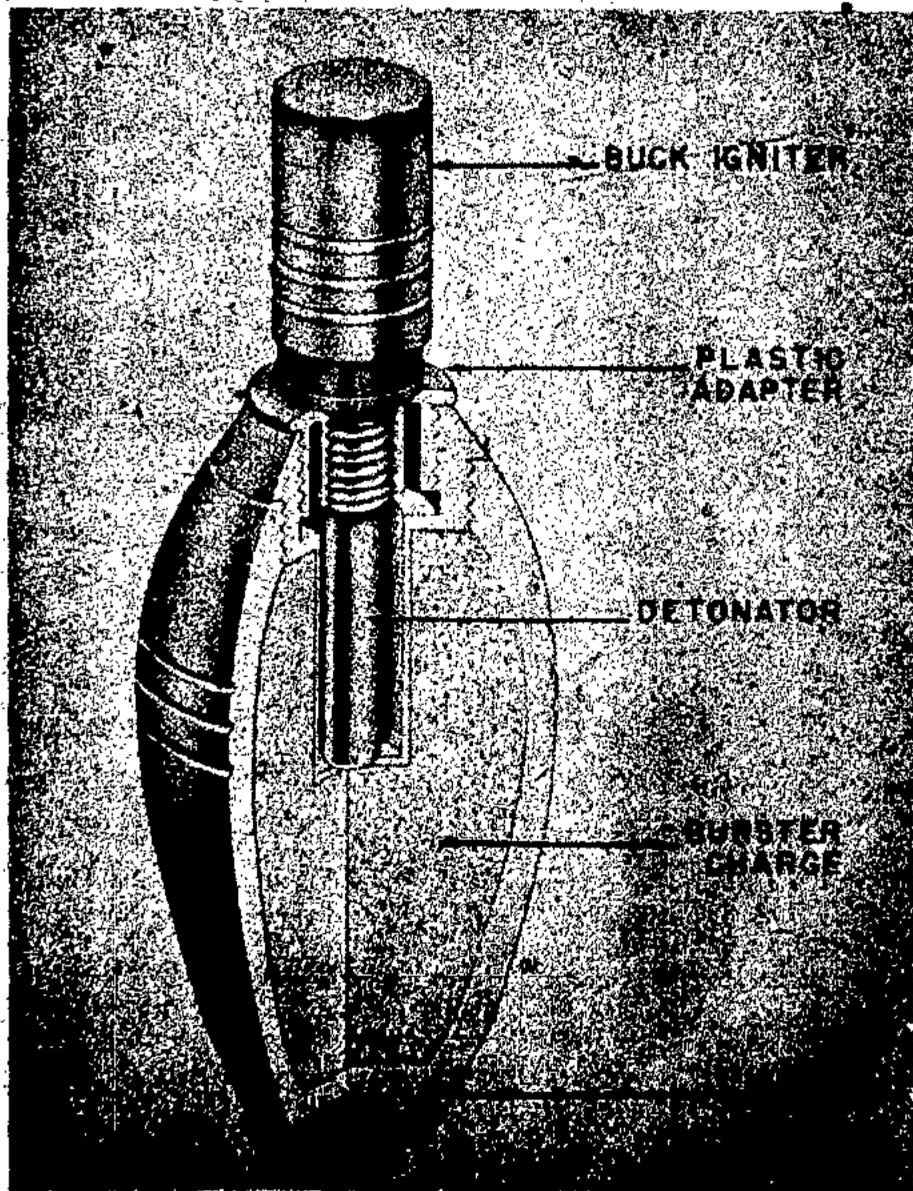
Figure 244—Behelfsmine W-1—Antipersonnel
