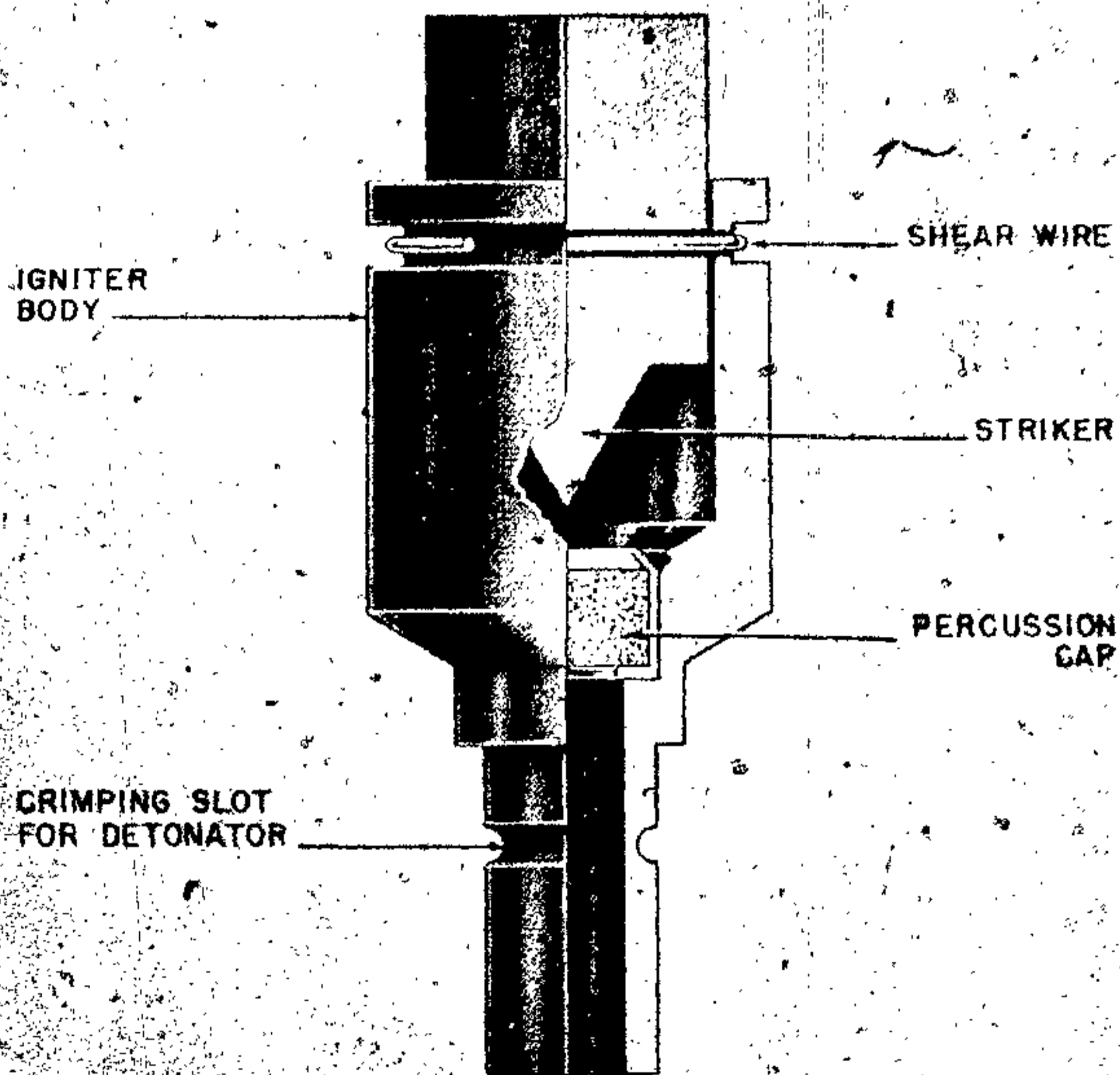
Figure 274—Fi. Es. Mi. Z. Pressure Igniter
