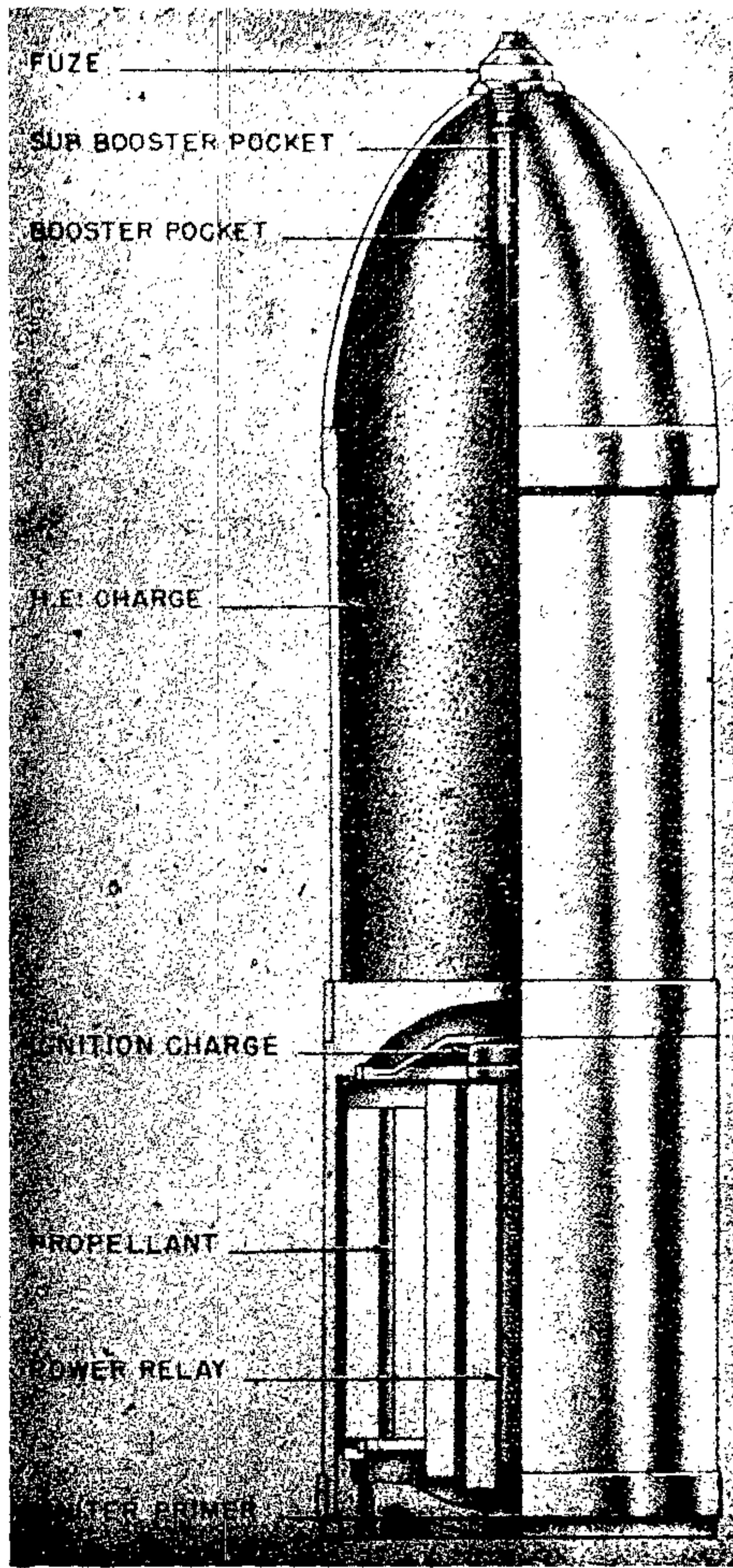
Figure 219—38-cm H. E. Rocket
