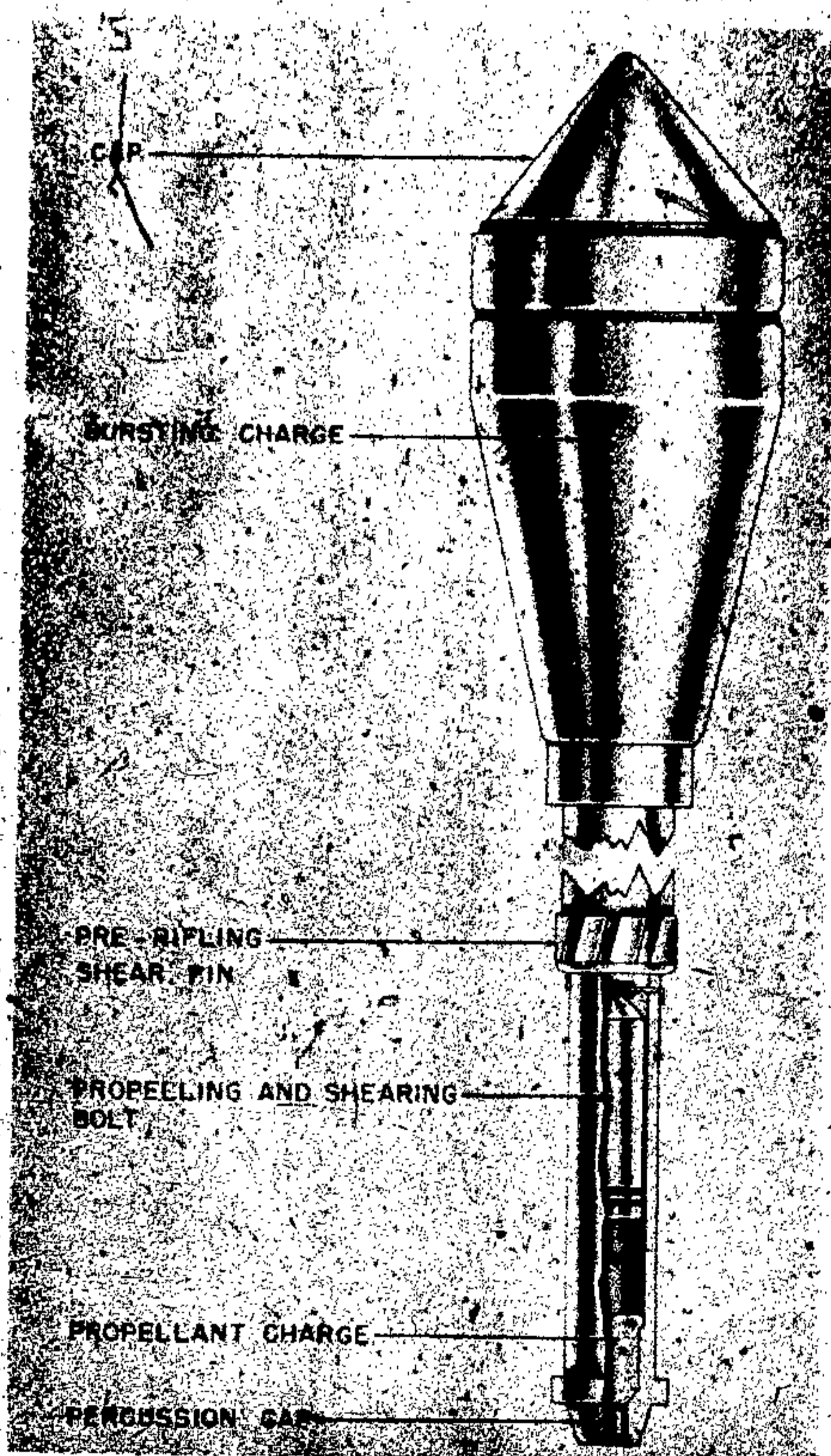
Figure 313—Pz. W. K. 42 L. P. Hollow Charge Pistol Grenade
