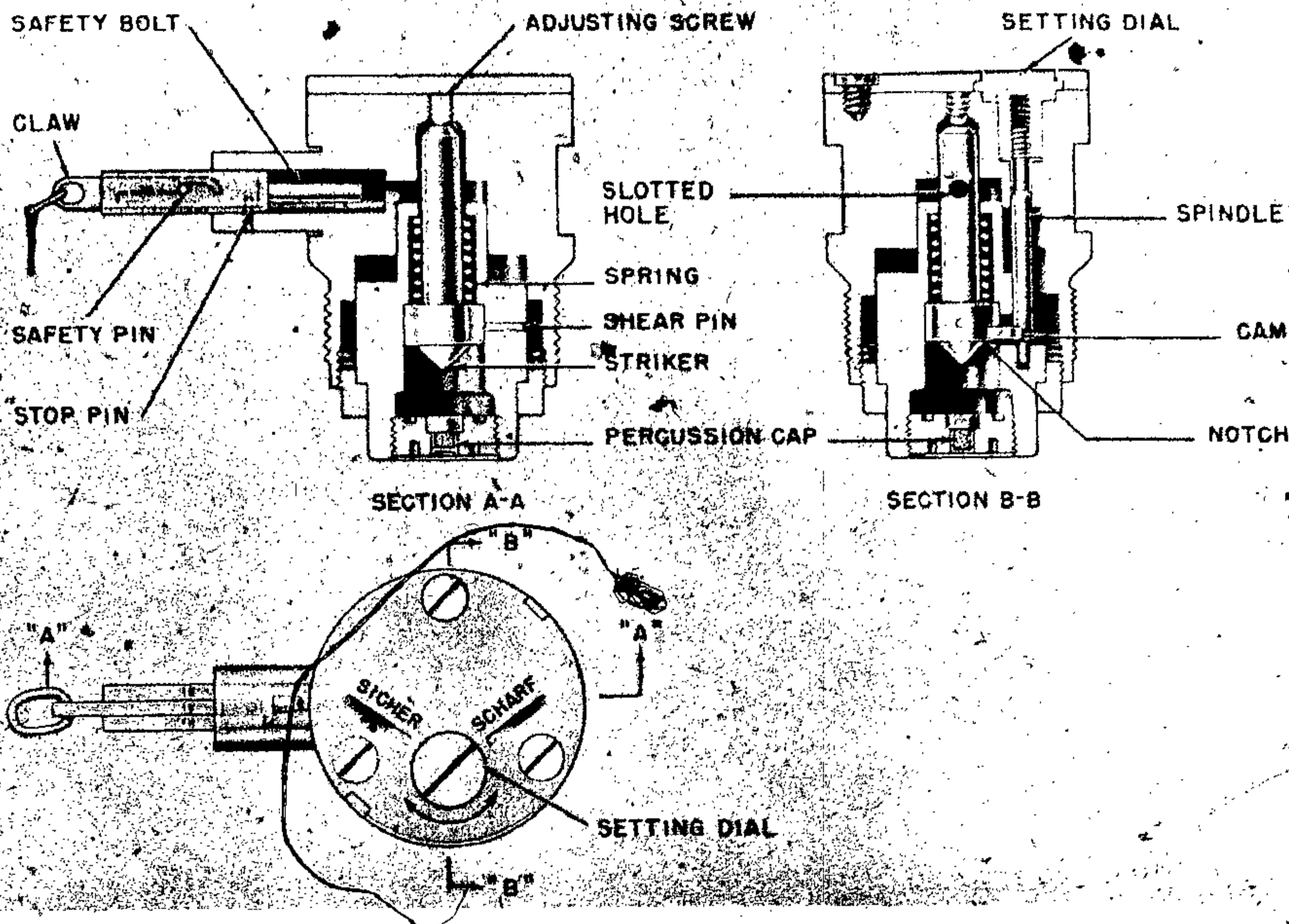
Figure 269—T. Mi. Z. 35 Pressure Igniter
