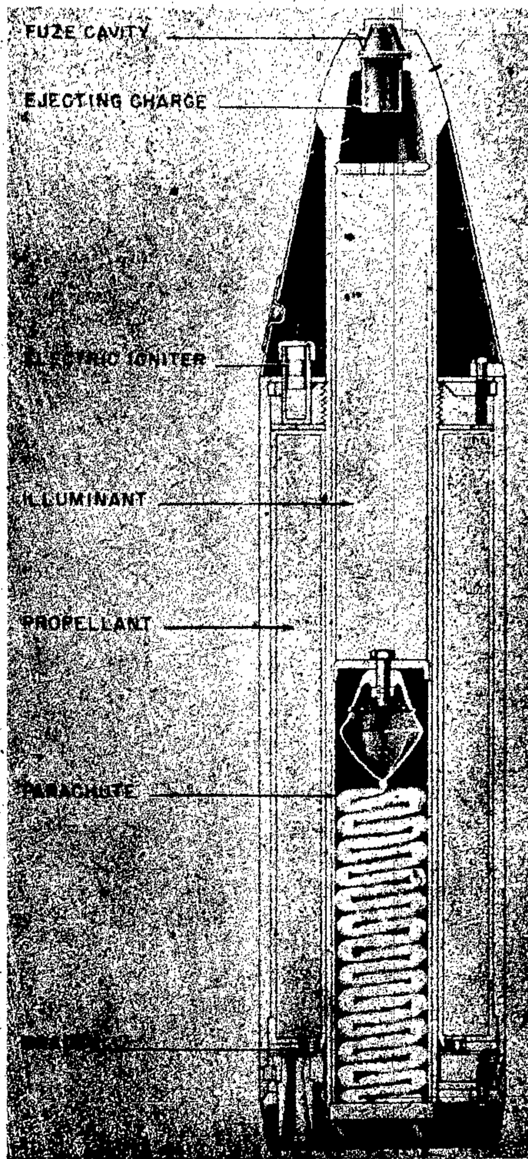
Figure 223—21-cm R-Lg Rocket
