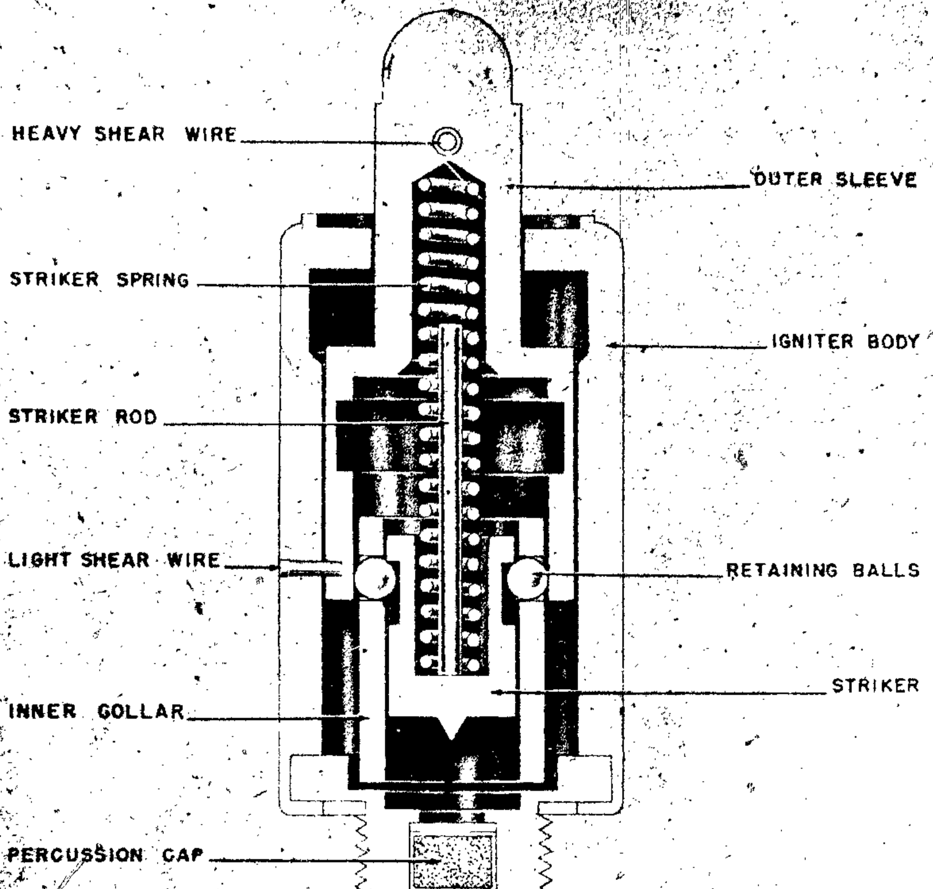
Figure 271—T. Mi. Z. 43 Pressure Igniter
