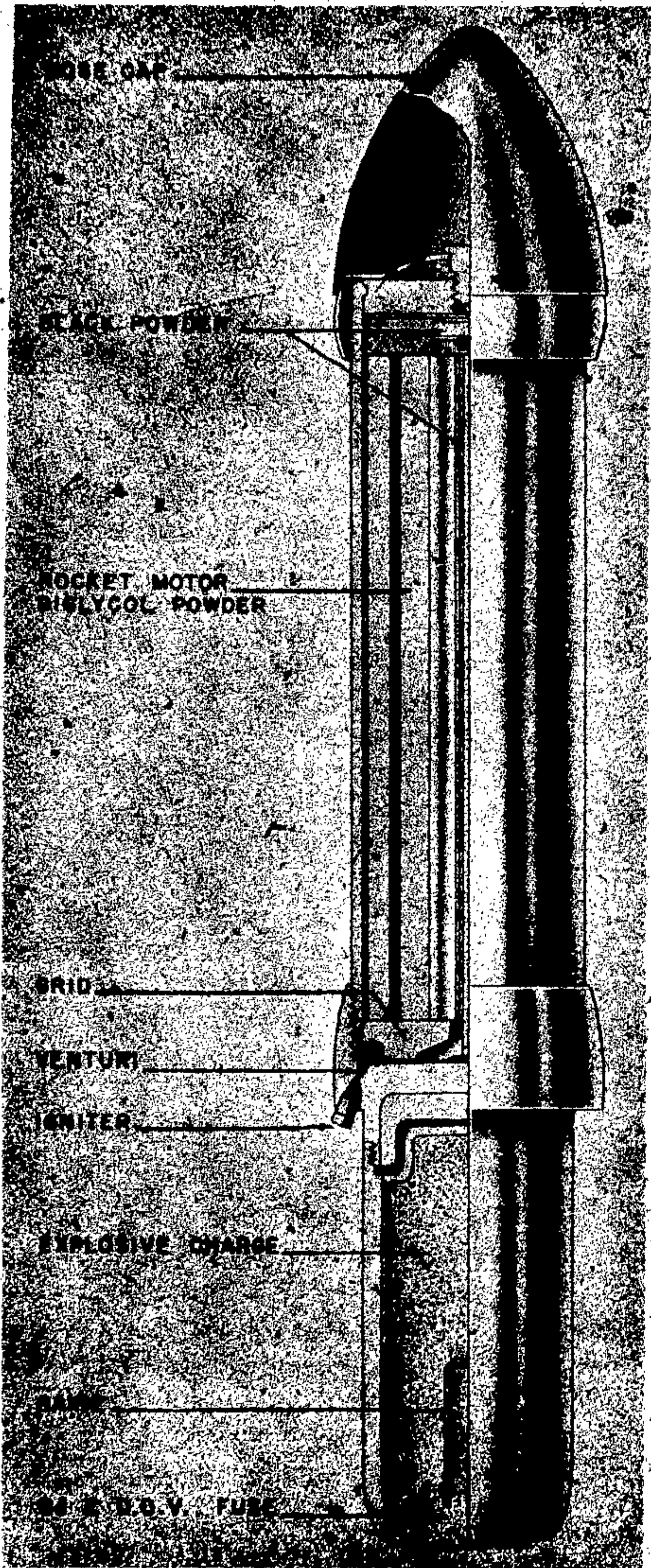
Figure 211—15-cm H. E. Rocket
