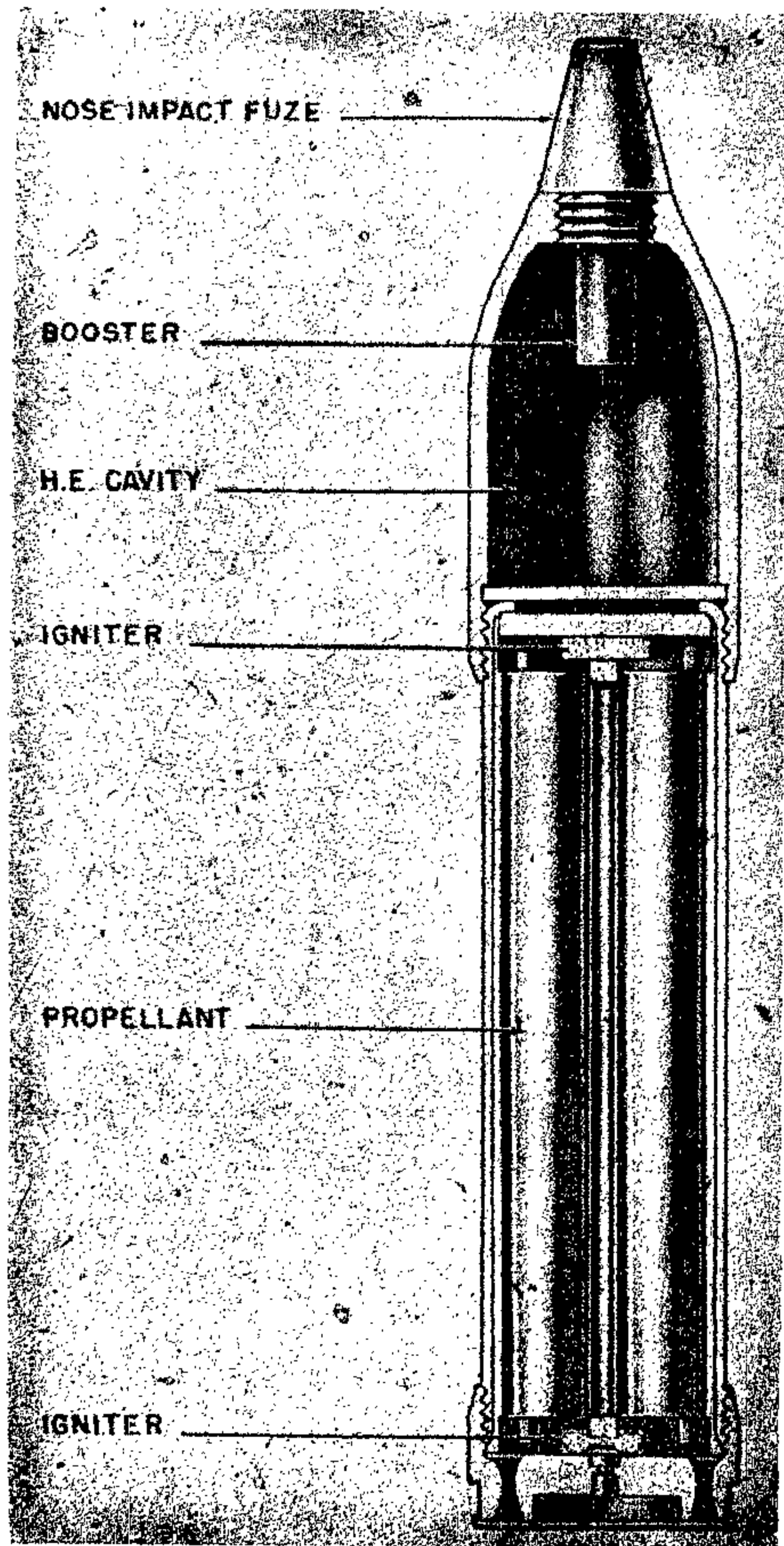
Figure 221—8.6-cm R. Spgr L/5.5 Rocket
