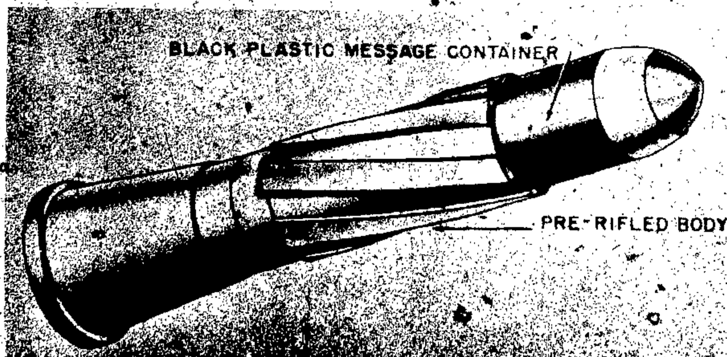
Figure 314—27-mm Message Pistol Grenade
