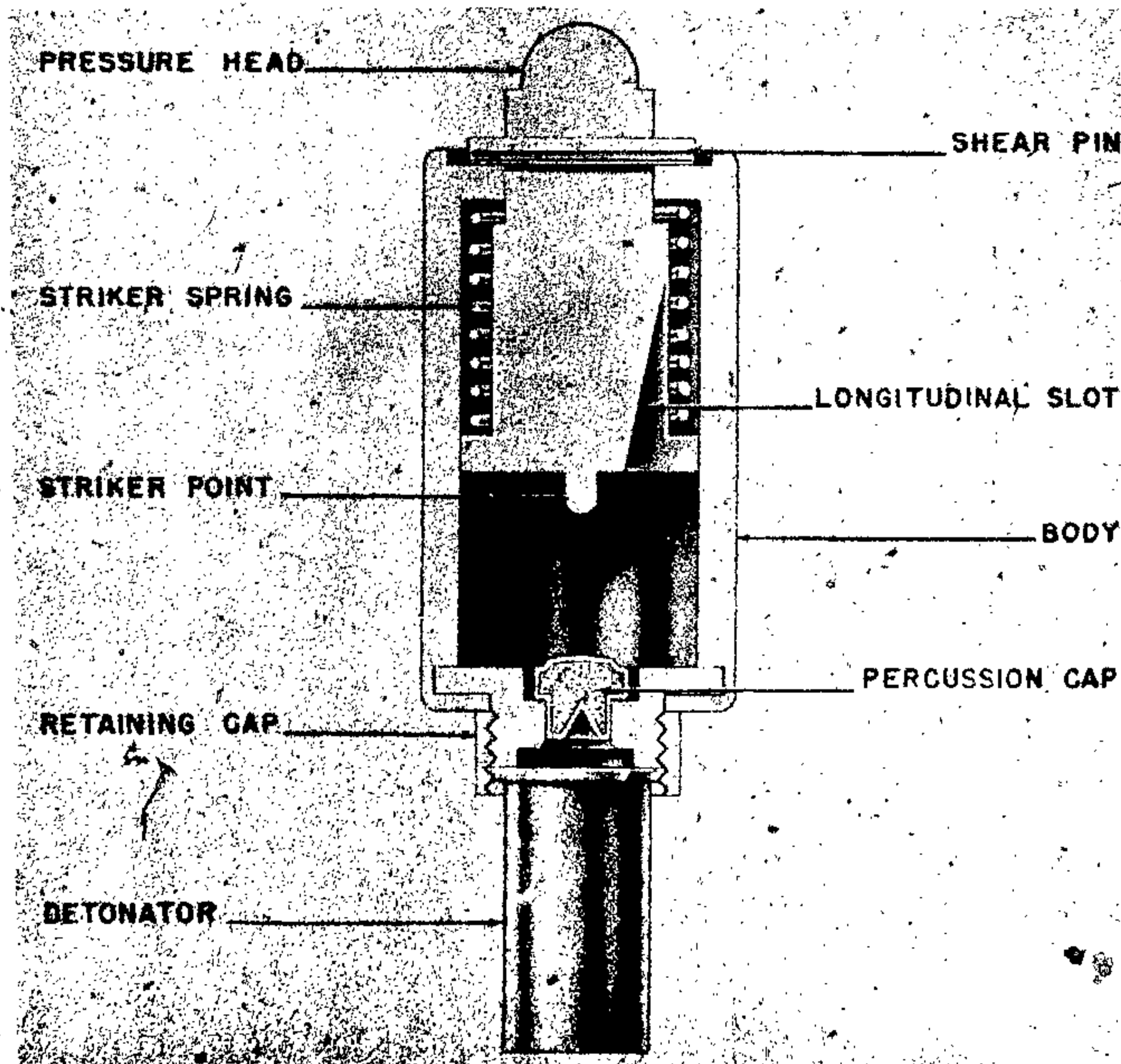
Figure 270—T. Mi. Z. 42 Pressure Igniter
