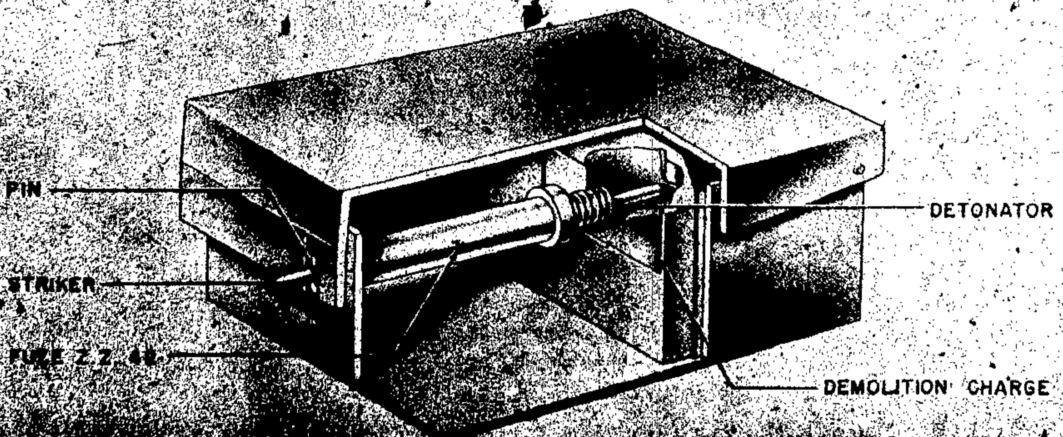
Figure 243—Schumine 42—Antipersonnel
