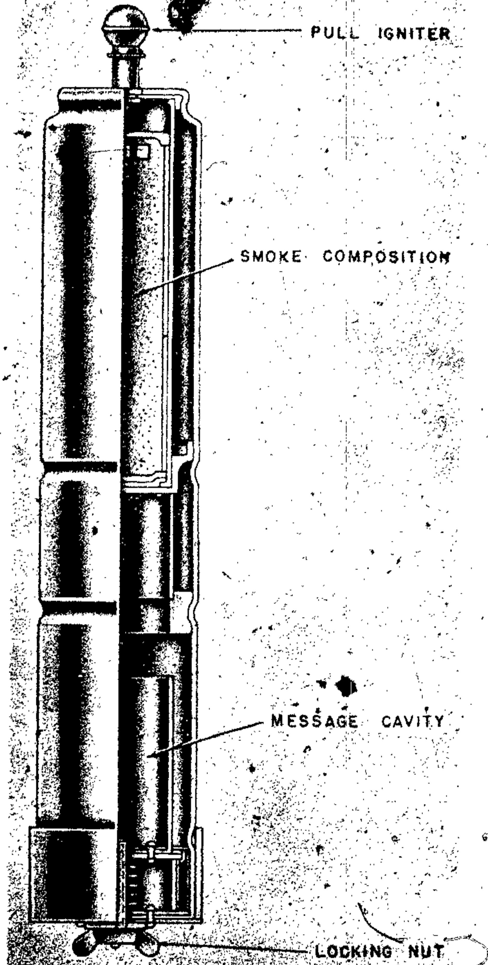
Figure 118—Message Tube (land)
