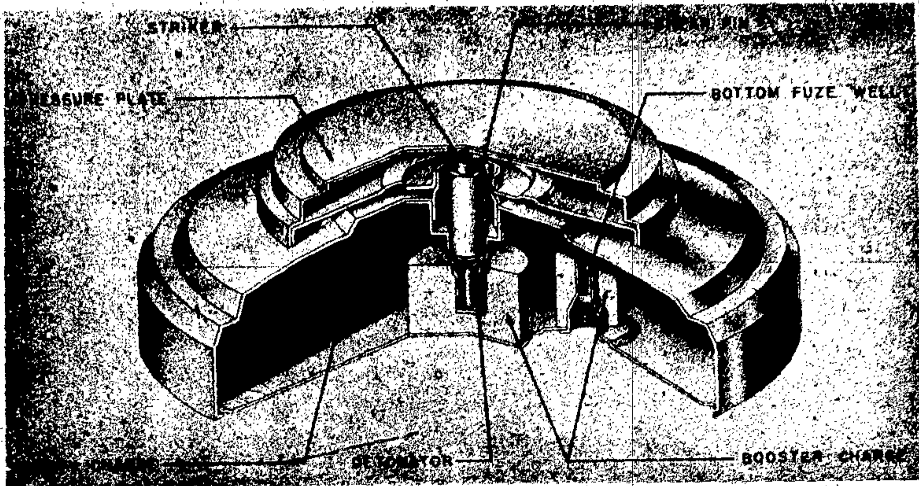
Figur 233—Tellermine 43—Antitank
