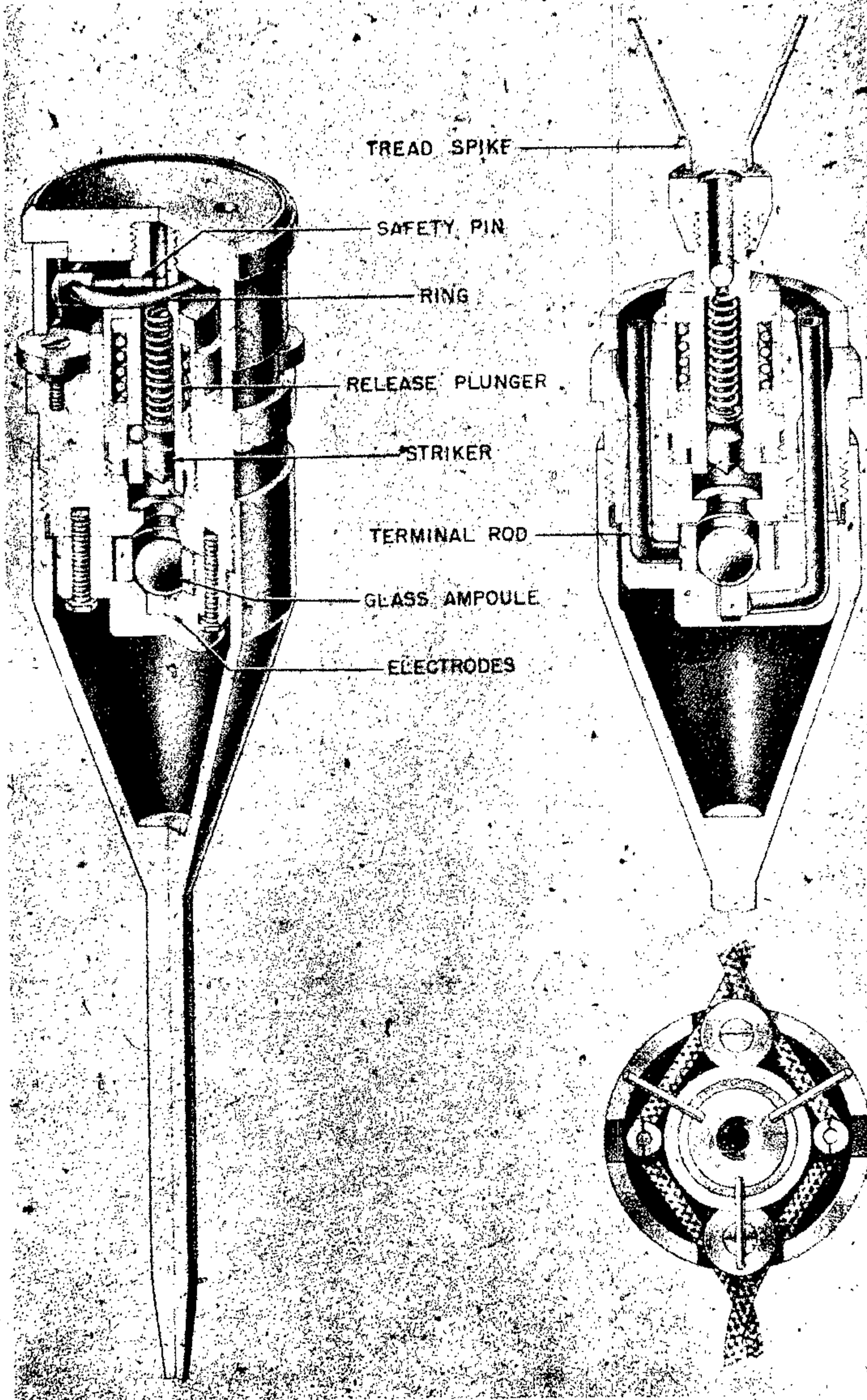
Figure 268—E. S. Mi. Z. 40 Pressure Igniter (Electric)
