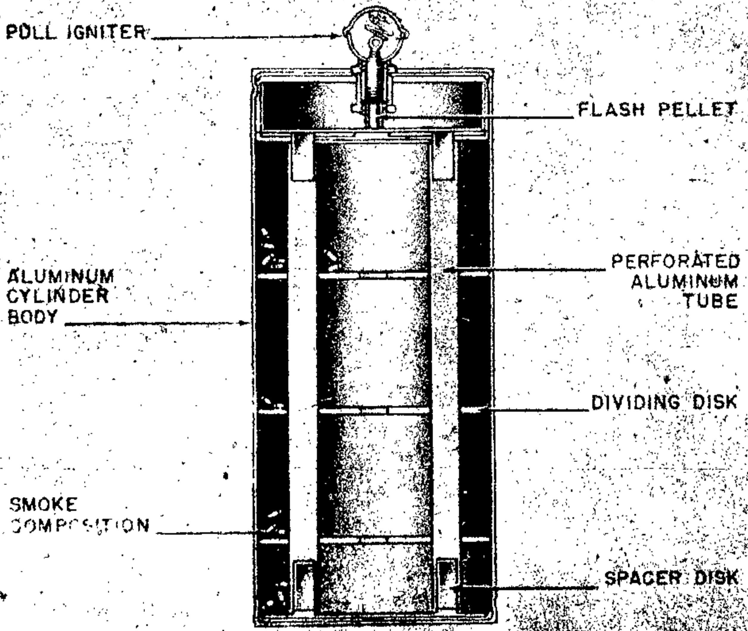
Figure 84—Smoke Signal Flare A. R. D. R.
