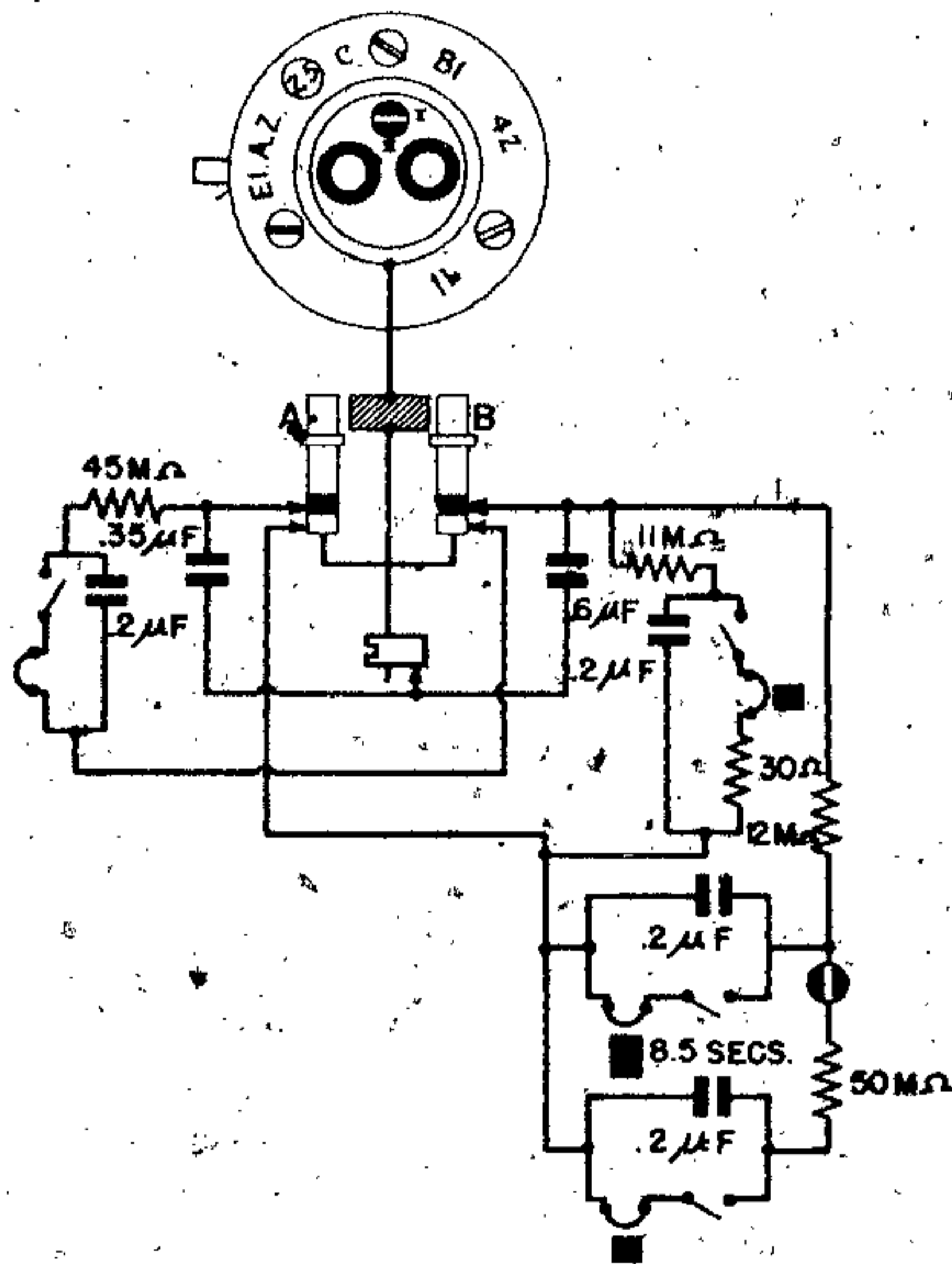
Figure 142—(25)C Electrical Impact Fuze
