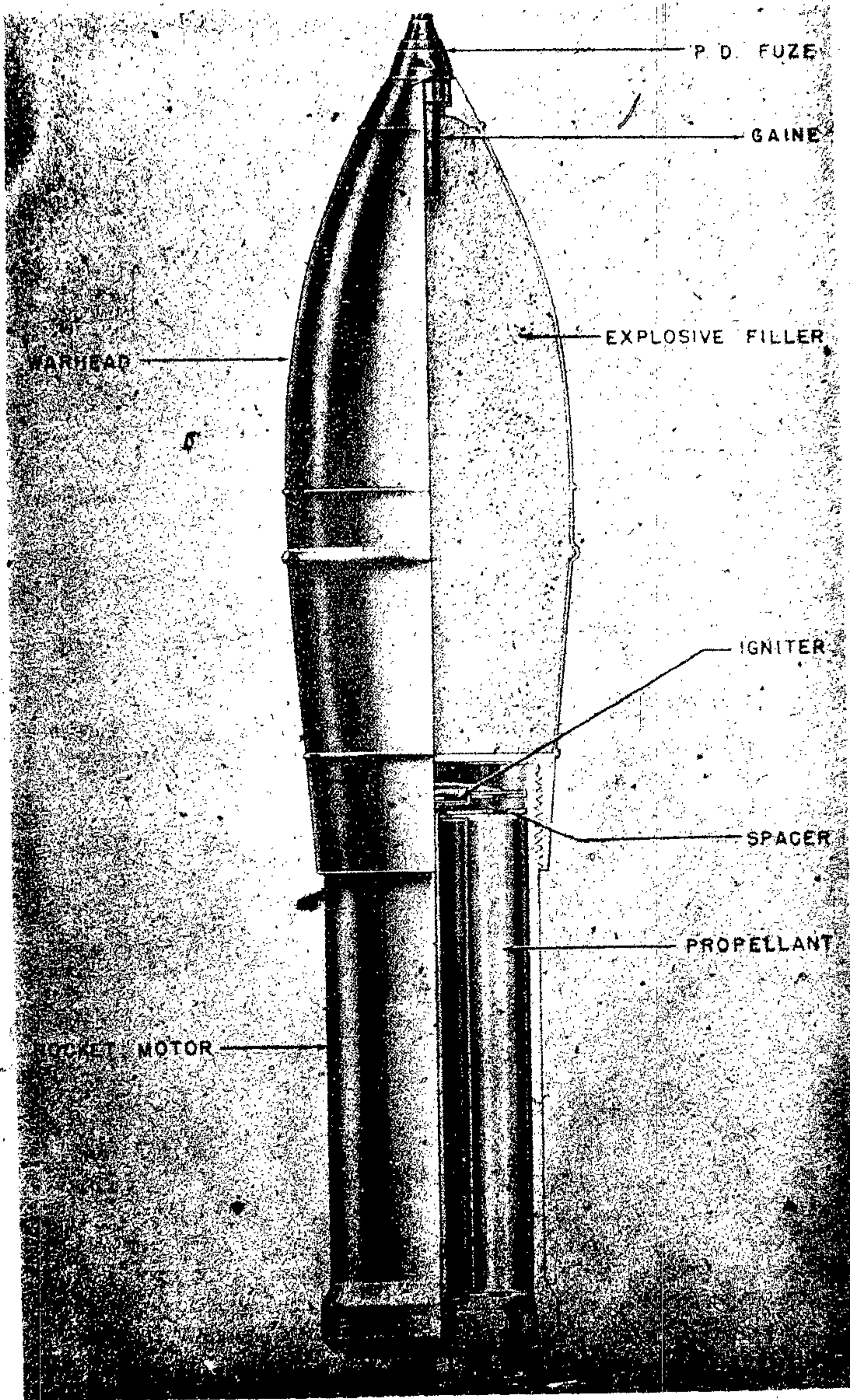
Figure 217—30-cm H. E. Rocket
