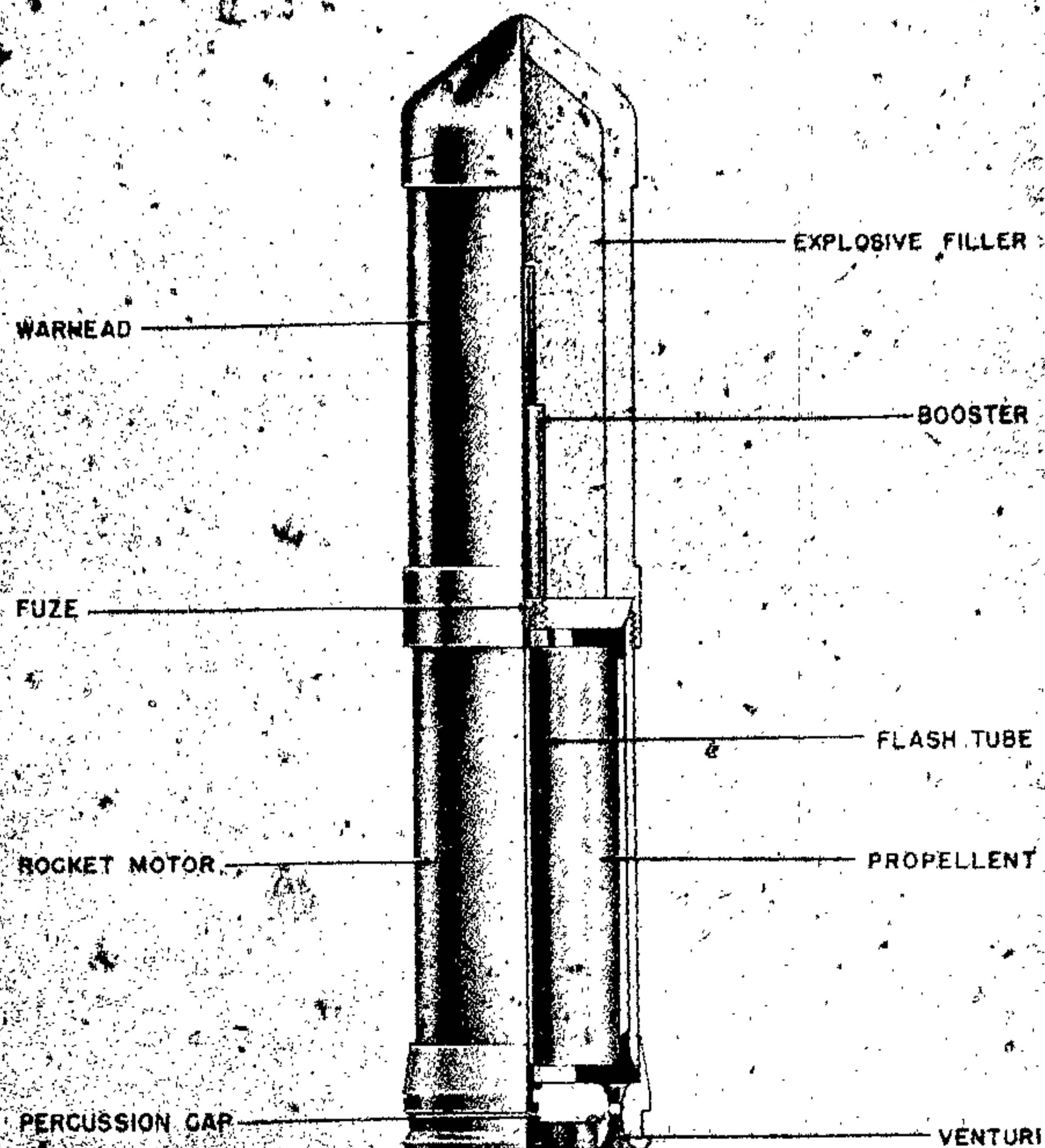
Figure 207—8.6-cm H. E. Rocket (Naval)
