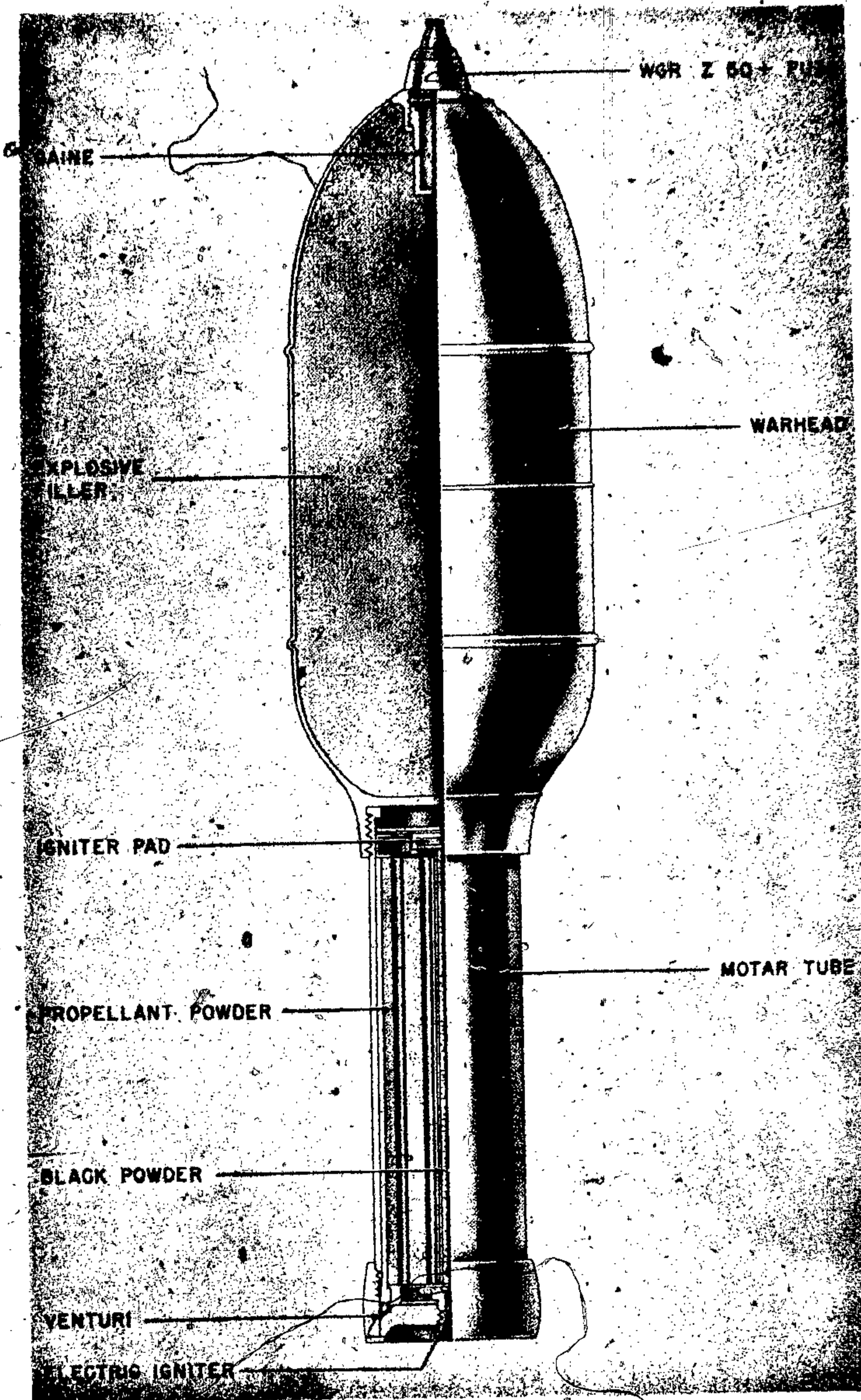
Figure 216—28-cm H. E. Rocket
