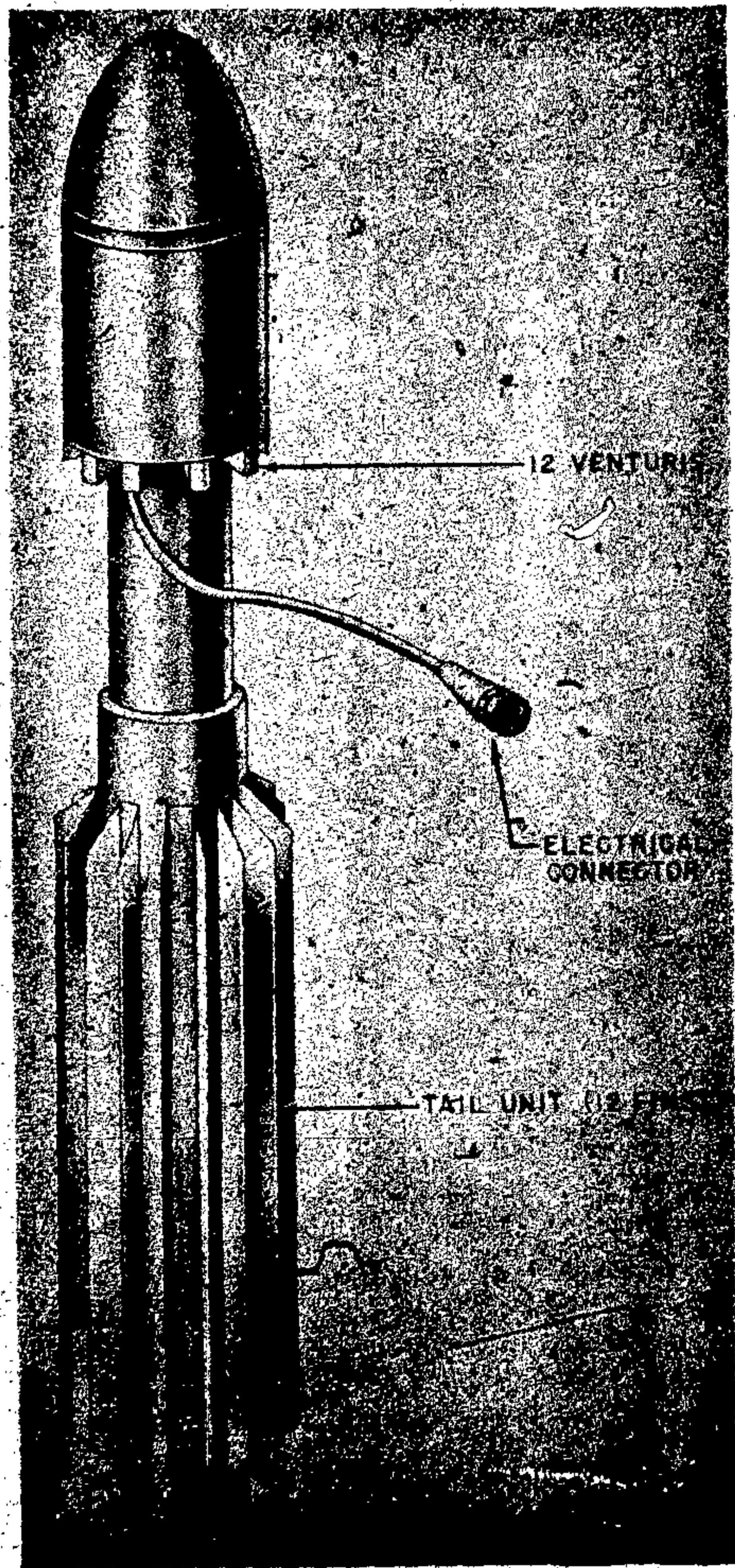
Figure 214—20-cm Antiaircraft Rocket
