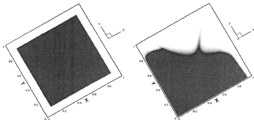
Рис. 3. Оседание квадратного облака частиц. Слева изображена начальная концентрация примеси, справа - концентрация примеси в момент времени t = 0.314 при A = 600 .
