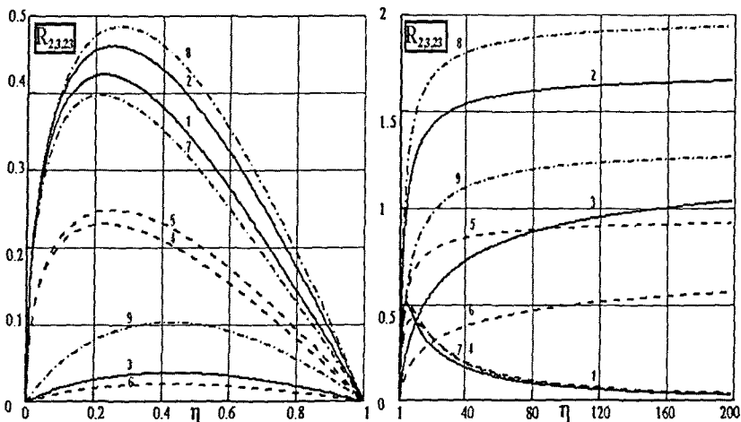
Рис. 1 Величины R_2 , R_3 и R_{23} в зависимости от отношения плотностей фаз \eta при \omega_1 = 1 (сплошная линия), \omega_1 = 0.1 (штрихованная линия) и \omega_1 = 10 (штрих-пунктир). Кривые 1, 4, 7 показывают влияние силы Бассэ ( R_3 ), 2, 5, 8 - суммарное влияние нестационарных и наследственных сил ( R_{23} ), а 3, 6, 9 - влияние силы присоединенных масс ( R_2 ).
