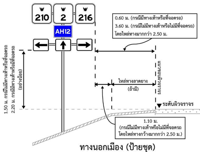
รูปที่ 1-1 มาตรฐานระยะการติดตั้งป้ายจราจรบนทางหลวงทั่วไป (ในเมืองและนอกเมือง)
