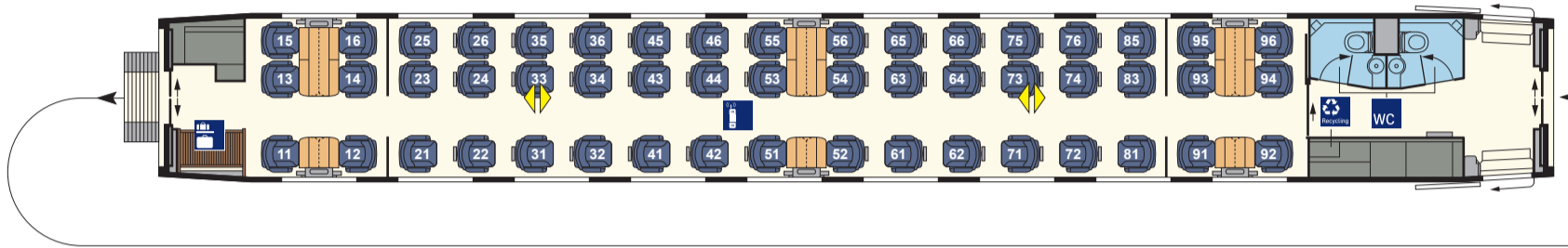
1. Kl.-Wagen (Apmz 407.1) Nr. 28/38
