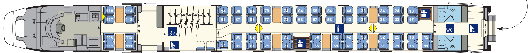
2. Kl.-Endwagen (Bpmdzf 5812.0) Nr. 1
