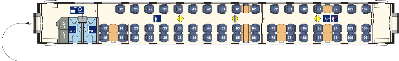
1. Kl.-Wagen (Apmz 805.3) Nr. 27/37
