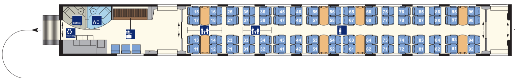
2. Kl.-Wagen (Bpmz 411.8) Nr. 24/34
