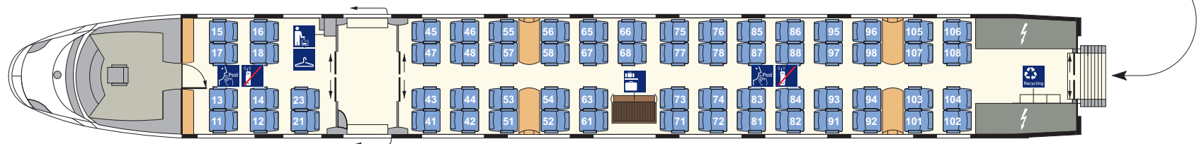
2. Kl.-Endwagen (Bpmzf 406.5) Nr. 21/31
