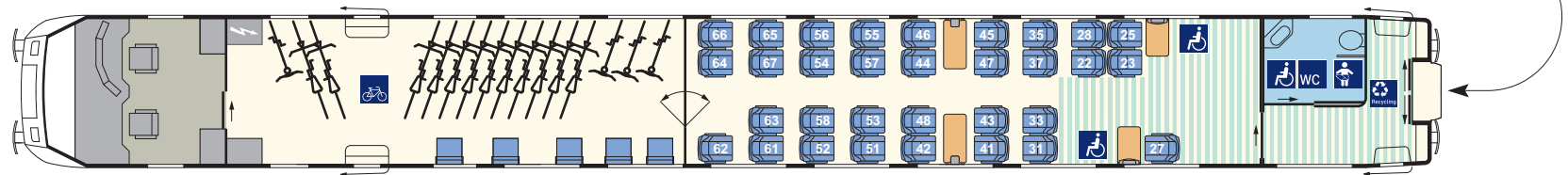
2. Kl.-Steuerwagen (Bpmmbdzf 286)
