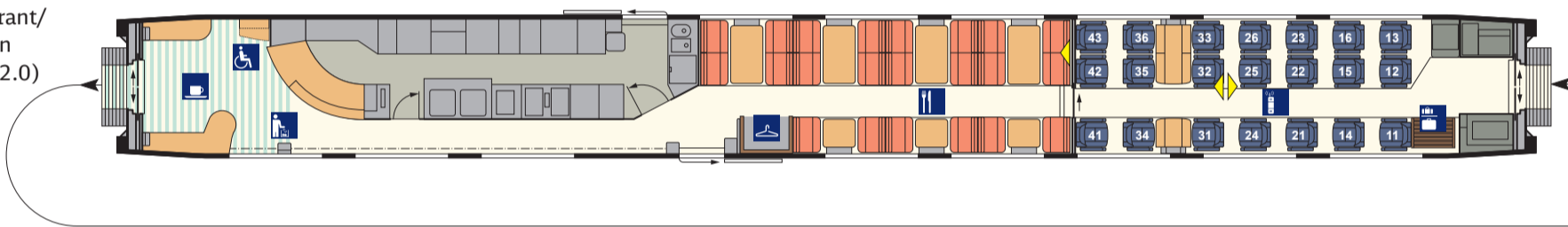
2. Kl.-Wagen (Bpmbsz 6412.0) Nr. 9
