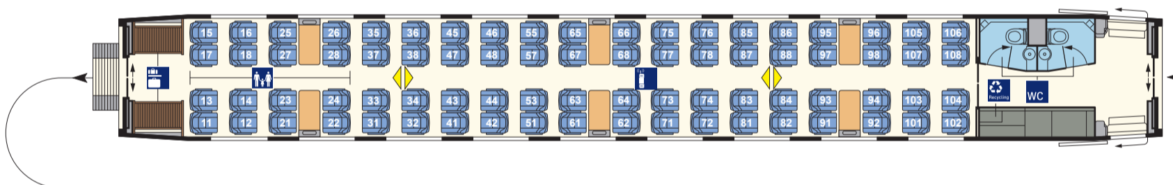
2. Kl.-Wagen (Bpmz 407.3) Nr. 24/34
