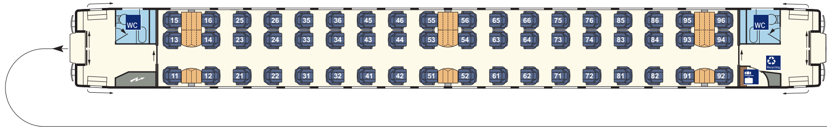
1. Kl.-Wagen (Apmmz 126)
