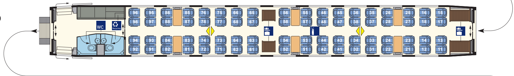
2. Kl.-Wagen (Bpmz 407.6) Nr. 22/32
