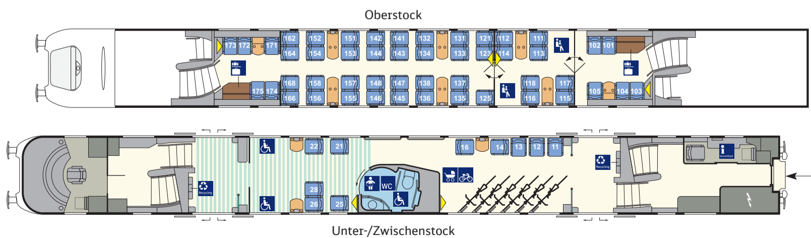
2. Kl.-Steuerwagen (DBpbzfa 668.2) Nr. 1
