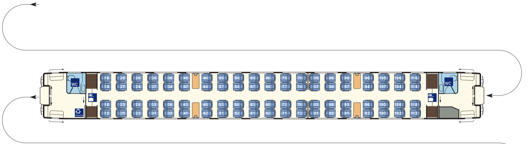
2. Kl.-Wagen (Bpmmz 284)
