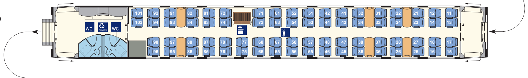
2. Kl.-Wagen (Bpmz 406.6) Nr. 22/32
