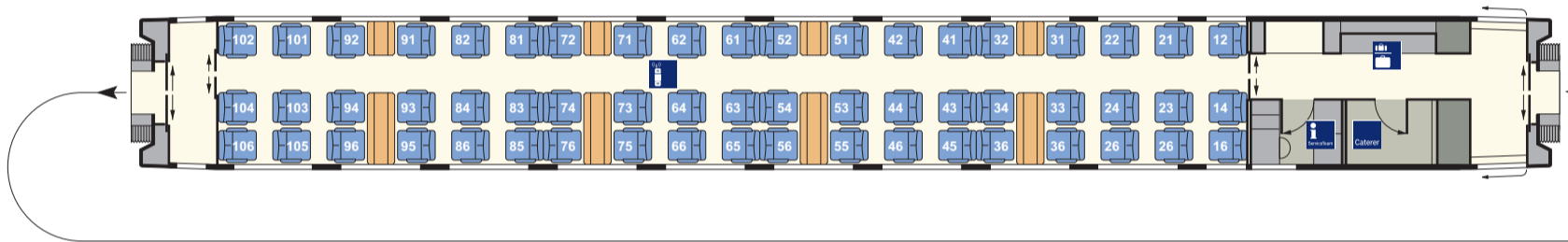
2. Kl.-Wagen (Apmz 116.4) Nr. 4
