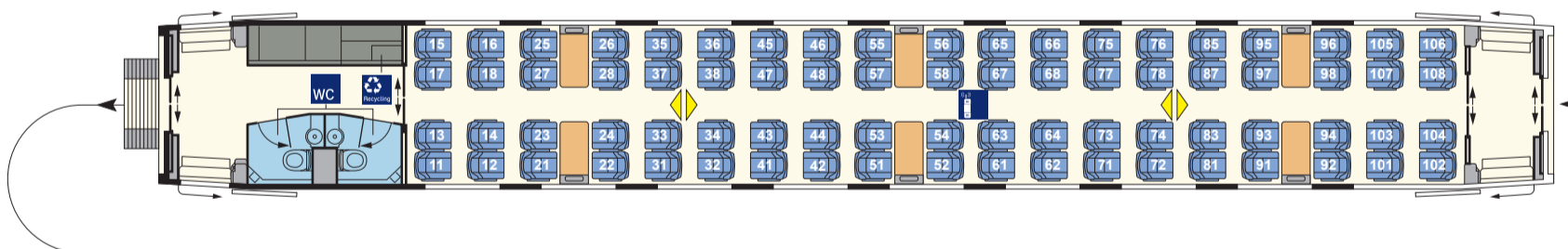
2. Kl.-Wagen (Bpmz 407.7) Nr. 23/33
