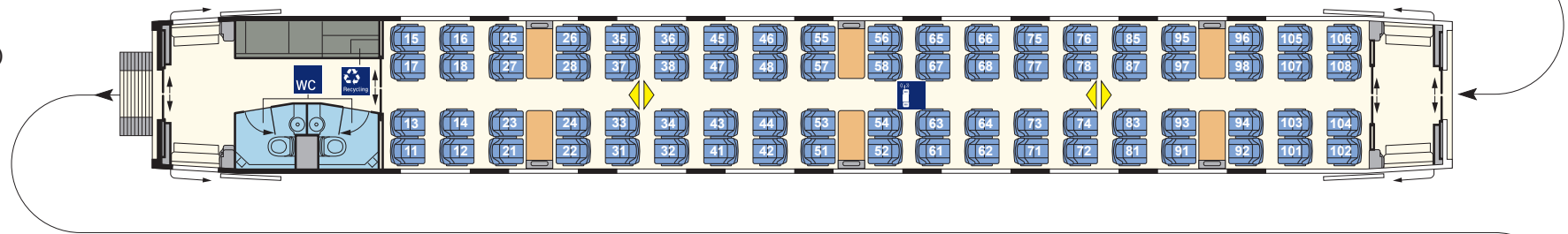
2. Kl.-Wagen (Bpmz 407.7) Nr. 23/33
