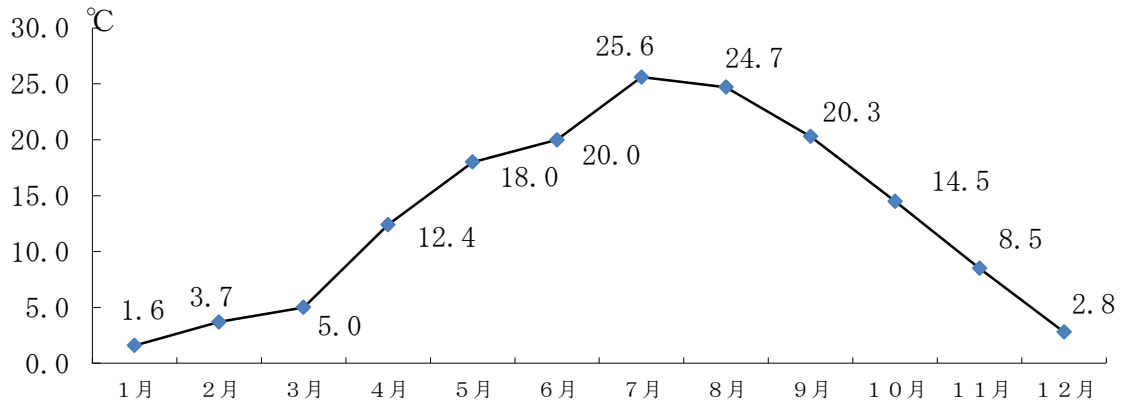
(8) 月別降水量(平成29年)
