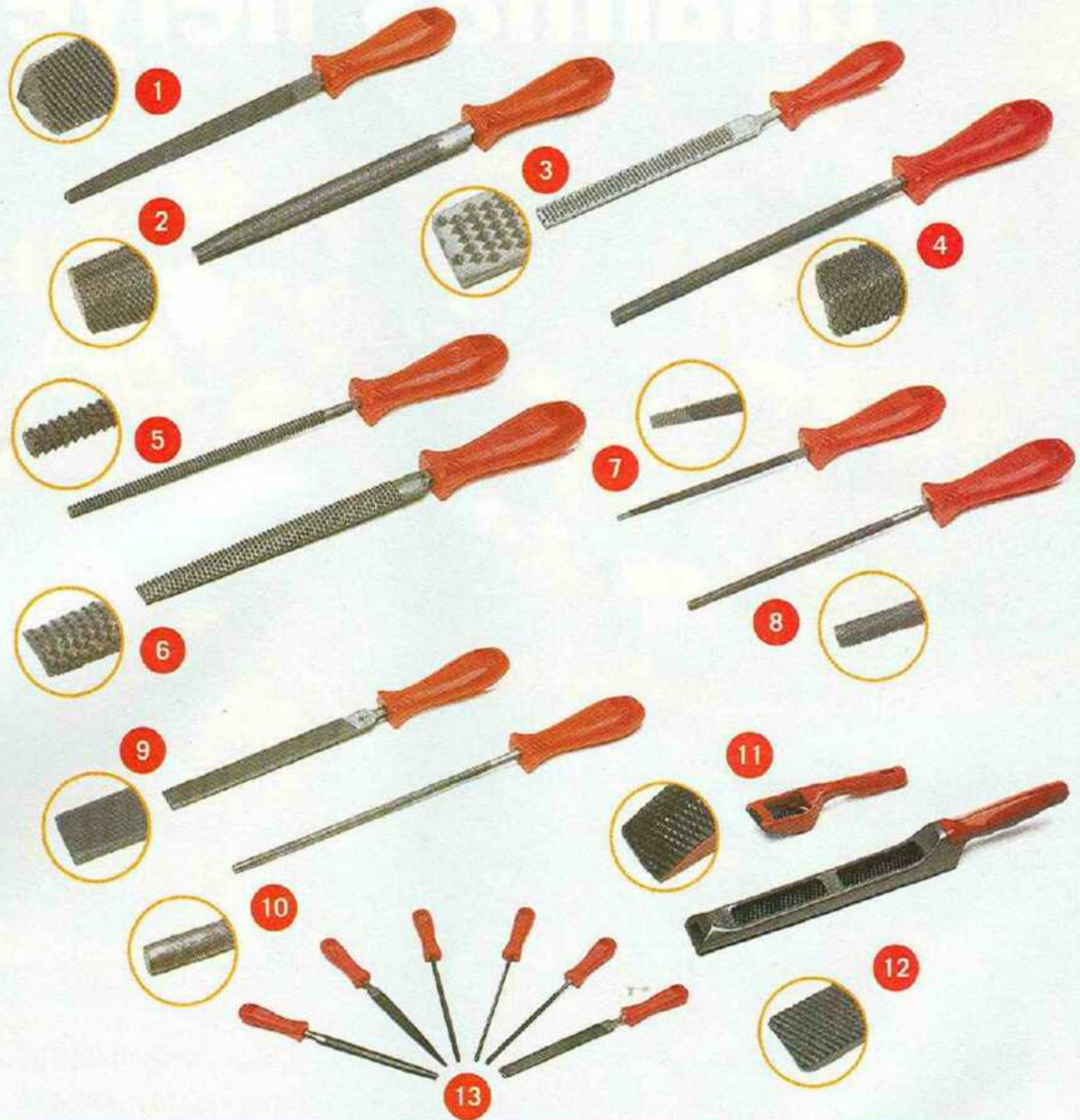
Egyszeres vágású reszelő.
