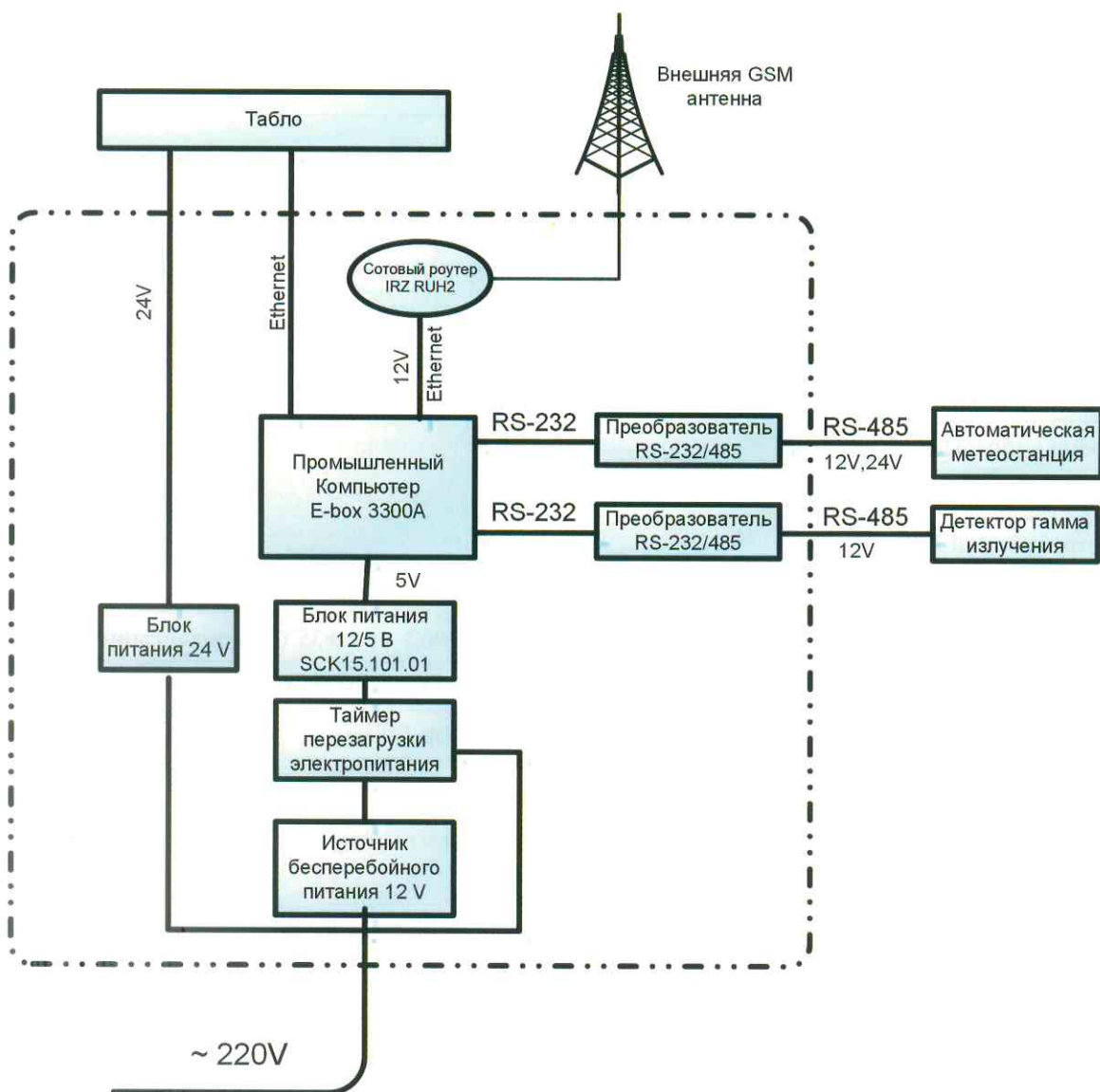
Рис. 4. Структурная схема блока БОП-ИТА (ТЕ)
