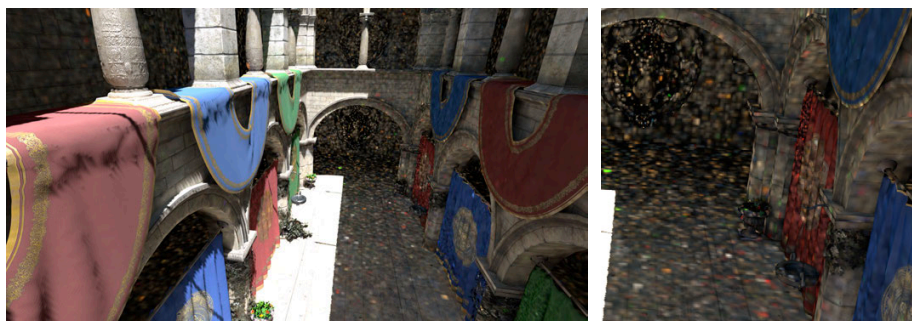
(d) PMJ-02 sample sequence [69]
