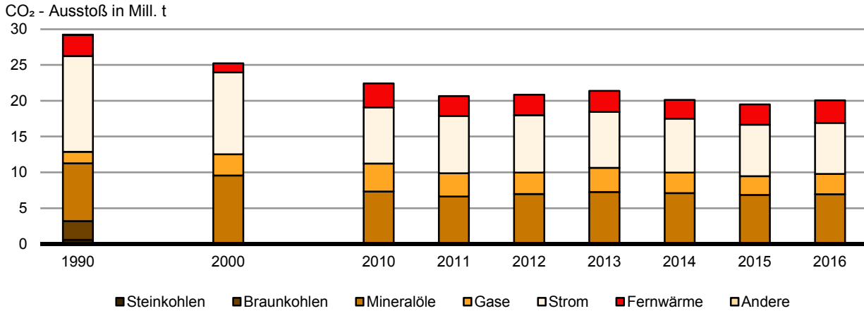
Kohlenstoffdioxid-Emissionen nach Energieträgern (Verursacherbilanz) 1990, 2000, 2010 bis 2016
