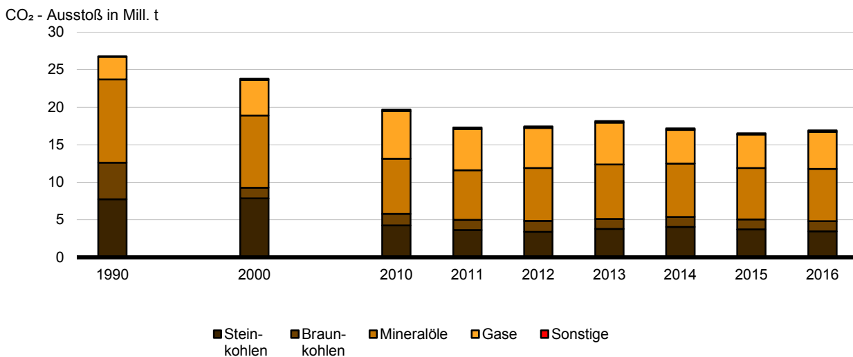
CO 2 -Emissionen nach Energieträgern (Quellenbilanz) 1990, 2000, 2010 bis 2016
