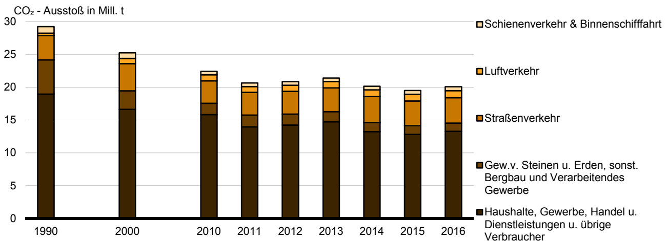
Kohlenstoffdioxid-Ausstoß nach Emittenten-Sektoren (Verursacherbilanz) 1990, 2000, 2010 bis 2016
