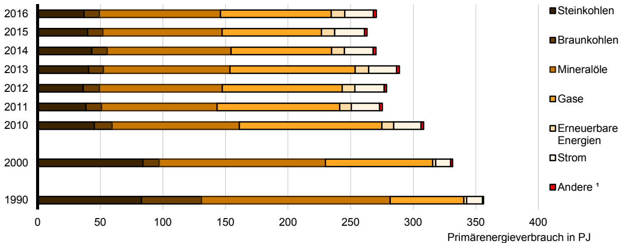
Primärenergieverbrauch nach Energieträgern im Land Berlin 1990, 2000, 2010 bis 2016
