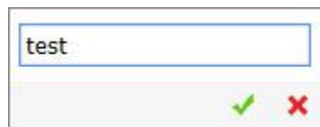
图 4-23 添加组
