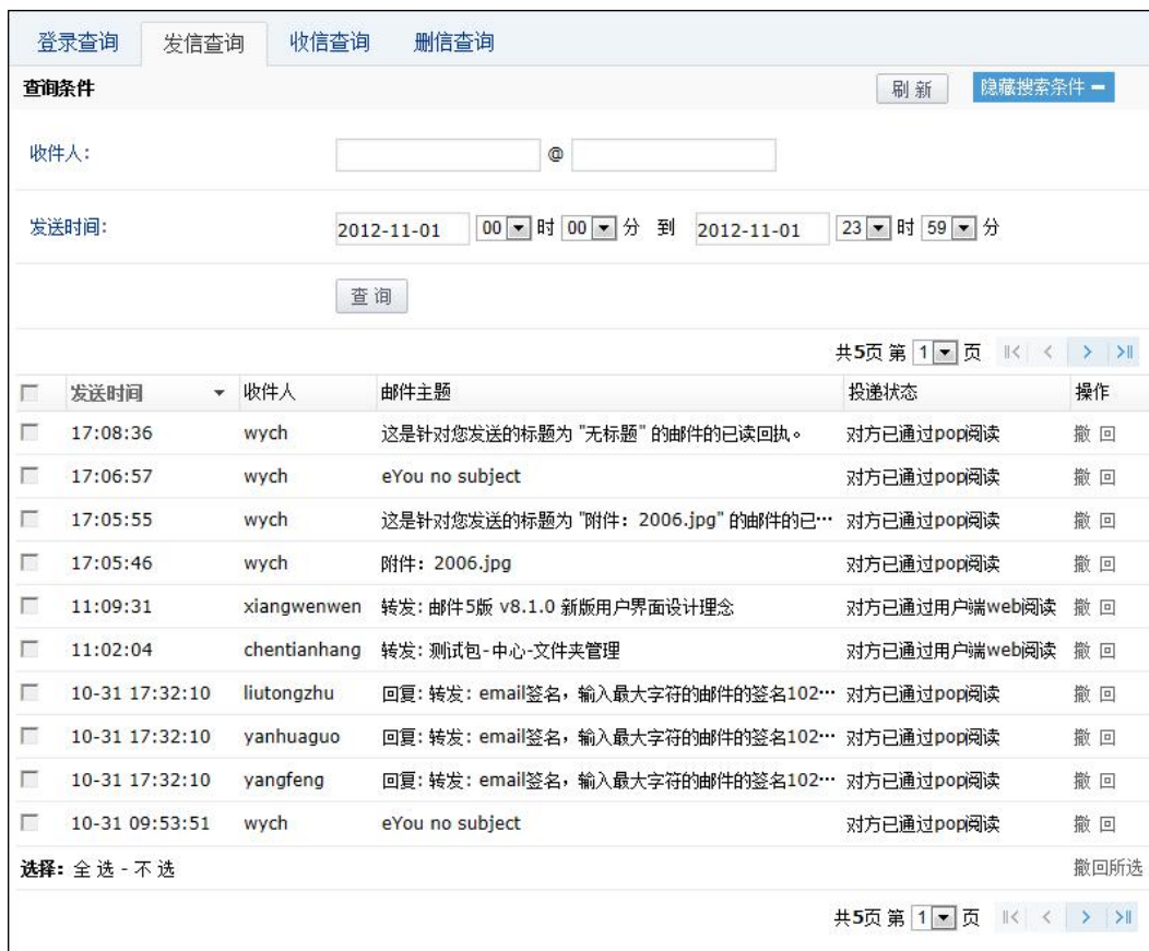
图 4-36 发信查询
