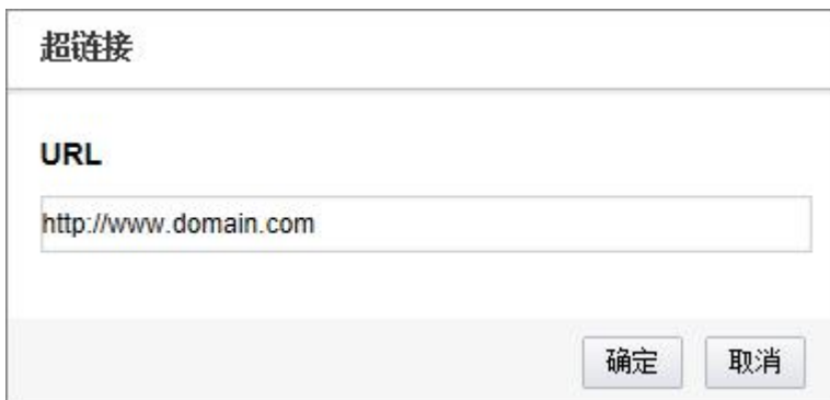
图 4-7 超链接
