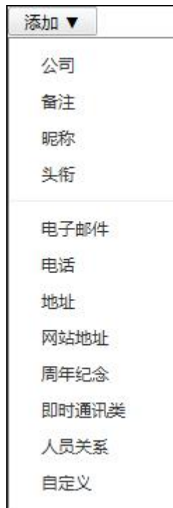
图 4-26 添加信息
