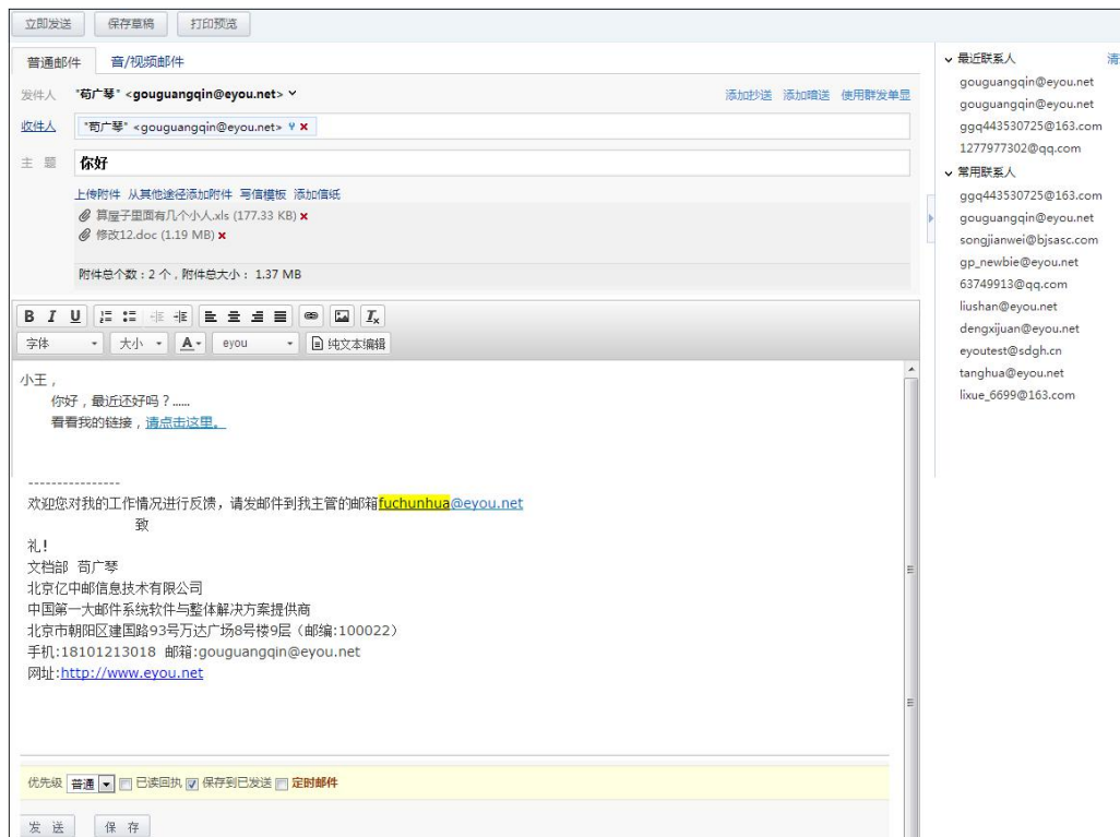
图 4-1 普通邮件
