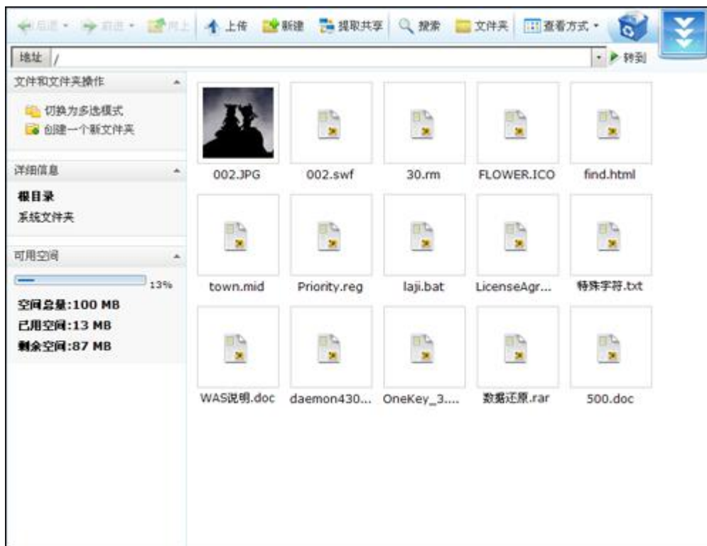
图 4-45 网盘
