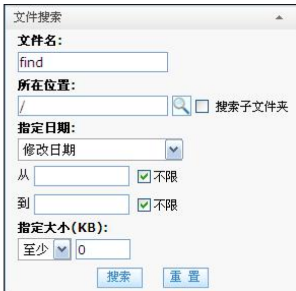
图 4-49 文件搜索
