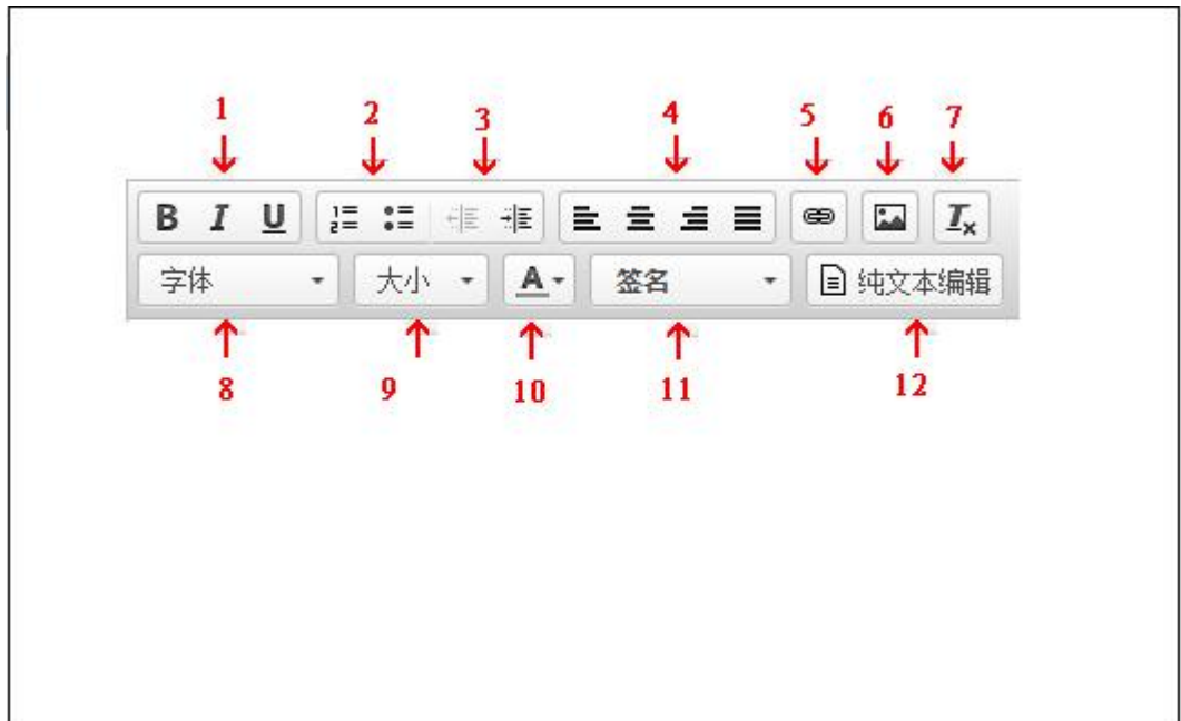
图 4-6 超文本编辑
