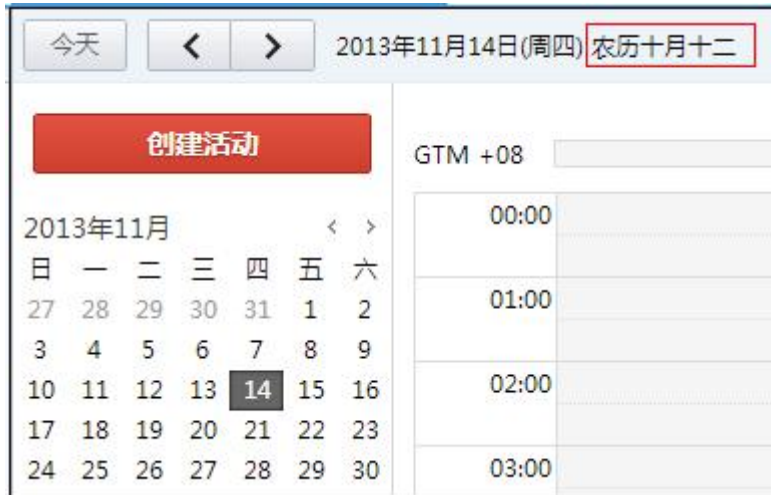
图 4-64 支持阴历
