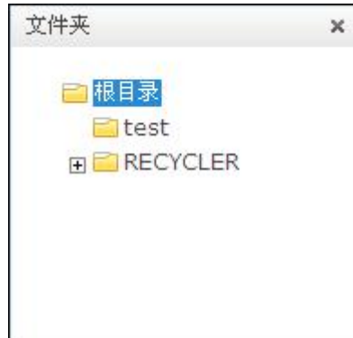
图 4-50 文件夹
