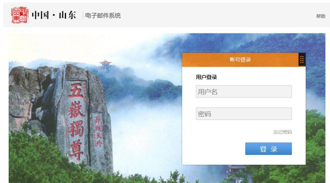
图 2-1 用户登录
