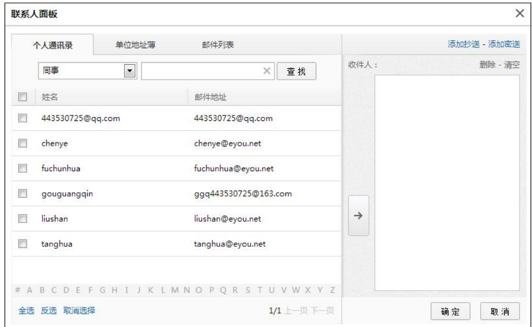
图 4-4 收件人
