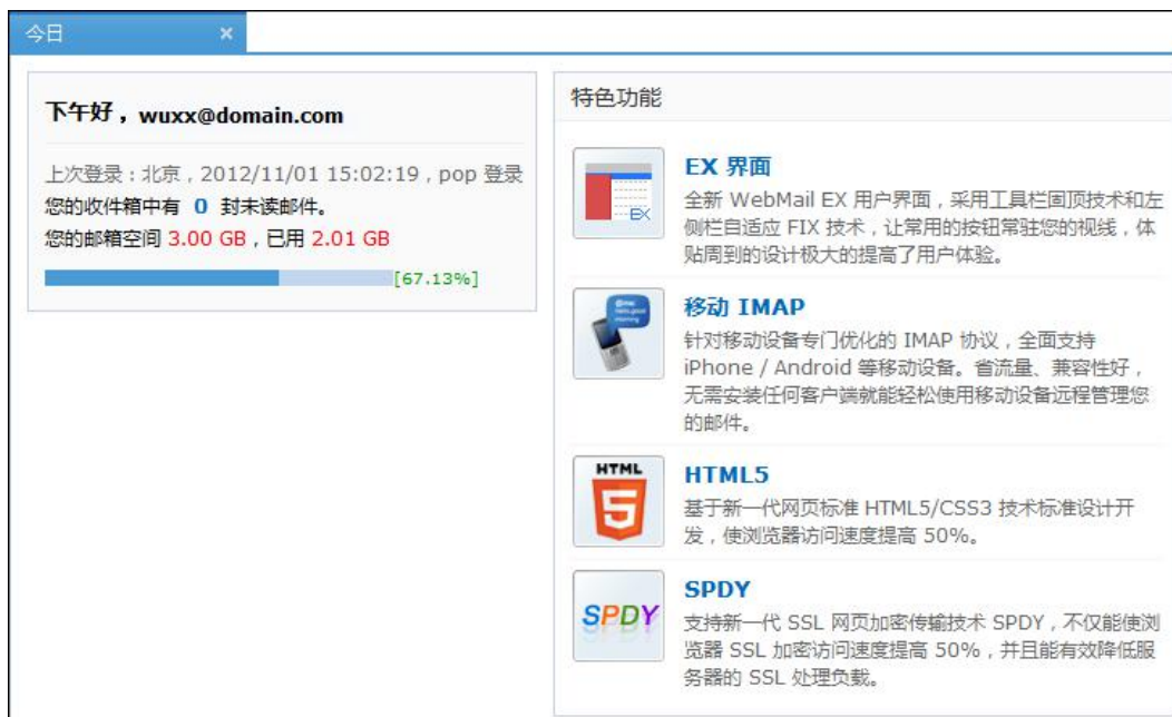
图 3-23 今日
