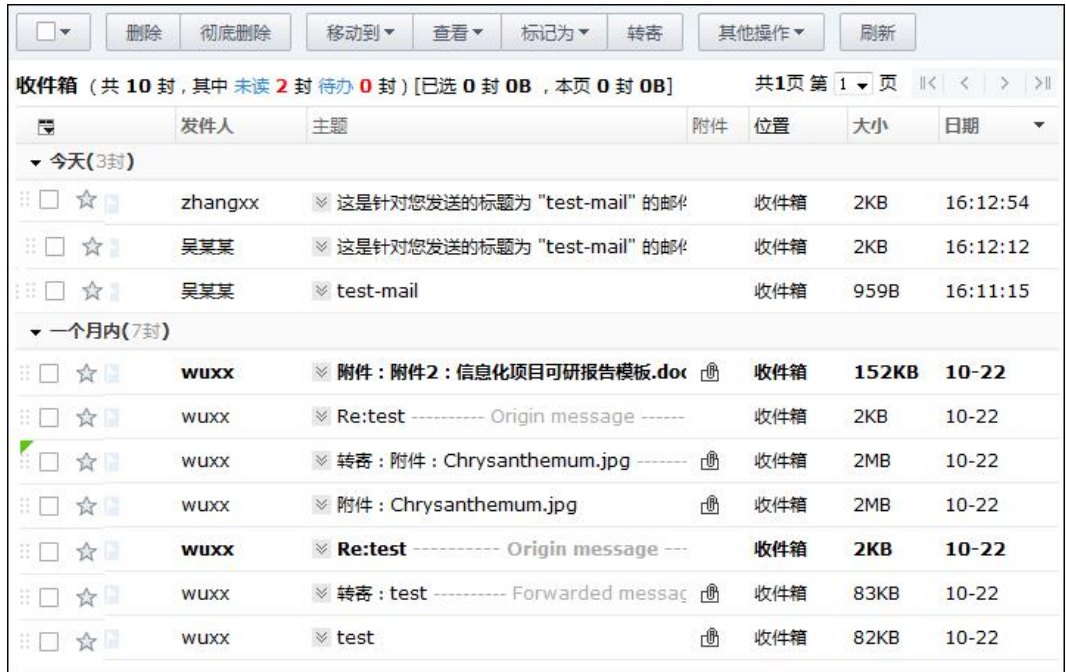
图 4-14 收件箱
