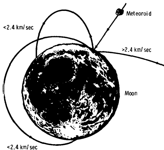
FIGURE 16-1.—Lunar ejecta.
