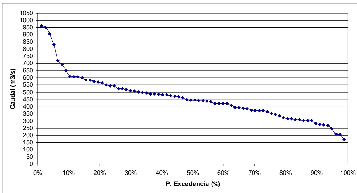
FIGURA 6.3-6 CURVA DE DURACIÓN ESTACIÓN FLUVIOMÉTRICA RÍO FUTALEUFÚ ANTES JUNTA RÍO MALITO
