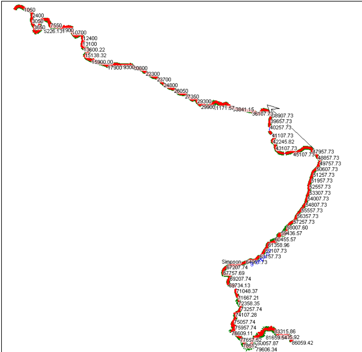
FIGURA 8.6-1 ESQUEMA EN PLANTA DEL MODELO HEC RAS
