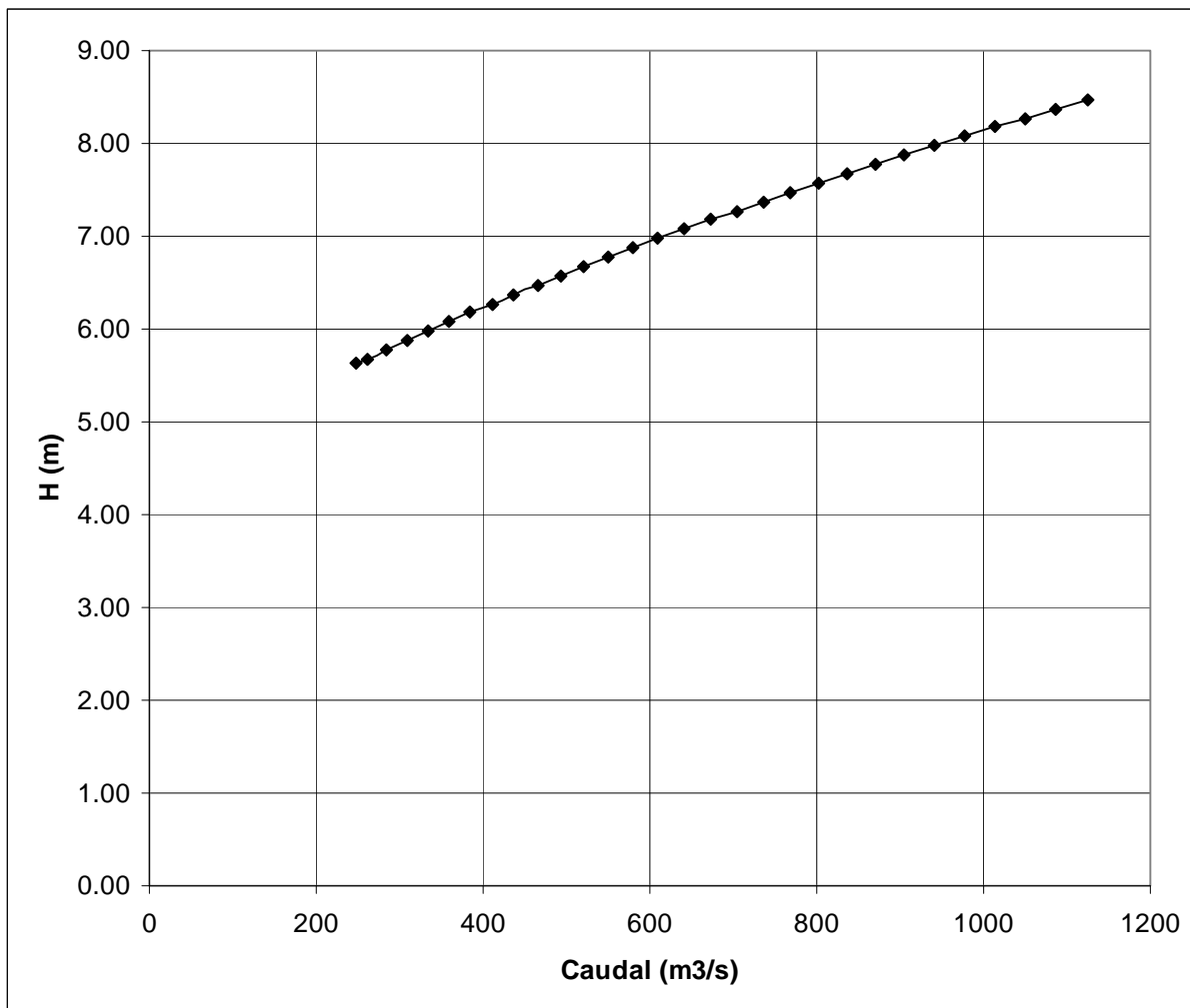
FIGURA 8.5-3 CURVA DE DESCARGA ESTACIÓN FLUVIOMÉTRICA RÍO BAKER EN DESAGÜE LAGO BERTRAND
