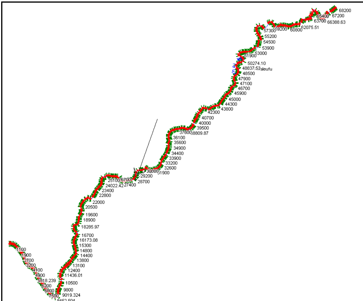
FIGURA 8.4-1 ESQUEMA EN PLANTA DEL MODELO HEC RAS
