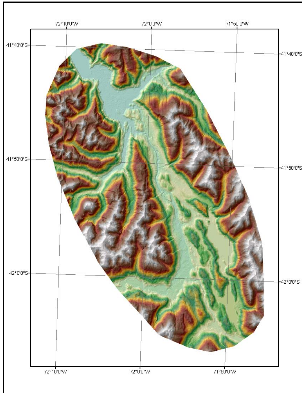
FIGURA 7-6 DEM GENERADO PARA TRAMO DE RÍO PUELO
