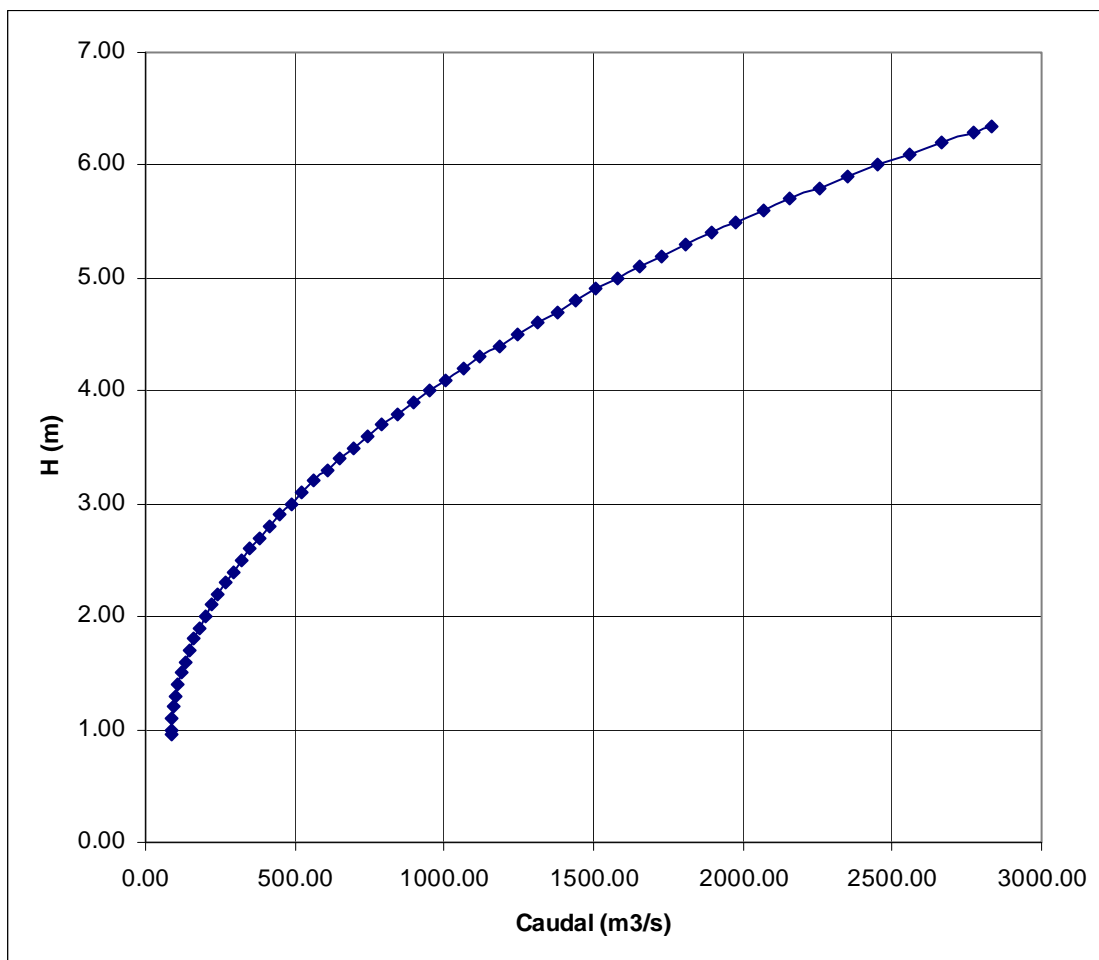
FIGURA 8.7-3 CURVA DE DESCARGA ESTACIÓN FLUVIOMÉTRICA RÍO SERRANO EN DESEMBOCADURA
