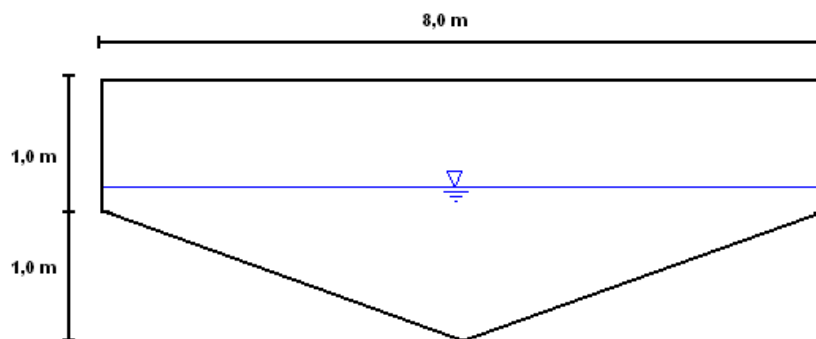
FIGURA 8.2-5 ESQUEMA PERFIL TRANSVERSAL ESTACIÓN FLUVIOMÉTRICA
