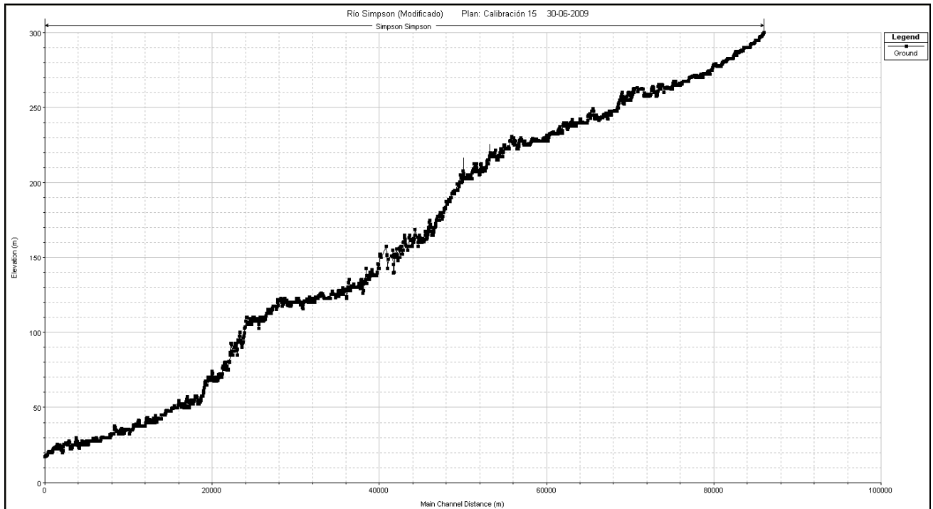
FIGURA 8.6-2 PERFIL LONGITUDINAL MODELO HEC-RAS
