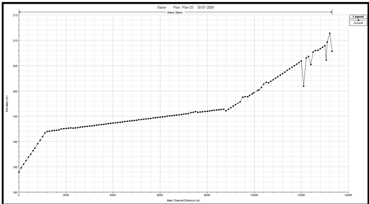
FIGURA 8.5-2 PERFIL LONGITUDINAL MODELO HEC-RAS
