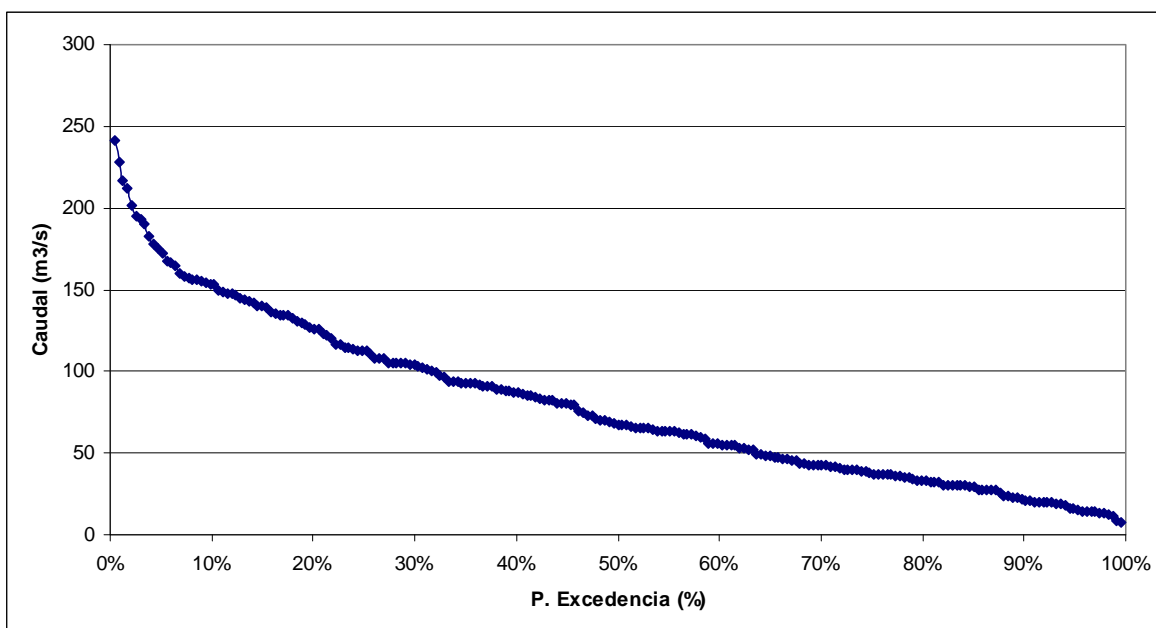
FIGURA 6.4-10 CURVA DE DURACIÓN EN PUNTO DE CONTROL 3, SECTOR ANTES JUNTA RÍO MAÑIGUALES, TRAMO FINAL
