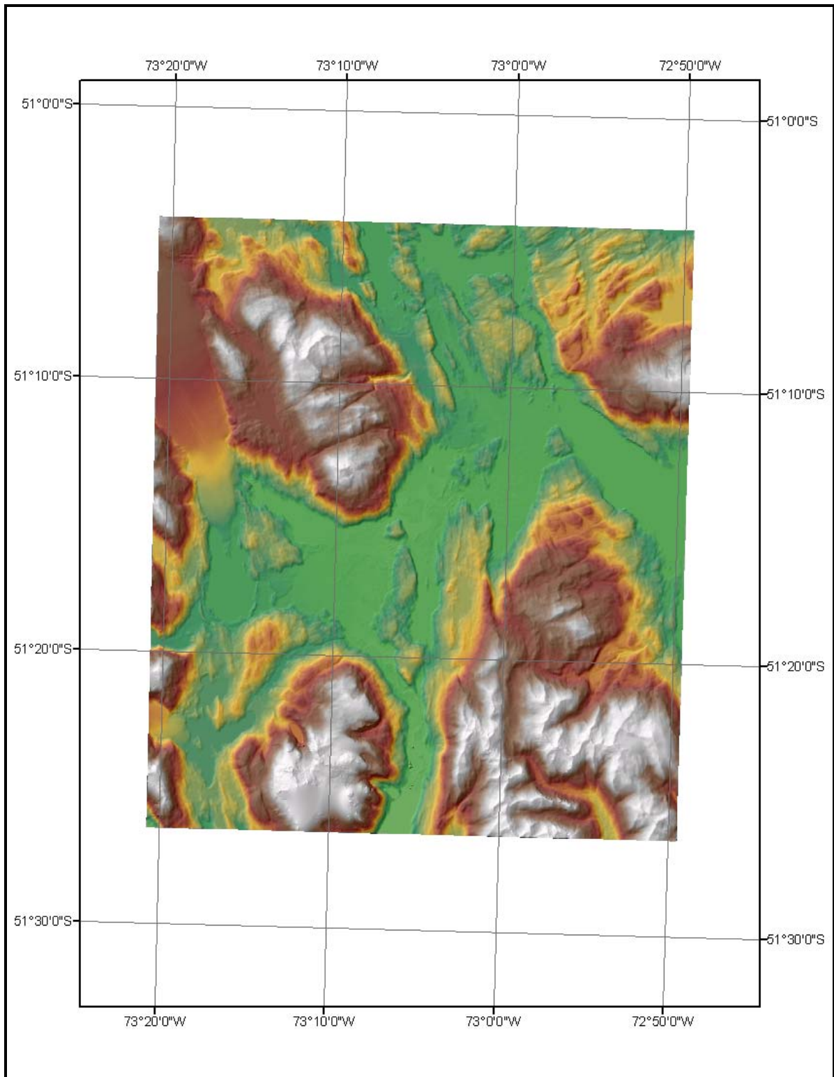
FIGURA 7-10 DEM GENERADO PARA TRAMO DE RÍO SERRANO
