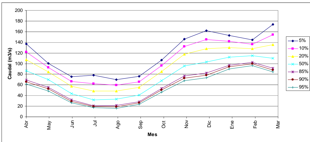
FIGURA 6.6-1 CURVA DE VARIACIÓN ESTACIONAL ESTACIÓN FLUVIOMÉTRICA RÍO SERRANO EN DESAGÜE LAGO TORO
