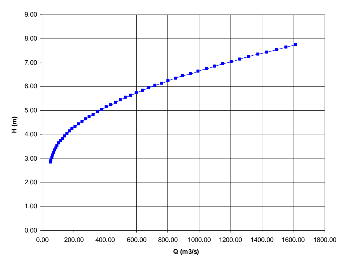
FIGURA 8.3-2 CURVA DE DESCARGA ESTACIÓN FLUVIOMÉTRICA RÍO PUELO ANTES JUNTA MANSO
