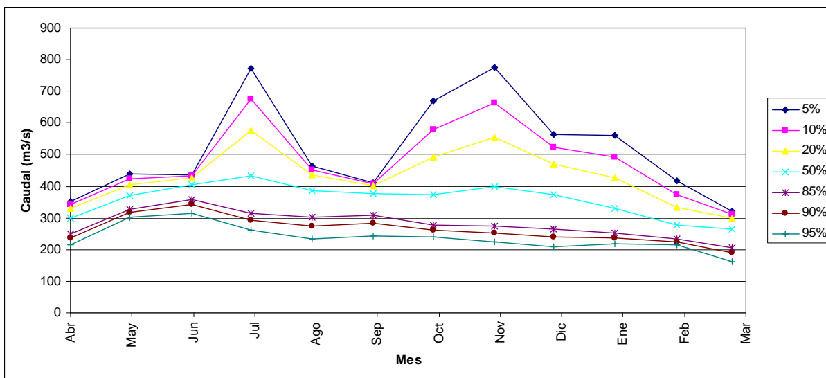
FIGURA 6.3-3 CURVA DE VARIACIÓN ESTACIONAL ESTACIÓN FLUVIOMÉTRICA RÍO FUTALEUFÚ EN LA FRONTERA
