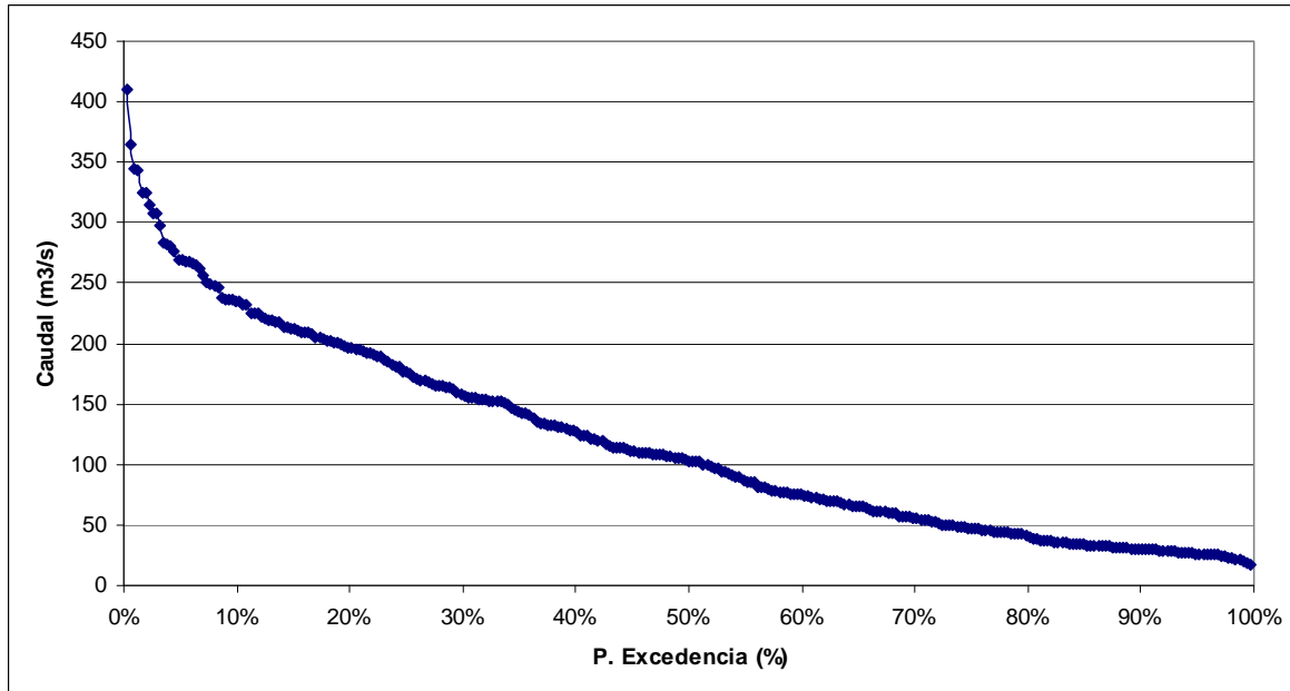
FIGURA 6.6-4 CURVA DE DURACIÓN ESTACIÓN FLUVIOMÉTRICA RÍO GREY ANTES JUNTA RÍO SERRANO.
