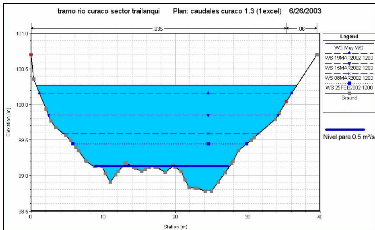
FIGURA 3-3 PERFIL TRANSVERSAL RÍO CURACO
