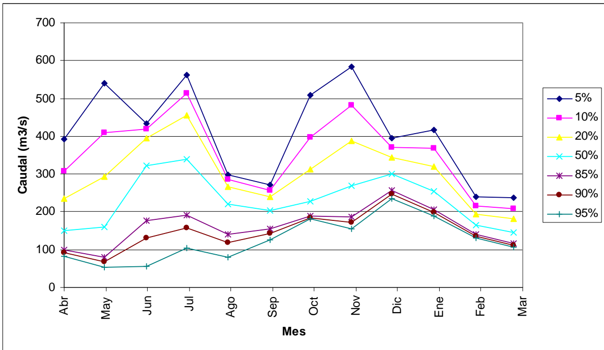
FIGURA 6.2-7 CURVA DE VARIACIÓN ESTACIONAL EN PUNTO DE CONTROL 1, SECTOR FRONTERA, TRAMO INICIAL
