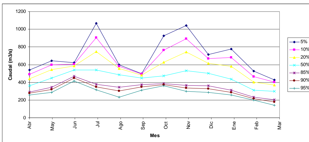
FIGURA 6.3-5 CURVA DE VARIACIÓN ESTACIONAL ESTACIÓN FLUVIOMÉTRICA RÍO FUTALEUFÚ ANTES JUNTA RÍO MALITO
