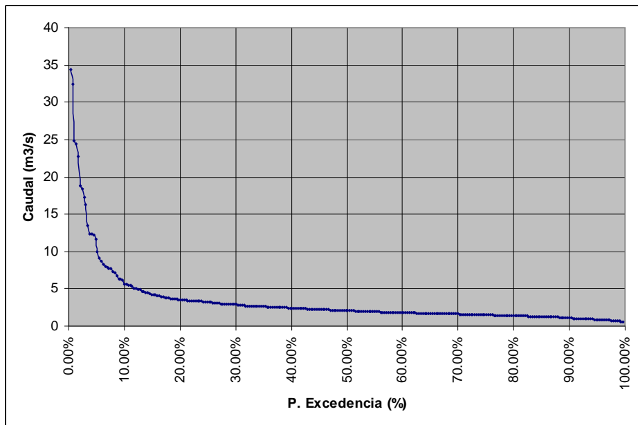
FIGURA 6.1-6 CURVA DE DURACIÓN EN PUNTO DE CONTROL 1, SECTOR MONTEGRANDE, TRAMO FINAL
