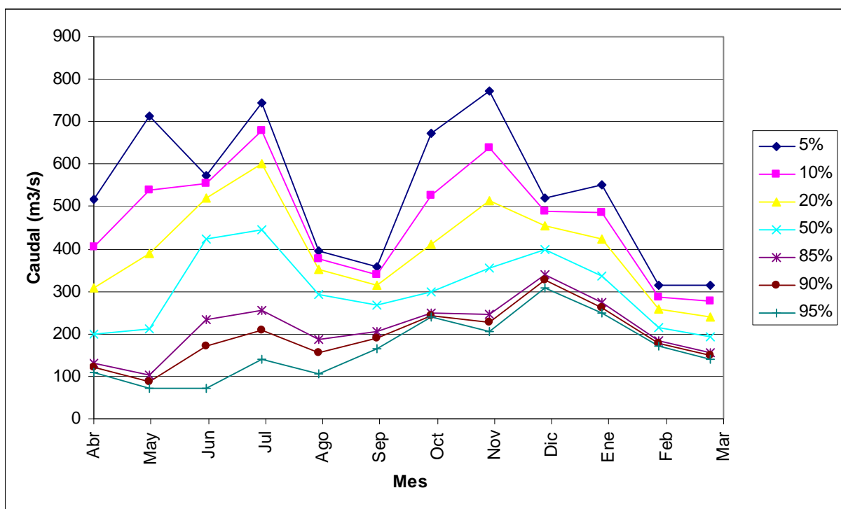
FIGURA 6.2-9 CURVA DE VARIACIÓN ESTACIONAL EN PUNTO DE CONTROL 2, TRAMO MEDIO
