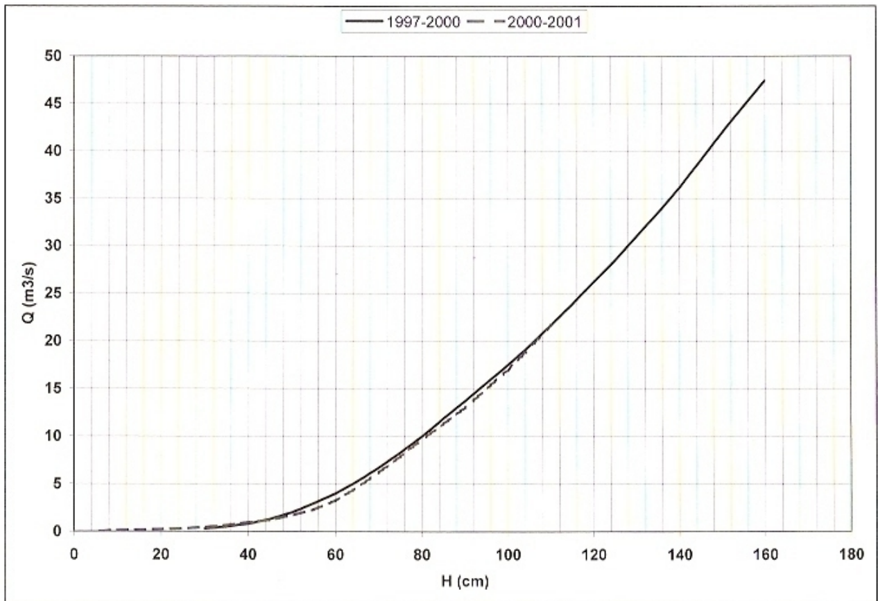
FIGURA 8.2-3 CURVA DE DESCARGA ESTACIÓN FLUVIOMÉTRICA RÍO COCHIGUAZ EN EL PEÑÓN
