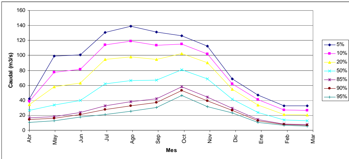
FIGURA 6.4-2 CURVA DE DURACIÓN ESTACIÓN FLUVIOMÉTRICA RÍO SIMPSON BAJO JUNTA RÍO COYHAIQUE
