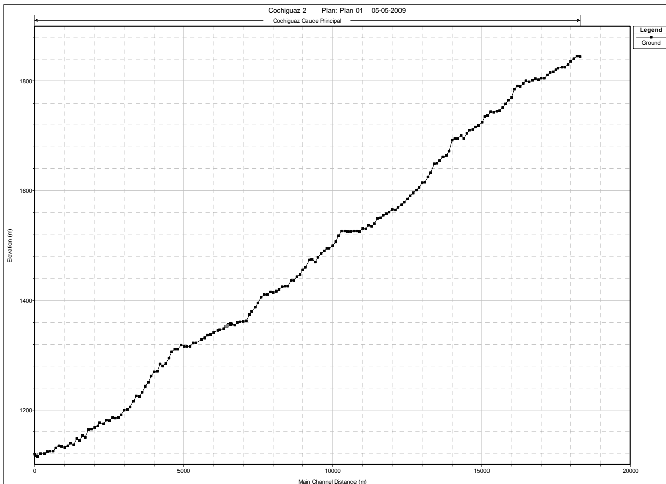
FIGURA 8.2-2 PERFIL LONGITUDINAL MODELO HEC-RAS
