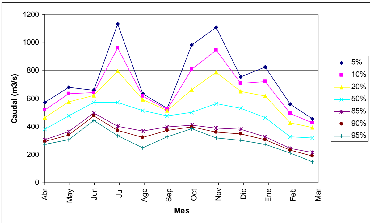
FIGURA 6.3-14 CURVA DE DURACIÓN EN PUNTO DE CONTROL 3, SECTOR LAGO YELCHO, TRAMO FINAL
