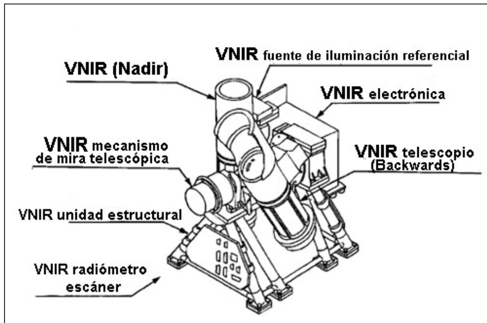
FIGURA 7-3 SISTEMA TELESCÓPICO DEL SENSOR ASTER
