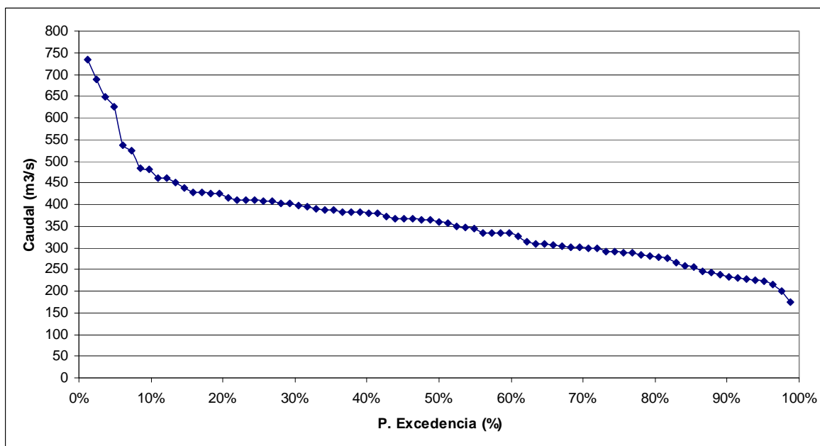
FIGURA 6.3-4 CURVA DE DURACIÓN ESTACIÓN FLUVIOMÉTRICA RÍO FUTALEUFÚ EN LA FRONTERA
