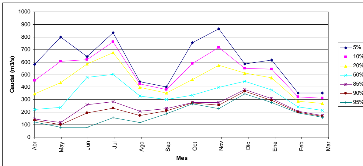
FIGURA 6.2-3 CURVA DE VARIACIÓN ESTACIONAL ESTACIÓN FLUVIOMÉTRICA RÍO PUELO ANTES JUNTA CON RÍO MANSO
