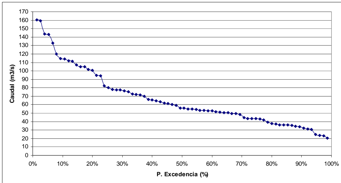
FIGURA 6.3-2 CURVA DE DURACIÓN ESTACIÓN FLUVIOMÉTRICA RÍO ESPOLÓN EN DESAGÜE LAGO ESPOLÓN
