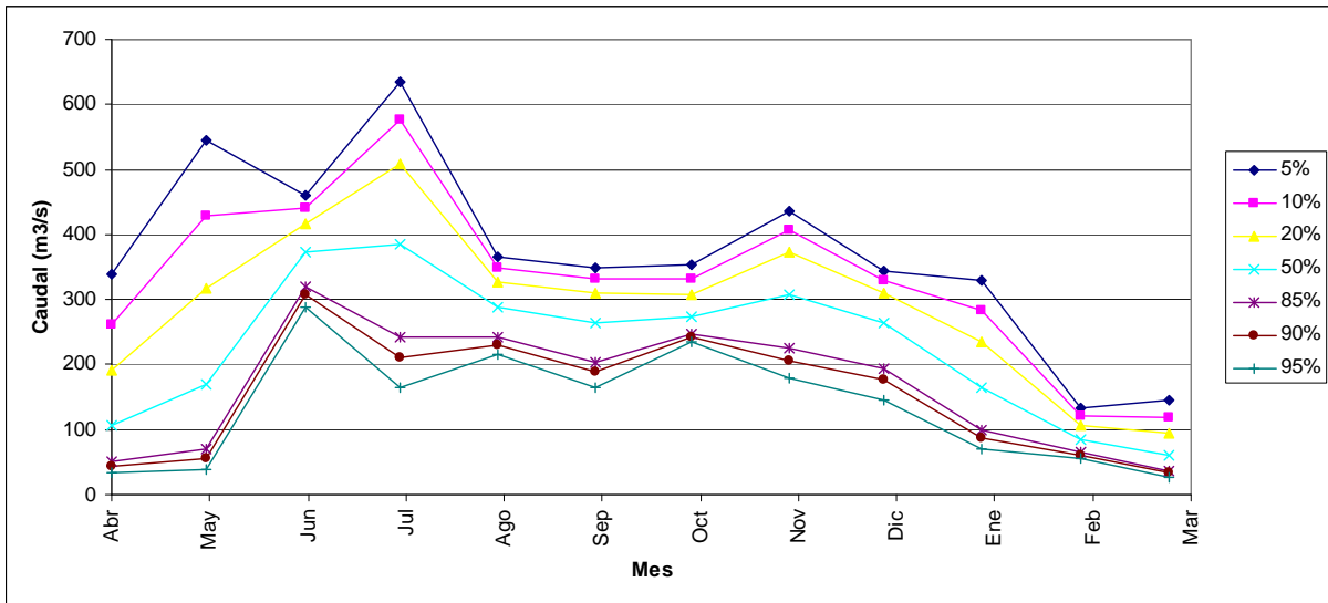
FIGURA 6.2-2 CURVA DE DURACIÓN ESTACIÓN FLUVIOMÉTRICA RÍO MANSO ANTES JUNTA CON RÍO PUELO
