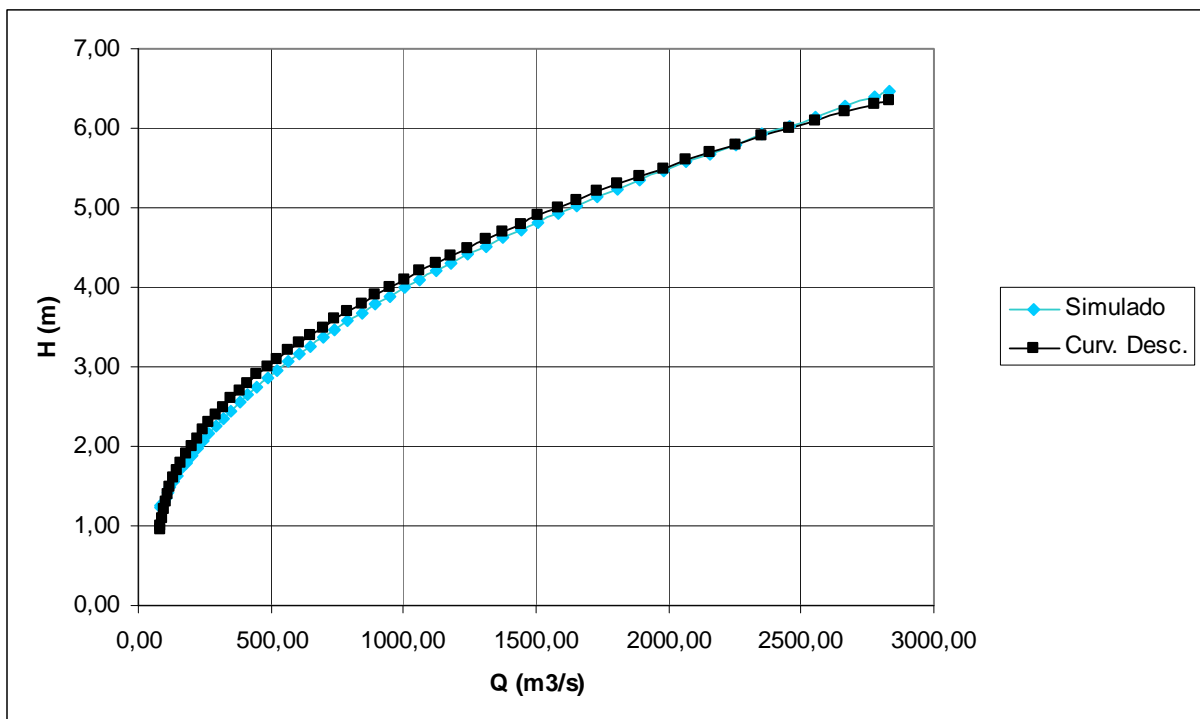
FIGURA 8.7-5 RESULTADOS CALIBRACIÓN ESTACIÓN FLUVIOMÉTRICA
