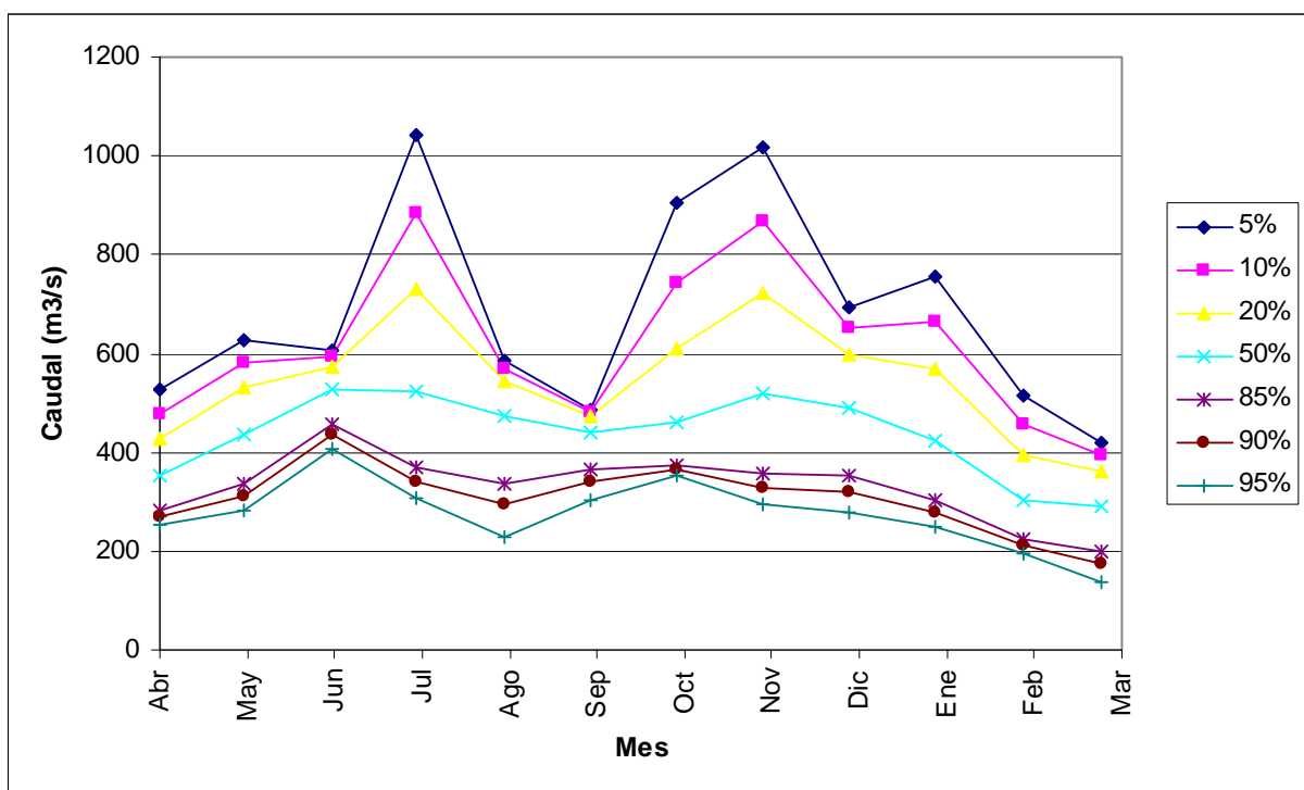
FIGURA 6.3-11 CURVA DE VARIACIÓN ESTACIONAL EN PUNTO DE CONTROL 2, TRAMO MEDIO
