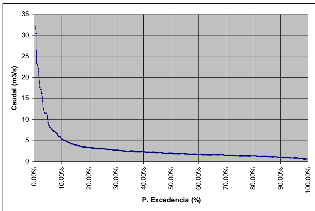
FIGURA 6.1-2 CURVA DE DURACIÓN ESTACIÓN FLUVIOMÉTRICA COCHIGUAZ EN EL PEÑÓN
