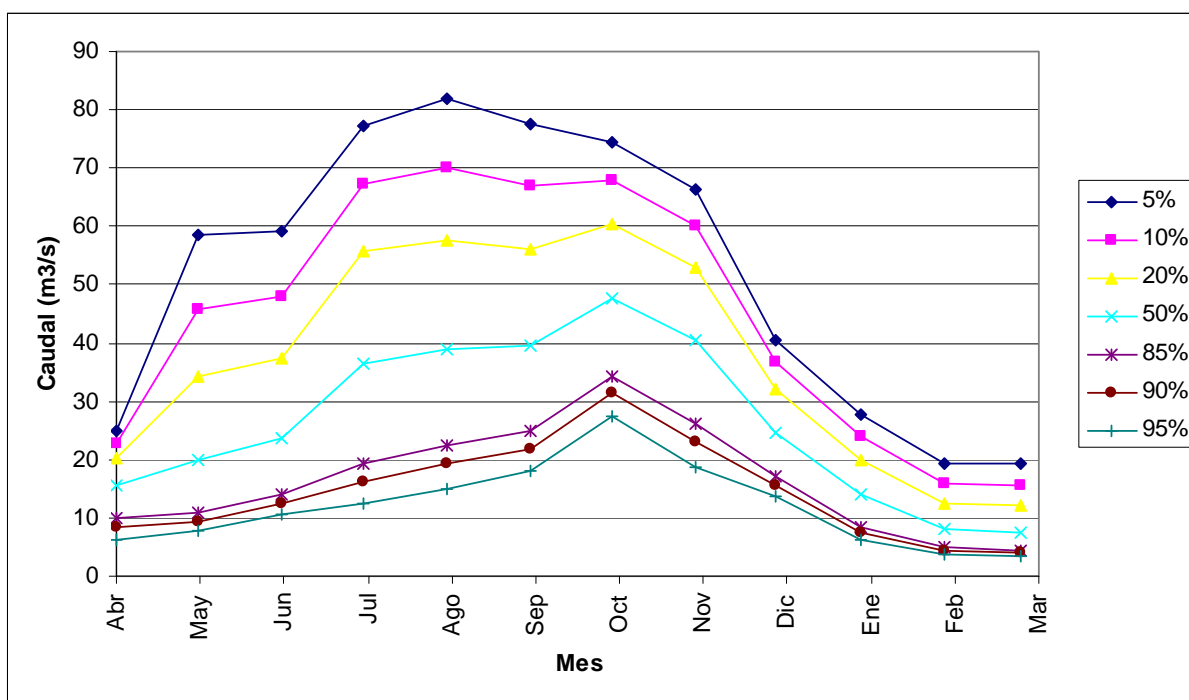
FIGURA 6.4-5 CURVA DE VARIACIÓN ESTACIONAL EN PUNTO DE CONTROL 1, SECTOR ANTES JUNTA RÍO POLUX, TRAMO INICIAL
