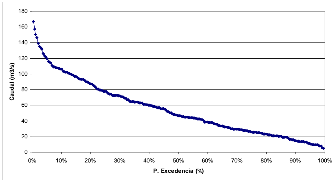
FIGURA 6.4-8 CURVA DE DURACIÓN EN PUNTO DE CONTROL 2, TRAMO MEDIO
