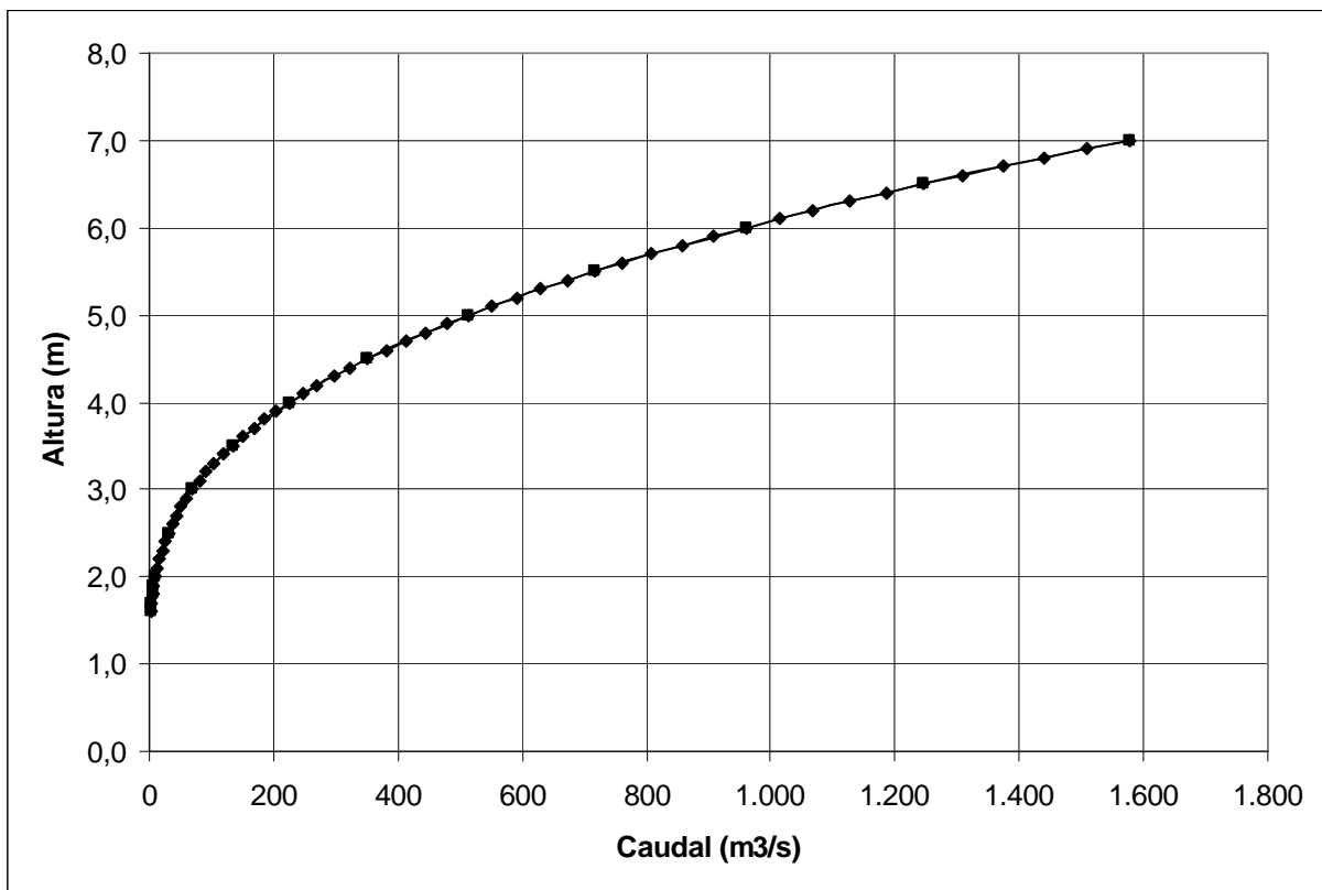
FIGURA 8.6-3 CURVA DE DESCARGA ESTACIÓN FLUVIOMÉTRICA RÍO SIMPSON BAJO JUNTA COYHAIQUE
