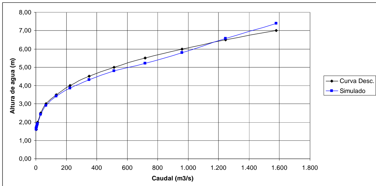
FIGURA 8.6-6 RESULTADOS CALIBRACIÓN ESTACIÓN FLUVIOMÉTRICA
