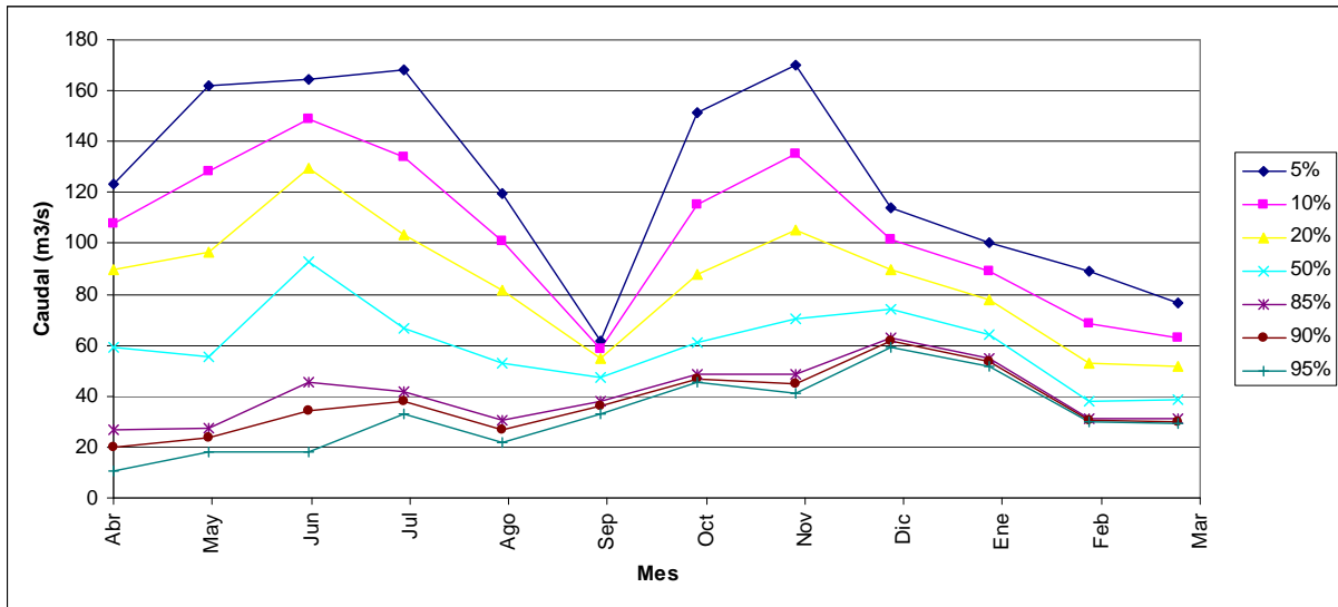
FIGURA 6.3-2 CURVA DE DURACIÓN ESTACIÓN FLUVIOMÉTRICA RÍO ESPOLÓN EN DESAGÜE LAGO ESPOLÓN
