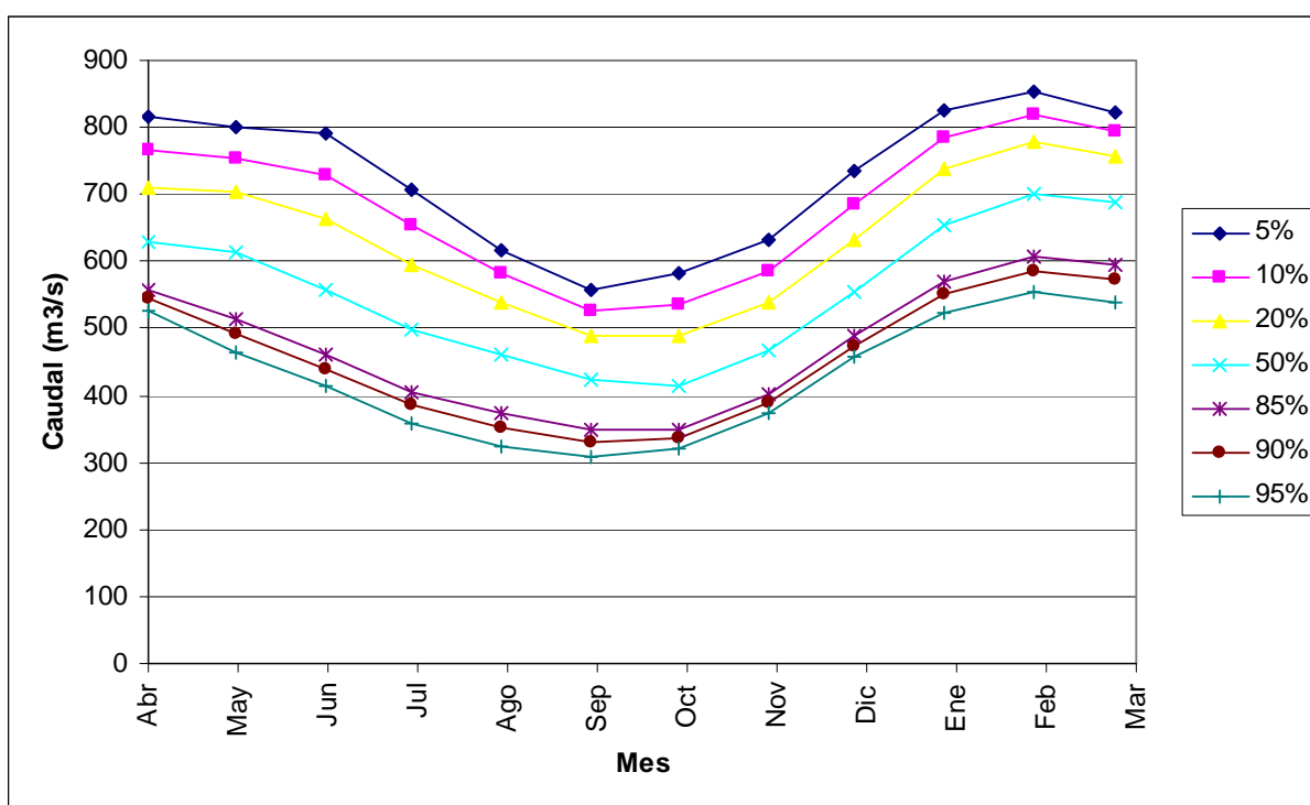
FIGURA 6.5-9 CURVA DE VARIACIÓN ESTACIONAL EN PUNTO DE CONTROL 3, SECTOR DESAGÜE LAGO BERTRAND, TRAMO INICIAL
