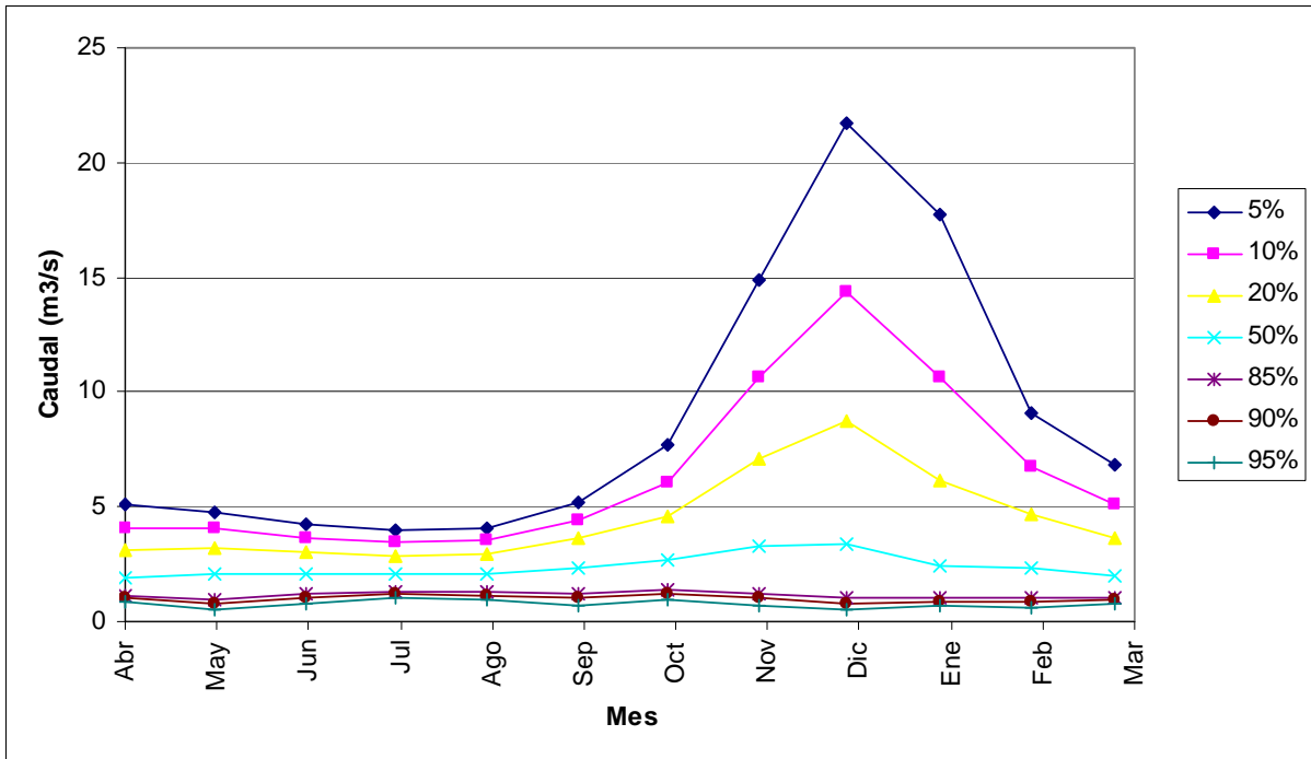
FIGURA 6.1-6 CURVA DE DURACIÓN EN PUNTO DE CONTROL 1, SECTOR MONTEGRANDE, TRAMO FINAL
