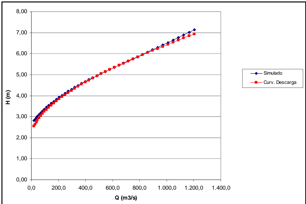
FIGURA 8.4-4 RESULTADOS CALIBRACIÓN ESTACIÓN FLUVIOMÉTRICA FUTALEUFÚ EN LA FRONTERA
