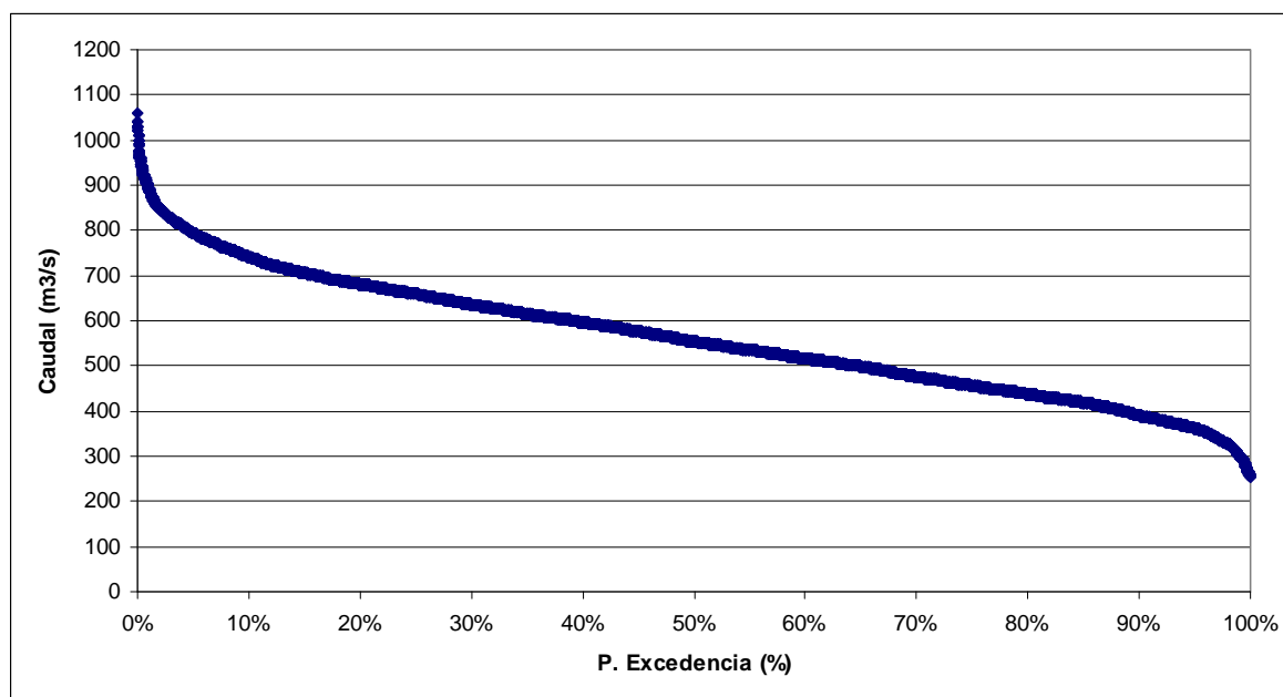
FIGURA 6.5-2 CURVA DE DURACIÓN ESTACIÓN FLUVIOMÉTRICA RÍO BAKER EN DESAGÜE LAGO BERTRAND (ENDESA)
