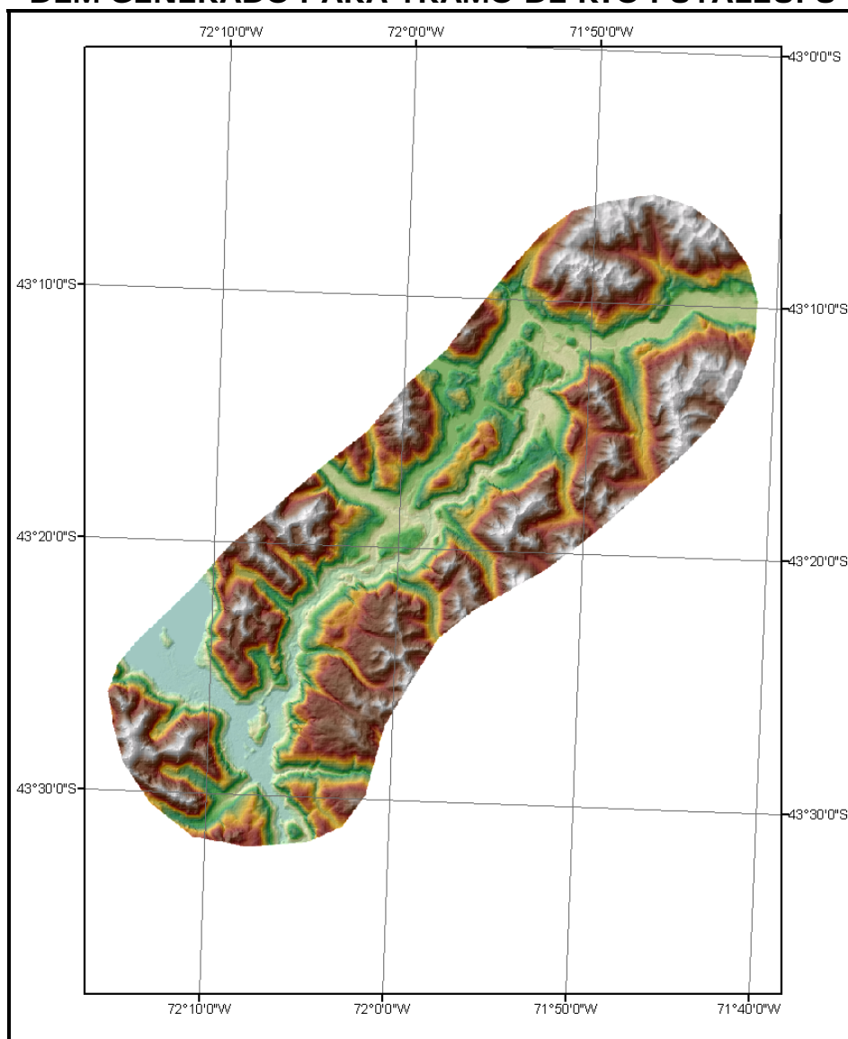
FIGURA 7-7 DEM GENERADO PARA TRAMO DE RÍO FUTALEUFÚ
