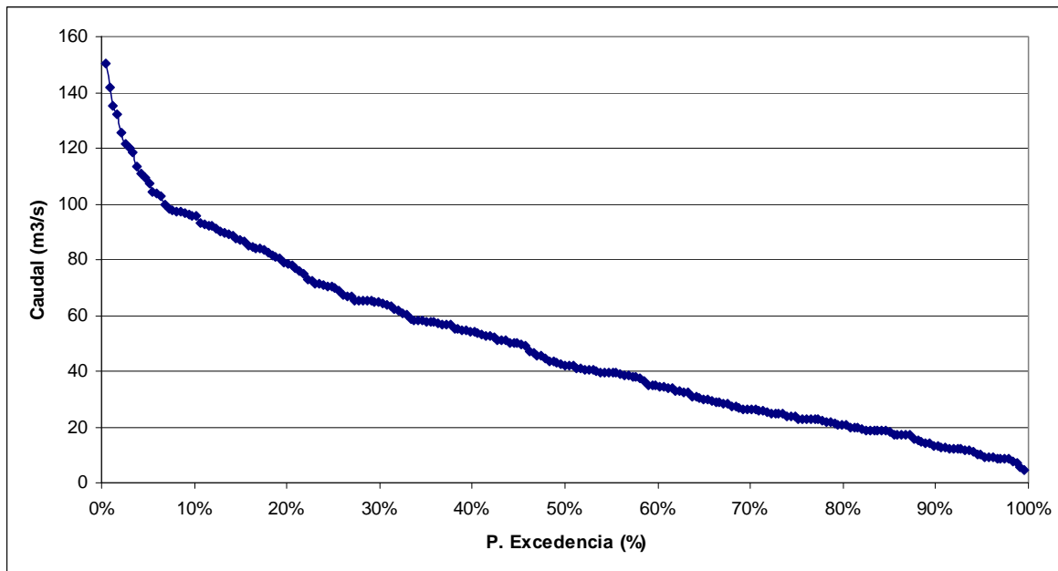
FIGURA 6.4-2 CURVA DE DURACIÓN ESTACIÓN FLUVIOMÉTRICA RÍO SIMPSON BAJO JUNTA RÍO COYHAIQUE
