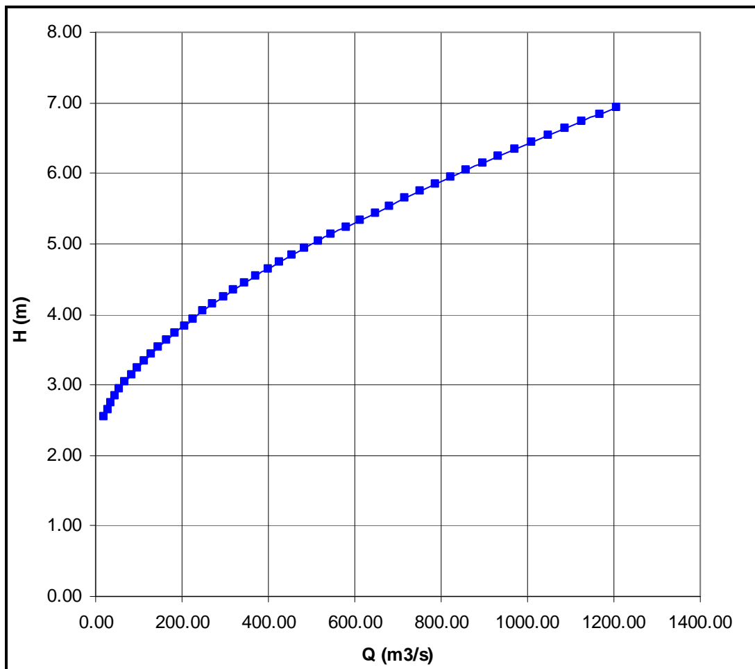
FIGURA 8.4-2 CURVA DE DESCARGA ESTACIÓN FLUVIOMÉTRICA RÍO FUTALEUFÚ EN LA FRONTERA
