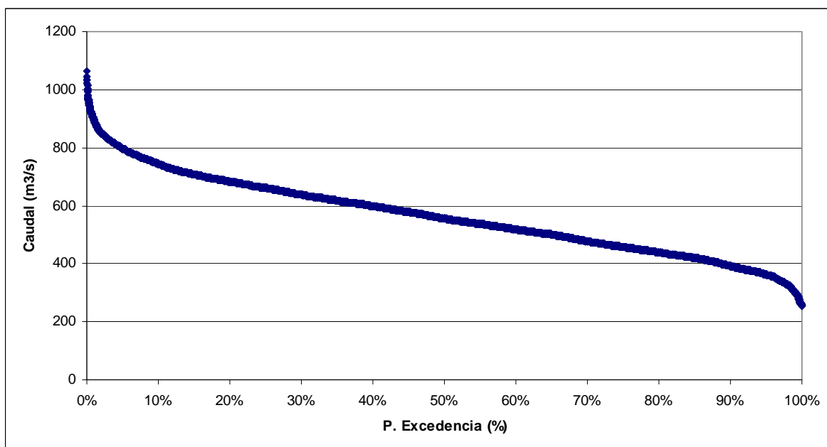
FIGURA 6.5-8 CURVA DE DURACIÓN EN PUNTO DE CONTROL 2, TRAMO MEDIO
