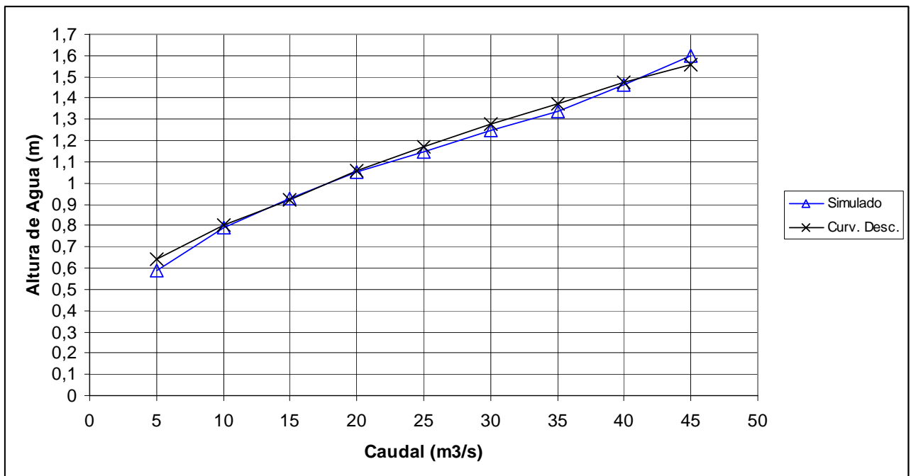
FIGURA 8.2-6 RESULTADOS CALIBRACIÓN ESTACIÓN FLUVIOMÉTRICA
