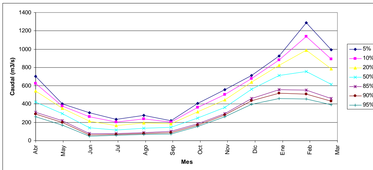
FIGURA 6.6-5 CURVA DE VARIACIÓN ESTACIONAL ESTACIÓN FLUVIOMÉTRICA RÍO SERRANO EN DESEMBOCADURA
