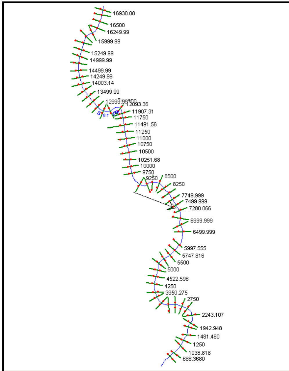
FIGURA 8.7-2 ESQUEMA EN PLANTA DEL MODELO HEC RAS
