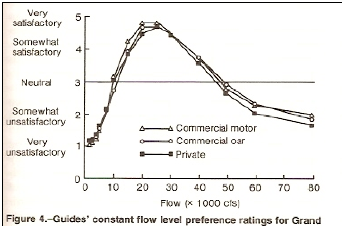
FIGURA 3-18 CURVAS DE CAUDALES ÓPTIMAS EN EL GRAN CAÑÓN PARA EMBARCACIONES DE RÍO
