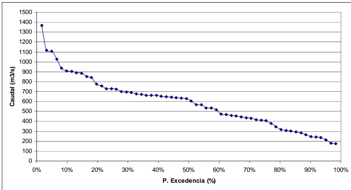
FIGURA 6.2-12 CURVA DE DURACIÓN EN PUNTO DE CONTROL 3, SECTOR LAGO TAGUA-TAGUA, TRAMO FINAL
