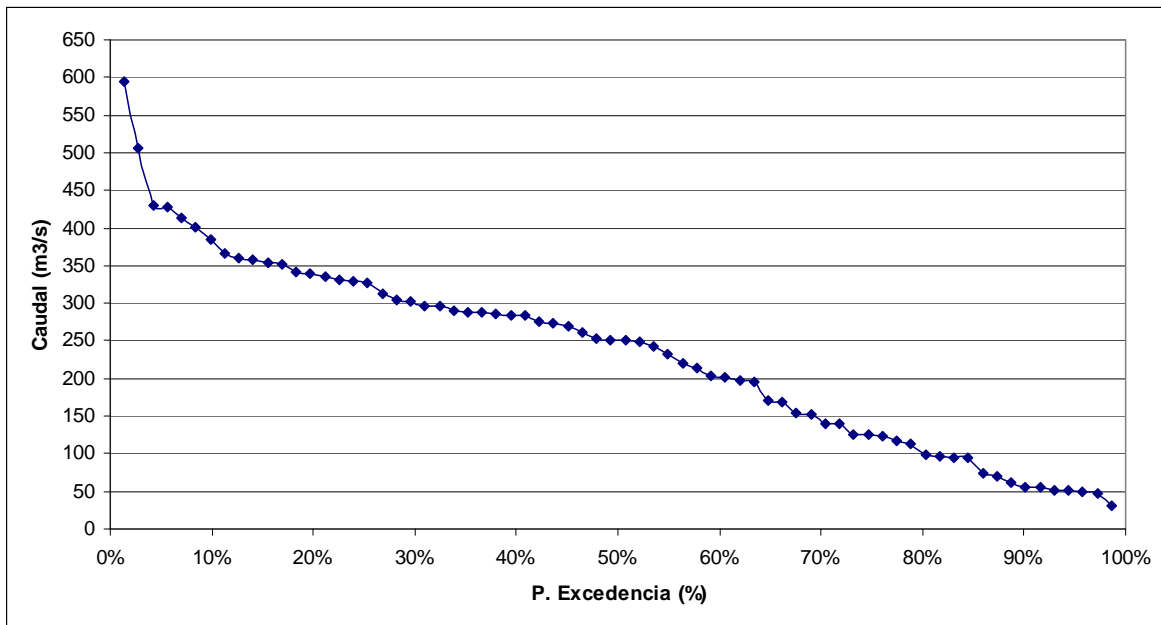
FIGURA 6.2-2 CURVA DE DURACIÓN ESTACIÓN FLUVIOMÉTRICA RÍO MANSO ANTES JUNTA CON RÍO PUELO
