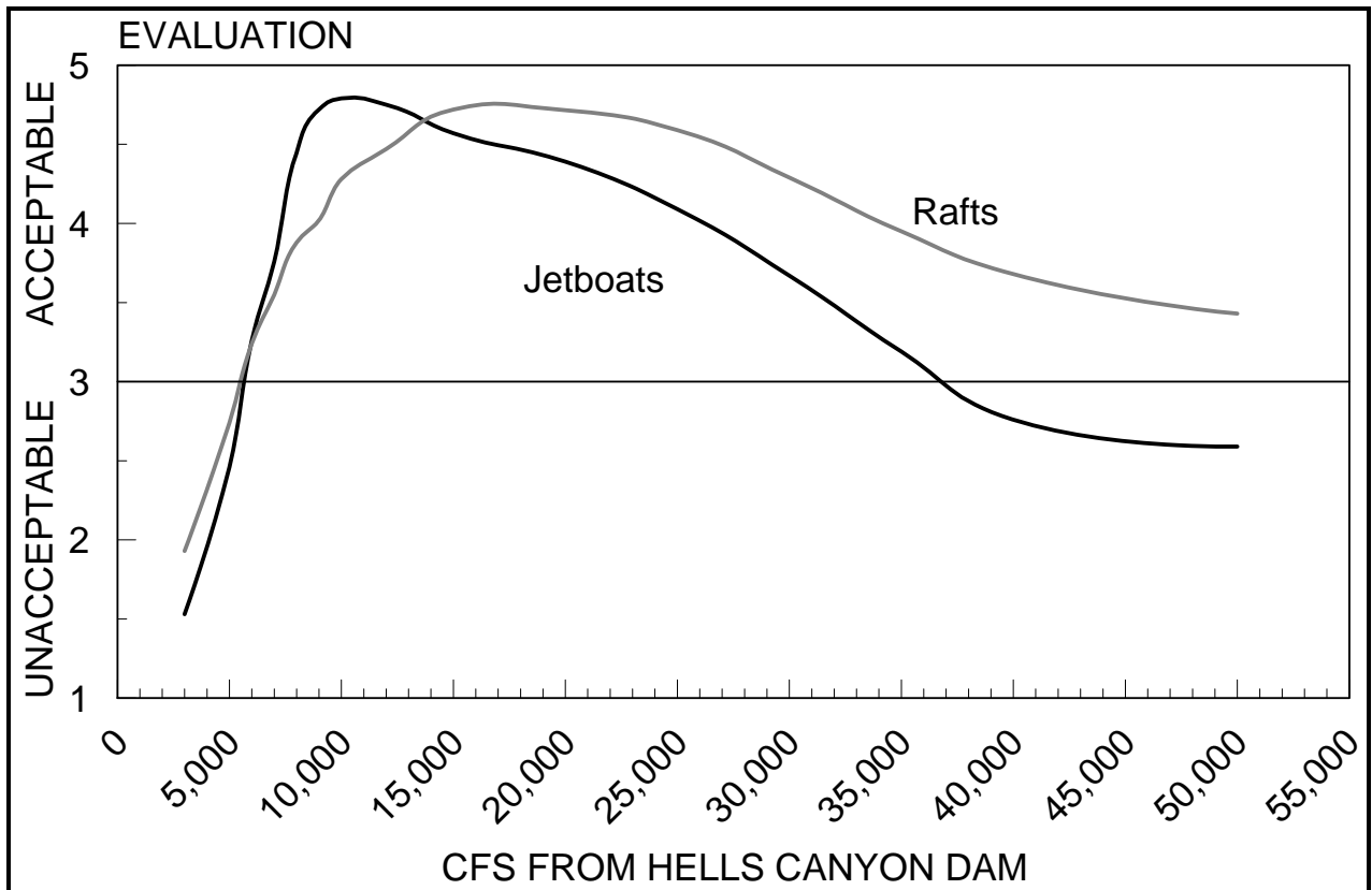
FIGURA 3.15 EVALUACIÓN DE CAUDALES PARA RAFTING Y LANCHAS EN RÍO SERPIENTE
