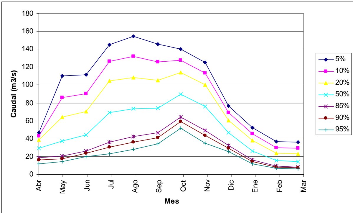
FIGURA 6.4-8 CURVA DE DURACIÓN EN PUNTO DE CONTROL 2, TRAMO MEDIO
