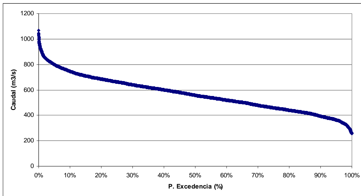
FIGURA 6.5-6 CURVA DE DURACIÓN EN PUNTO DE CONTROL 1, SECTOR CONF. RÍO NEF, TRAMO FINAL
