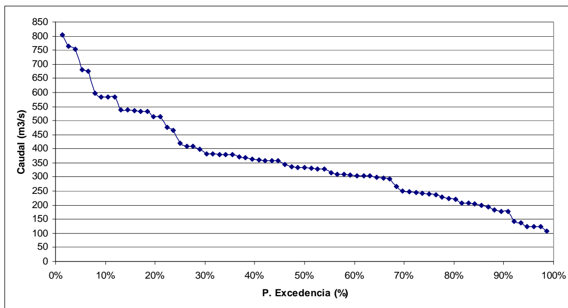
FIGURA 6.2-4 CURVA DE DURACIÓN ESTACIÓN FLUVIOMÉTRICA RÍO PUELO ANTES JUNTA CON RÍO MANSO
