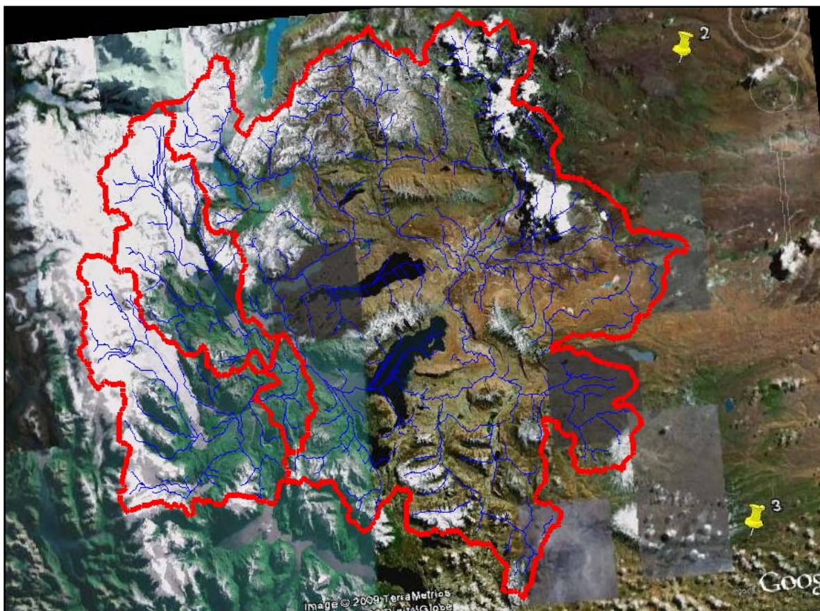
FIGURA 6.6-7 DELIMITACIÓN DE SUBCUENCAS RÍO SERRANO
