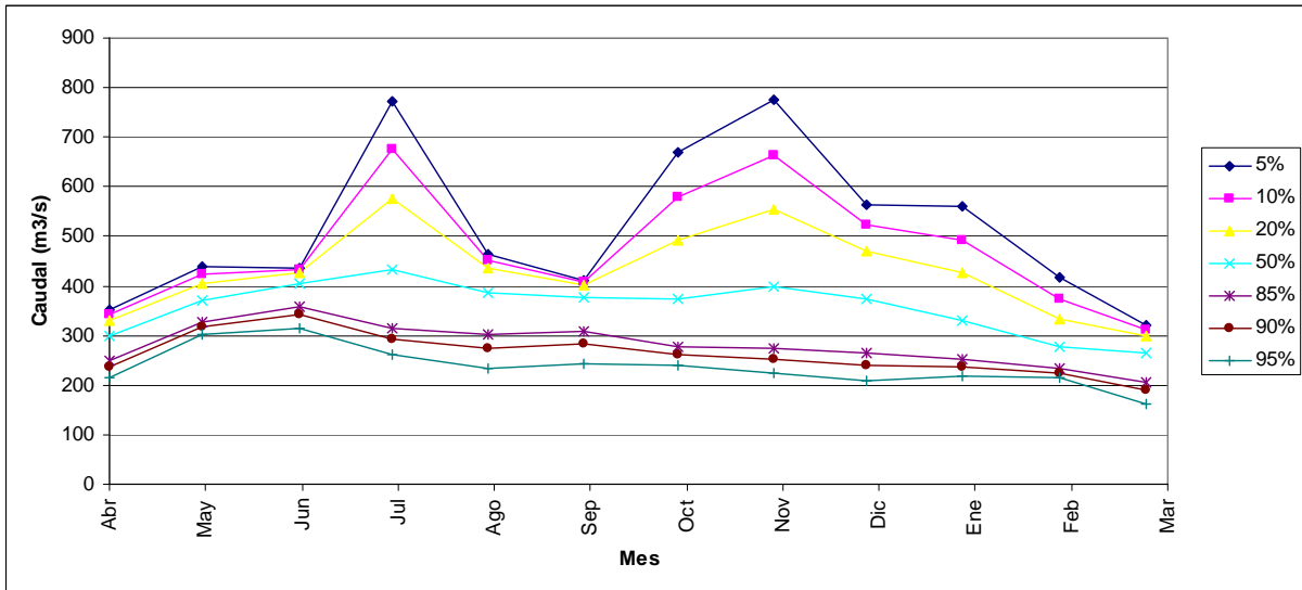
FIGURA 6.3-9 CURVA DE VARIACIÓN ESTACIONAL EN PUNTO DE CONTROL 1, SECTOR FRONTERA, TRAMO INICIAL
