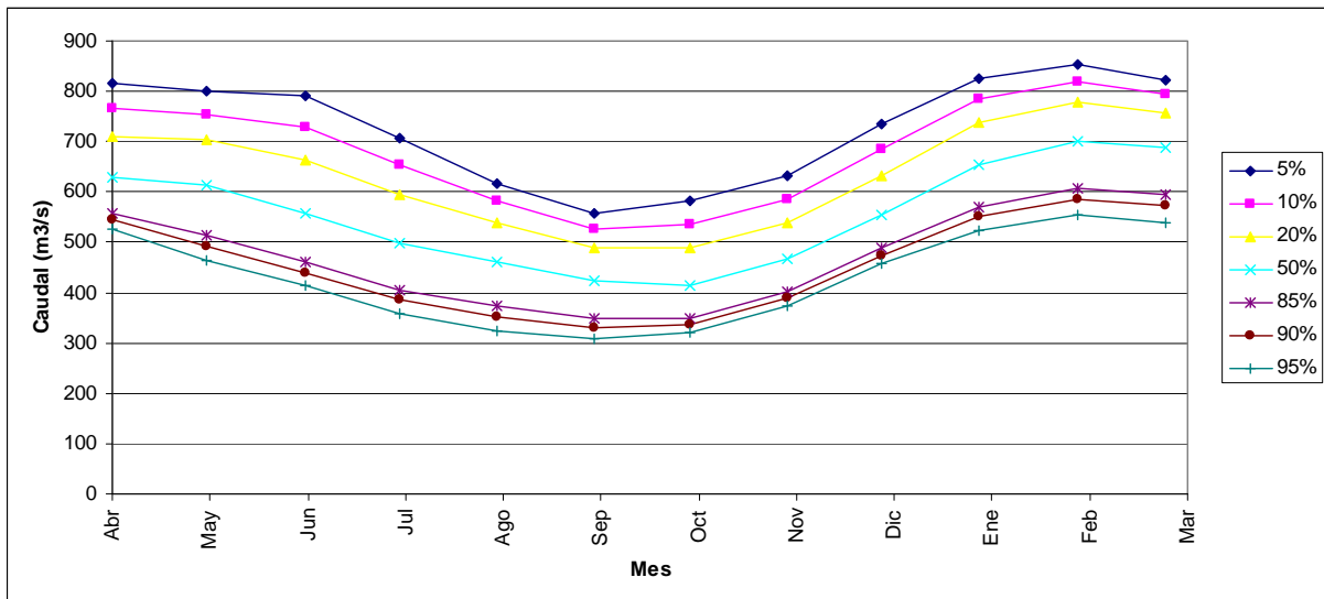
FIGURA 6.5-1 CURVA DE VARIACIÓN ESTACIONAL ESTACIÓN FLUVIOMÉTRICA RÍO BAKER EN DESAGÜE LAGO BERTRAND (ENDESA)
