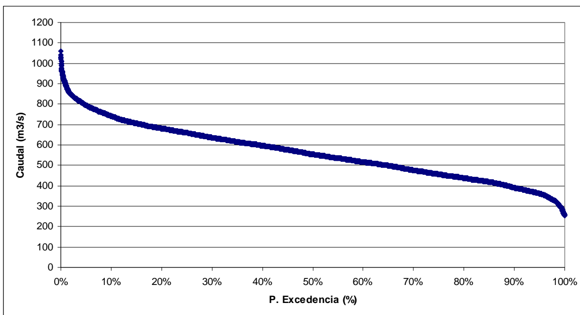
FIGURA 6.5-10 CURVA DE DURACIÓN EN PUNTO DE CONTROL 3, SECTOR DESAGÜE LAGO BERTRAND, TRAMO INICIAL
