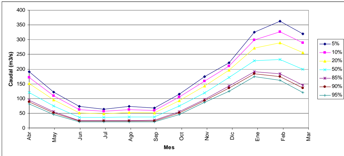
FIGURA 6.6-4 CURVA DE DURACIÓN ESTACIÓN FLUVIOMÉTRICA RÍO GREY ANTES JUNTA RÍO SERRANO.
