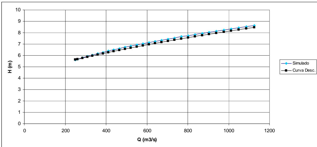
FIGURA 8.5-5 RESULTADOS CALIBRACIÓN ESTACIÓN FLUVIOMÉTRICA
