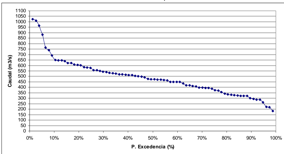
FIGURA 6.3-14 CURVA DE DURACIÓN EN PUNTO DE CONTROL 3, SECTOR LAGO YELCHO, TRAMO FINAL
