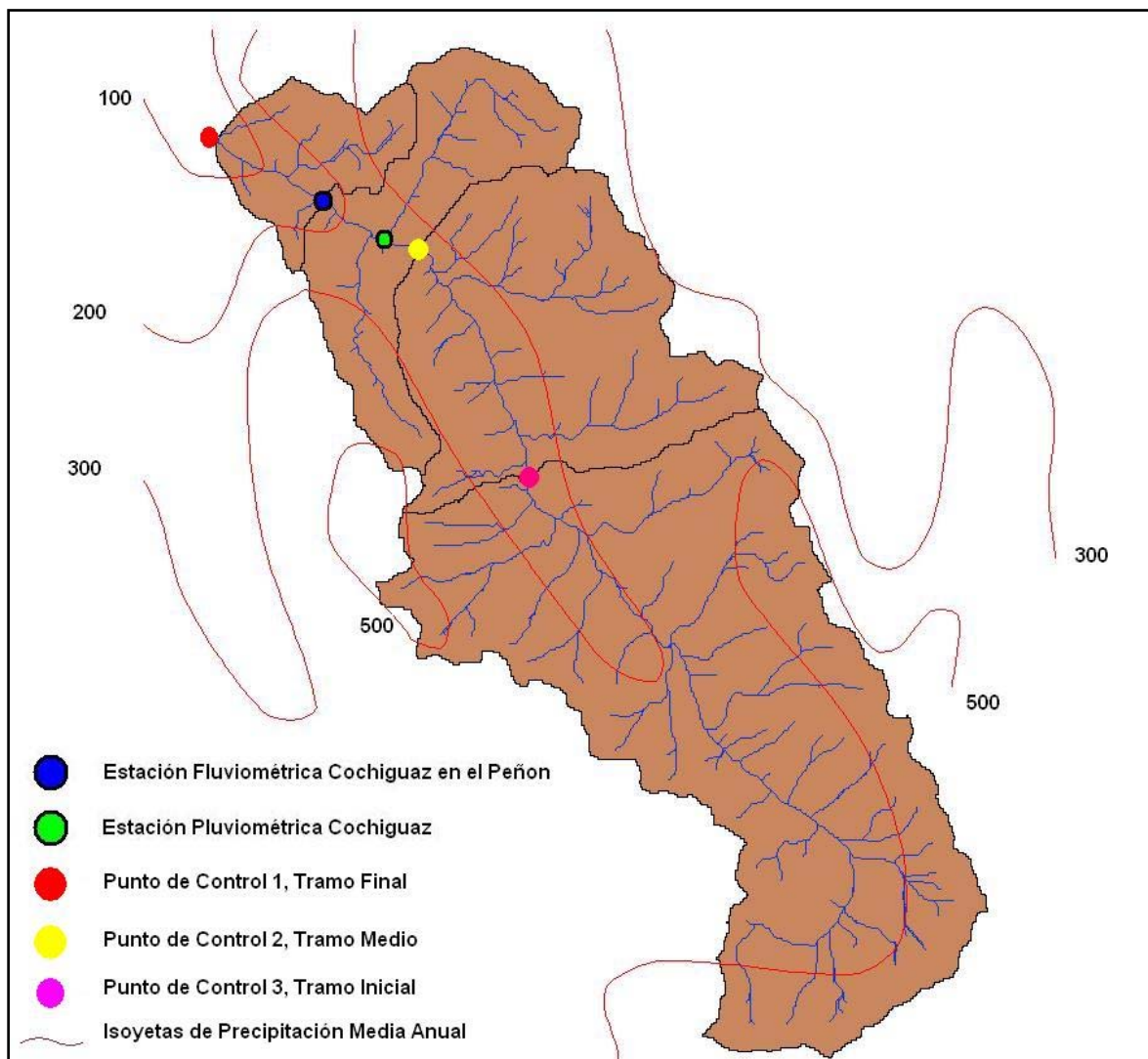
FIGURA 6.1-4 DELIMITACIÓN DE CUENCAS EN PUNTOS DE CONTROL
