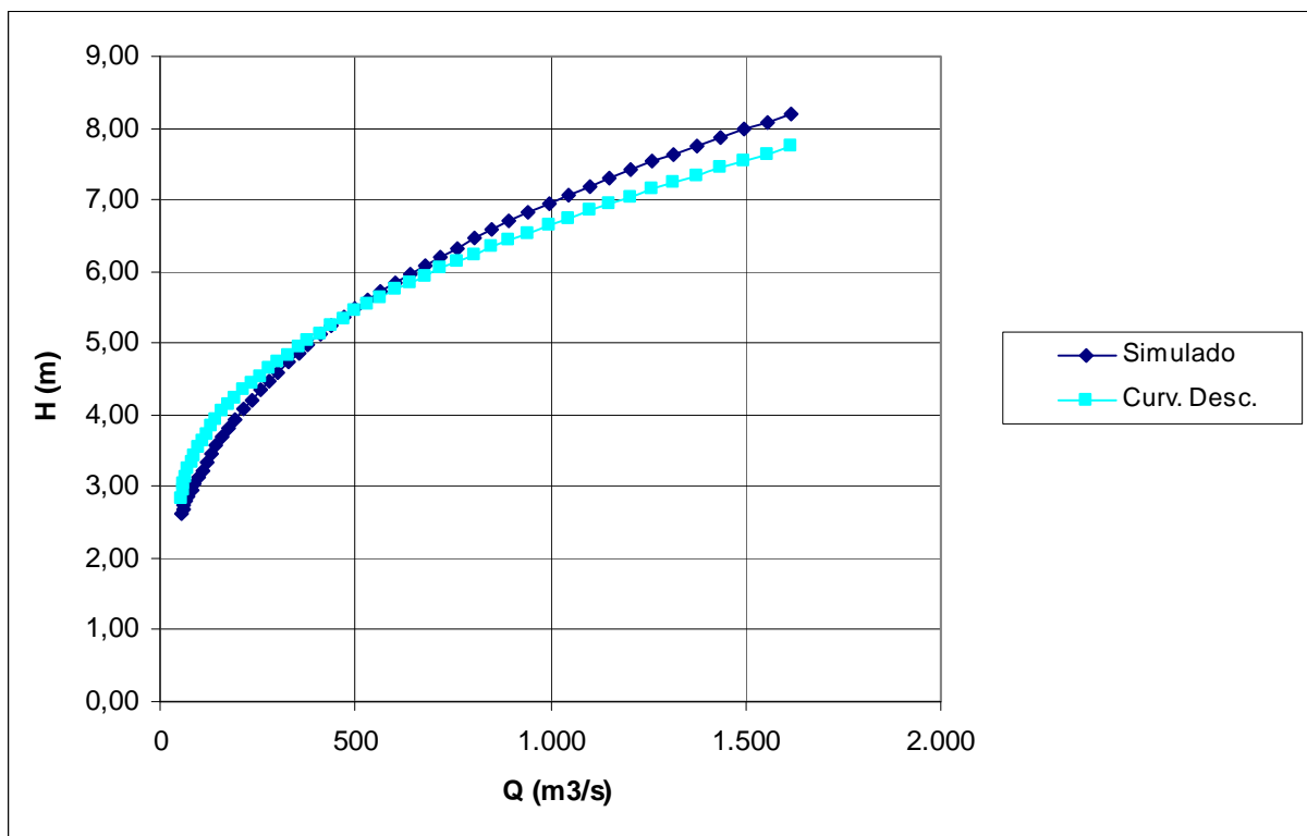
FIGURA 8.3-4 RESULTADOS CALIBRACIÓN ESTACIÓN FLUVIOMÉTRICA
