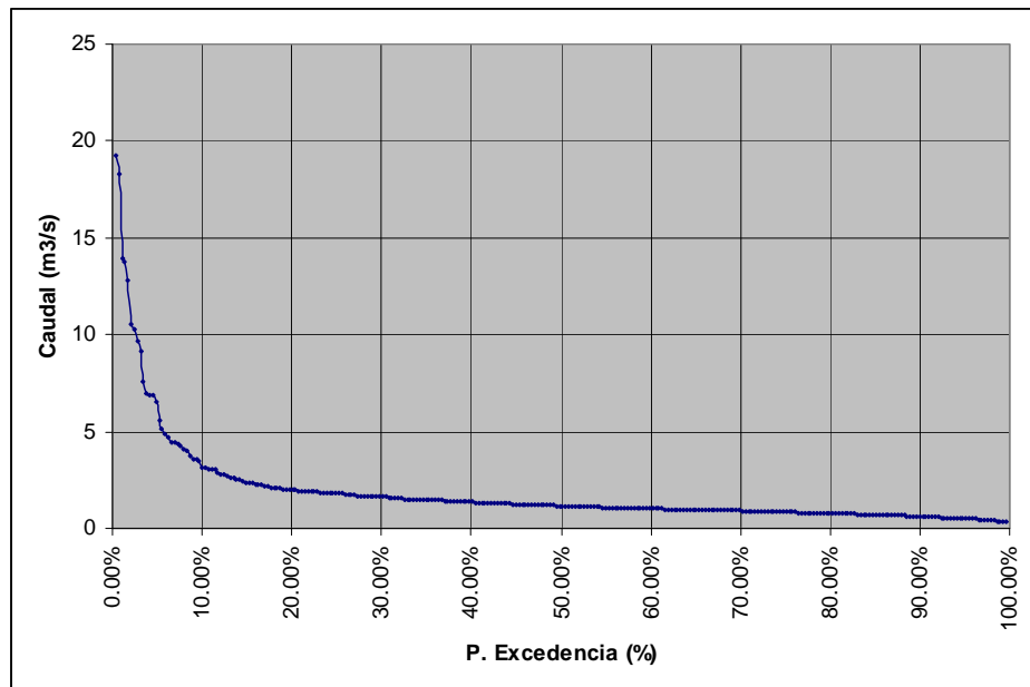
FIGURA 6.1-10 CURVA DE DURACIÓN EN PUNTO DE CONTROL 3, SECTOR SOL NACIENTE, TRAMO INICIAL
