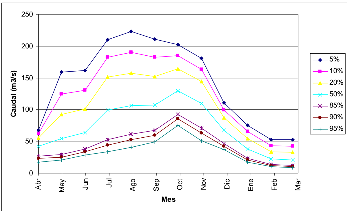
FIGURA 6.4-9 CURVA DE VARIACIÓN ESTACIONAL EN PUNTO DE CONTROL 3, SECTOR ANTES JUNTA RÍO MAÑIGUALES, TRAMO FINAL
