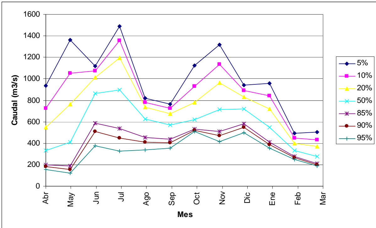
FIGURA 6.2-12 CURVA DE DURACIÓN EN PUNTO DE CONTROL 3, SECTOR LAGO TAGUA-TAGUA, TRAMO FINAL
