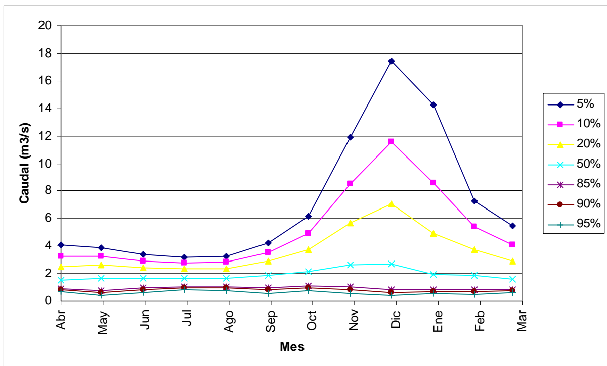
FIGURA 6.1-7 CURVA DE VARIACIÓN ESTACIONAL EN PUNTOS DE CONTROL 2, TRAMO MEDIO
