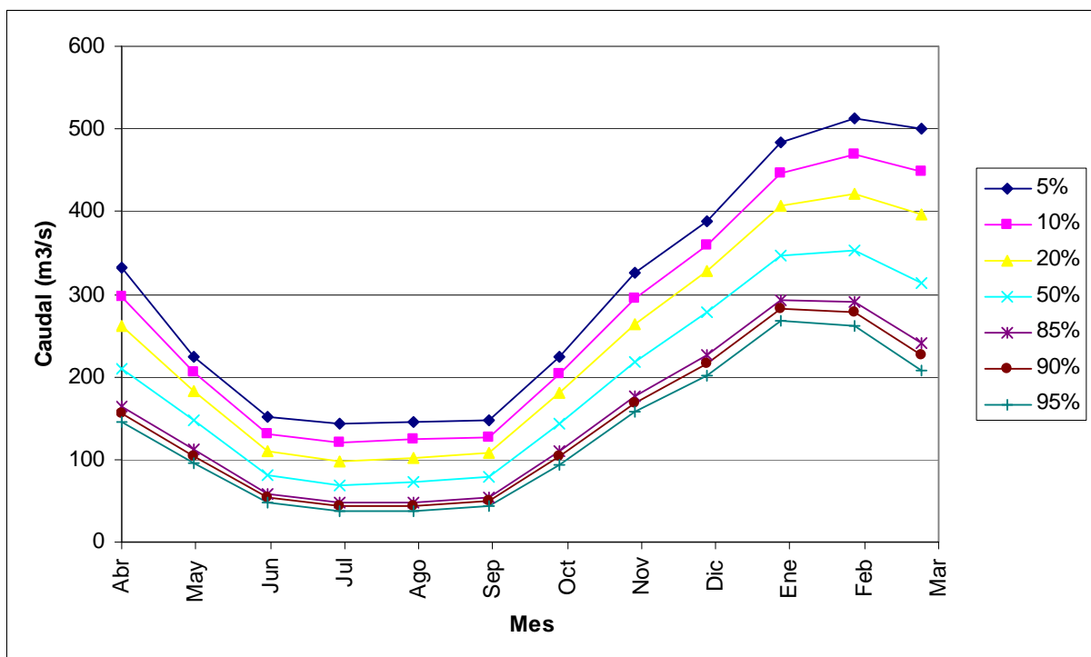
FIGURA 6.6-5 CURVA DE VARIACIÓN ESTACIONAL EN PUNTO DE CONTROL 2, RÍO SERRANO TRAMO MEDIO
