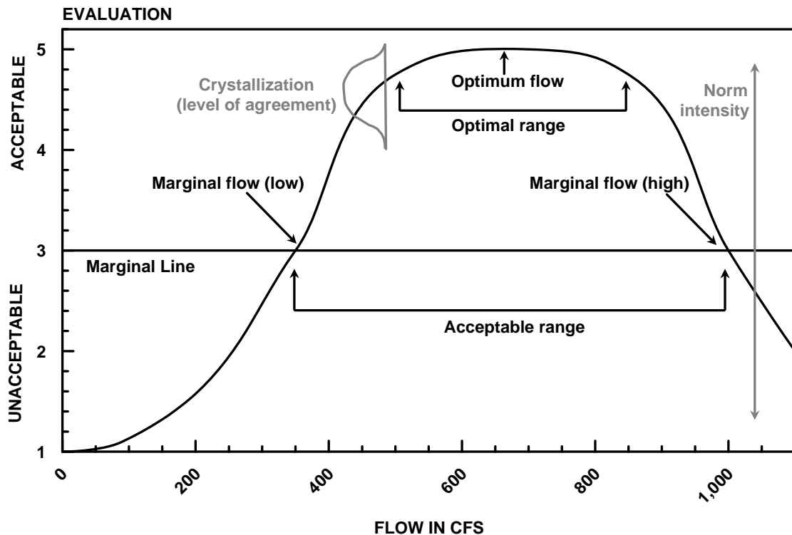
FIGURA 3-13 CURVA DE EJEMPLO DE UN CAUDAL TEÓRICO PARA USOS SEGÚN EL ENFOQUE ESTRUCTURAL
