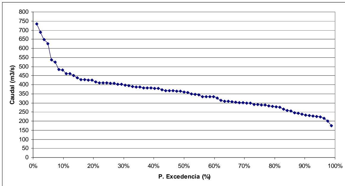
FIGURA 6.3-10 CURVA DE DURACIÓN EN PUNTO DE CONTROL 1, SECTOR FRONTERA, TRAMO INICIAL
