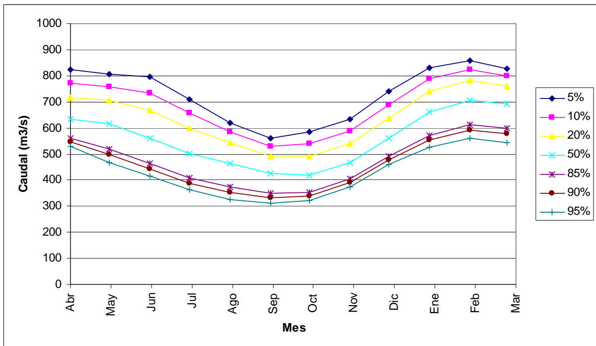
FIGURA 6.5-5 CURVA DE VARIACIÓN ESTACIONAL EN PUNTO DE CONTROL 1, SECTOR CONF. RÍO NEF, TRAMO FINAL.
