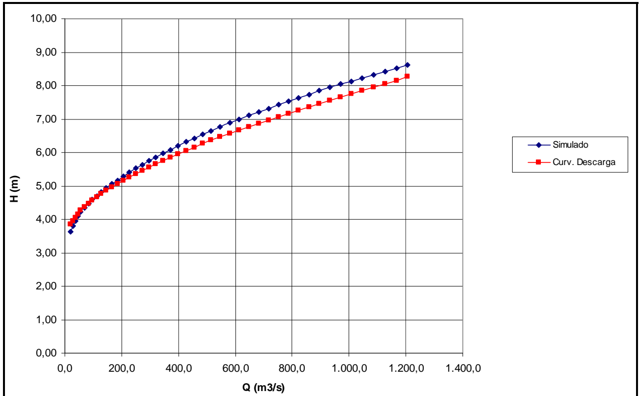
FIGURA 8.4-5 RESULTADOS CALIBRACIÓN ESTACIÓN FLUVIOMÉTRICA FUTALEUFÚ ANTES JUNTA MALITO
