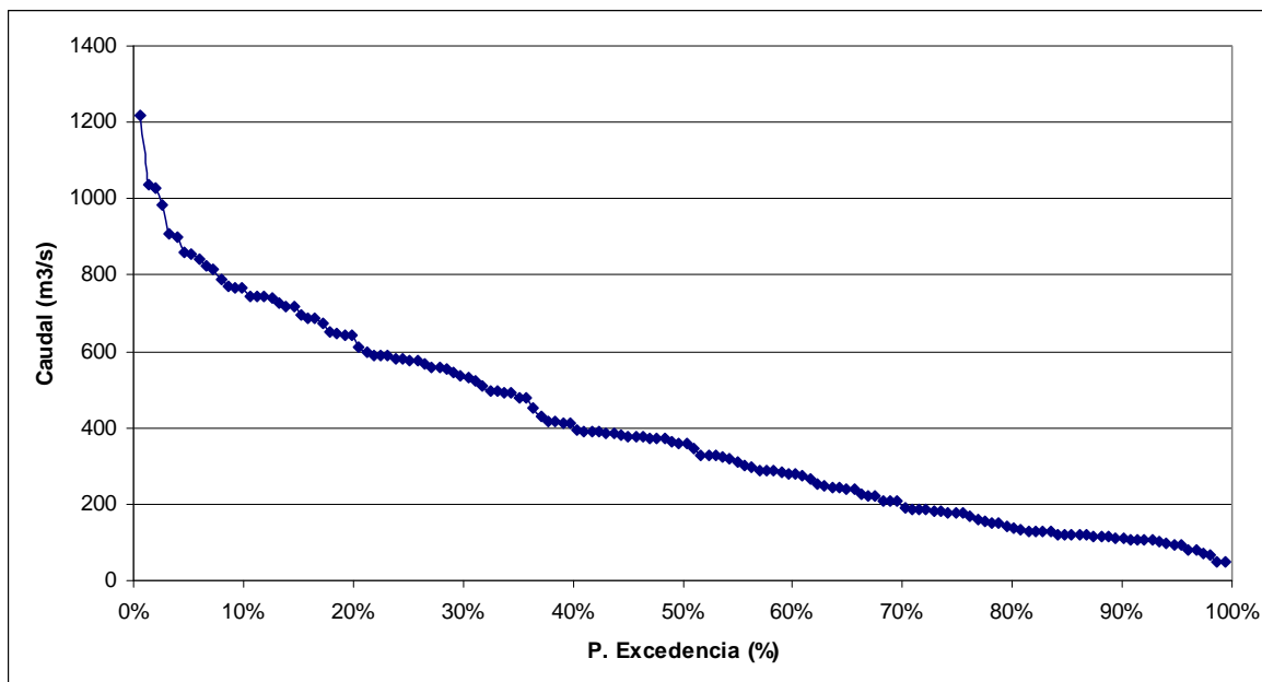
FIGURA 6.6-6 CURVA DE DURACIÓN ESTACIÓN FLUVIOMÉTRICA RÍO SERRANO EN DESEMBOCADURA
