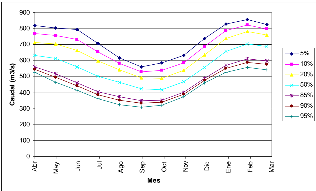
FIGURA 6.5-8 CURVA DE DURACIÓN EN PUNTO DE CONTROL 2, TRAMO MEDIO
