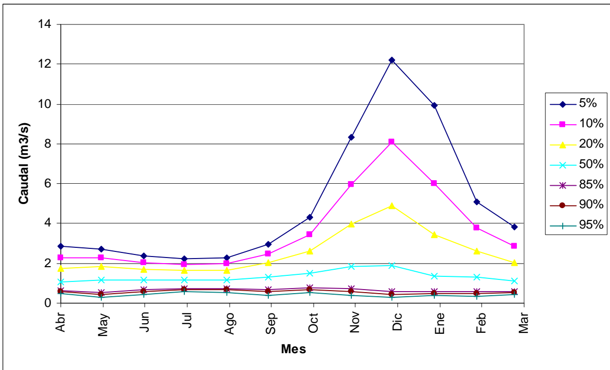
FIGURA 6.1-10 CURVA DE DURACIÓN EN PUNTO DE CONTROL 3, SECTOR SOL NACIENTE, TRAMO INICIAL
