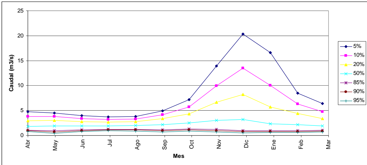
FIGURA 6.1-2 CURVA DE DURACIÓN ESTACIÓN FLUVIOMÉTRICA COCHIGUAZ EN EL PEÑÓN
