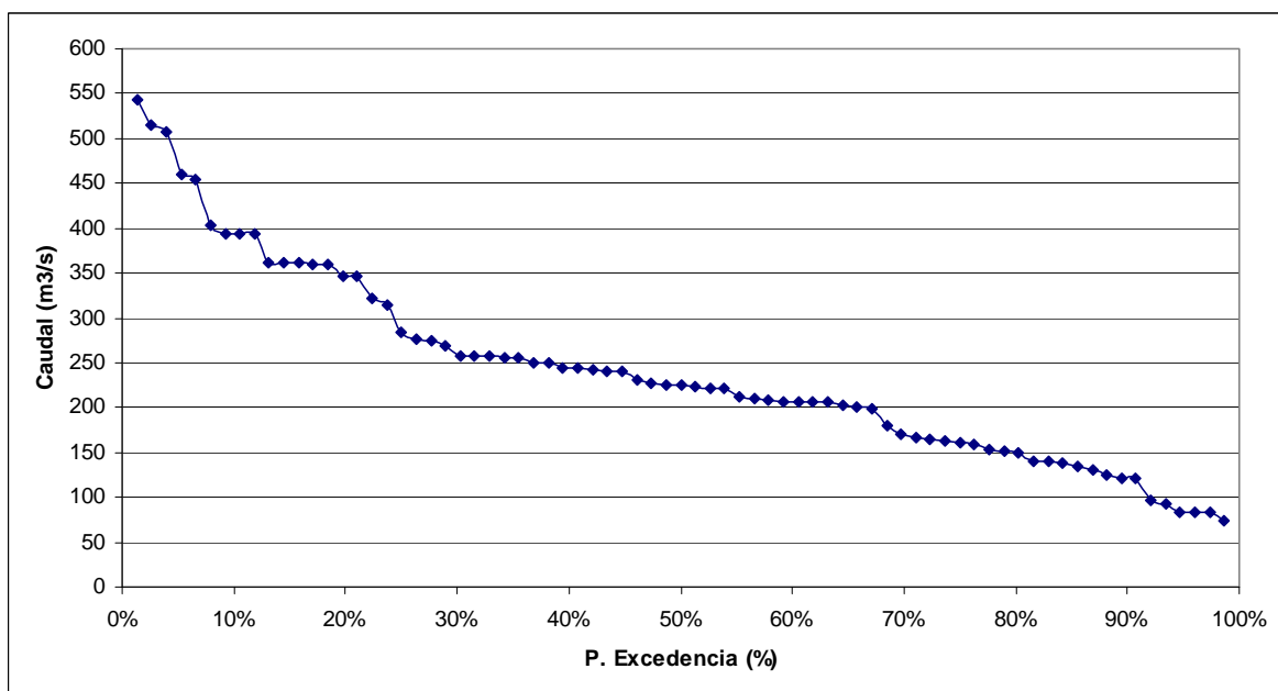
FIGURA 6.2-8 CURVA DE DURACIÓN EN PUNTO DE CONTROL 1, SECTOR FRONTERA, TRAMO INICIAL
