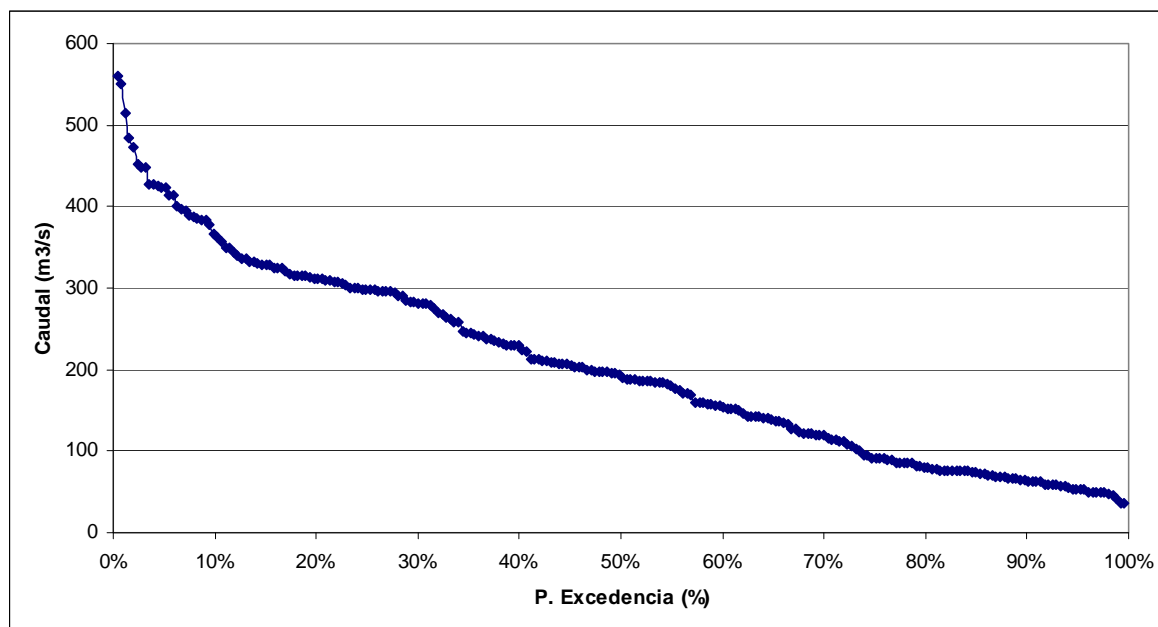
FIGURA 6.6-6 CURVA DE DURACIÓN EN PUNTO DE CONTROL 2, RÍO SERRANO TRAMO MEDIO.
