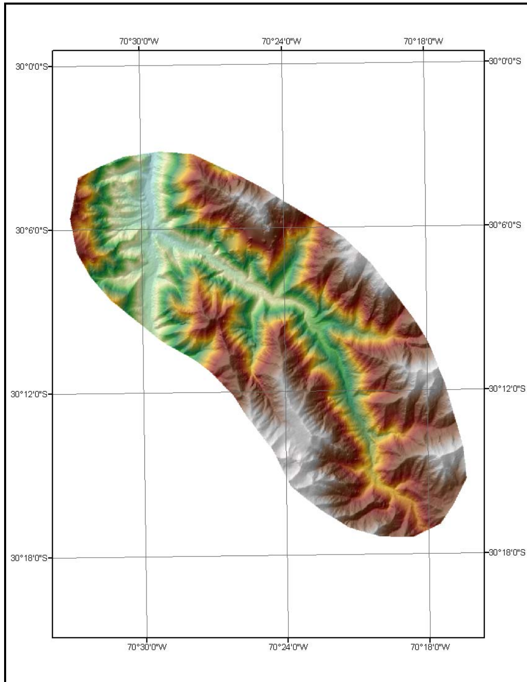
FIGURA 7-5 DEM GENERADO PARA TRAMO DE RÍO COCHIGUAZ
