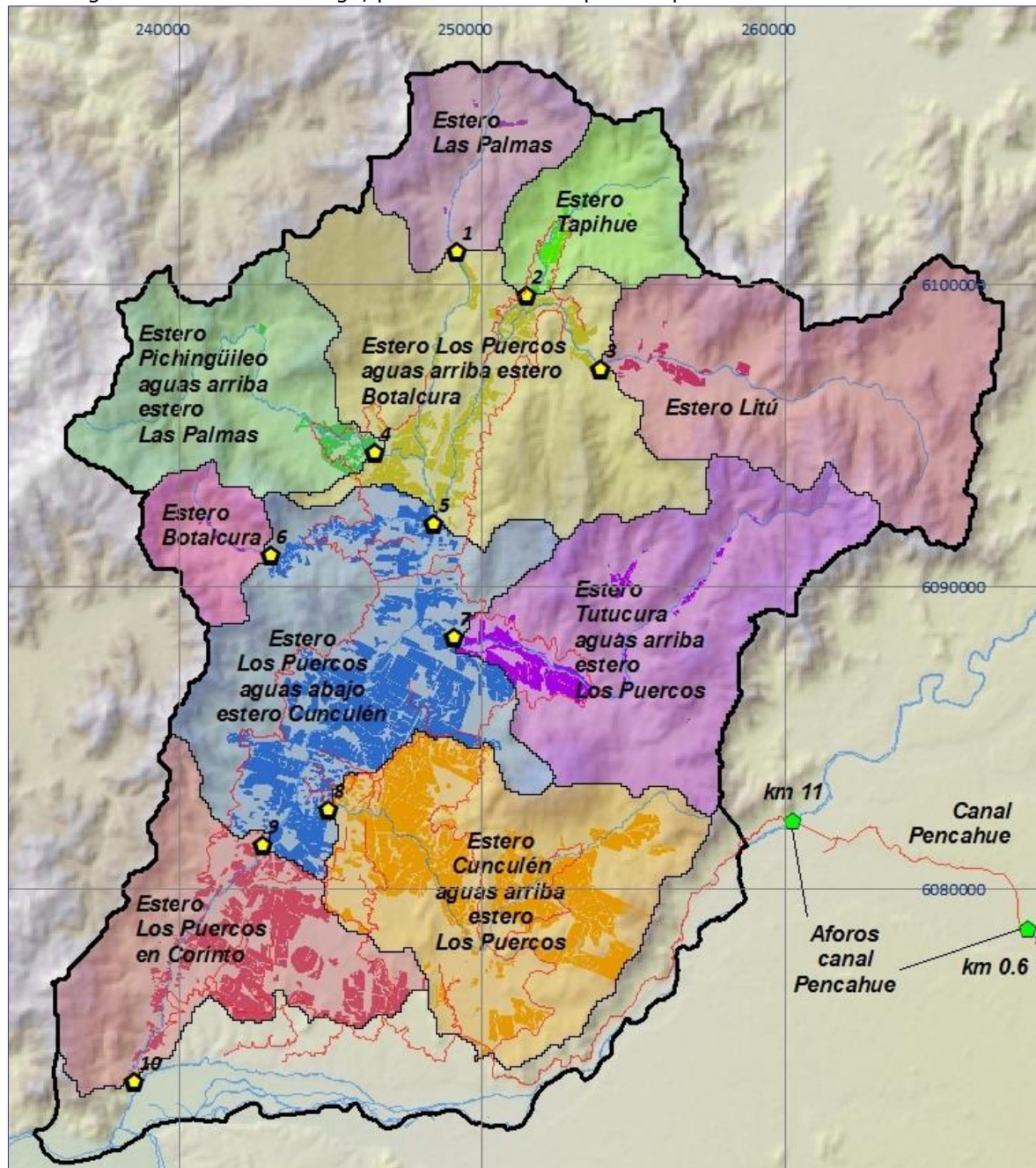
Figura III-9. Áreas de riego, por subcuenca de aporte superficial a secciones de aforo
