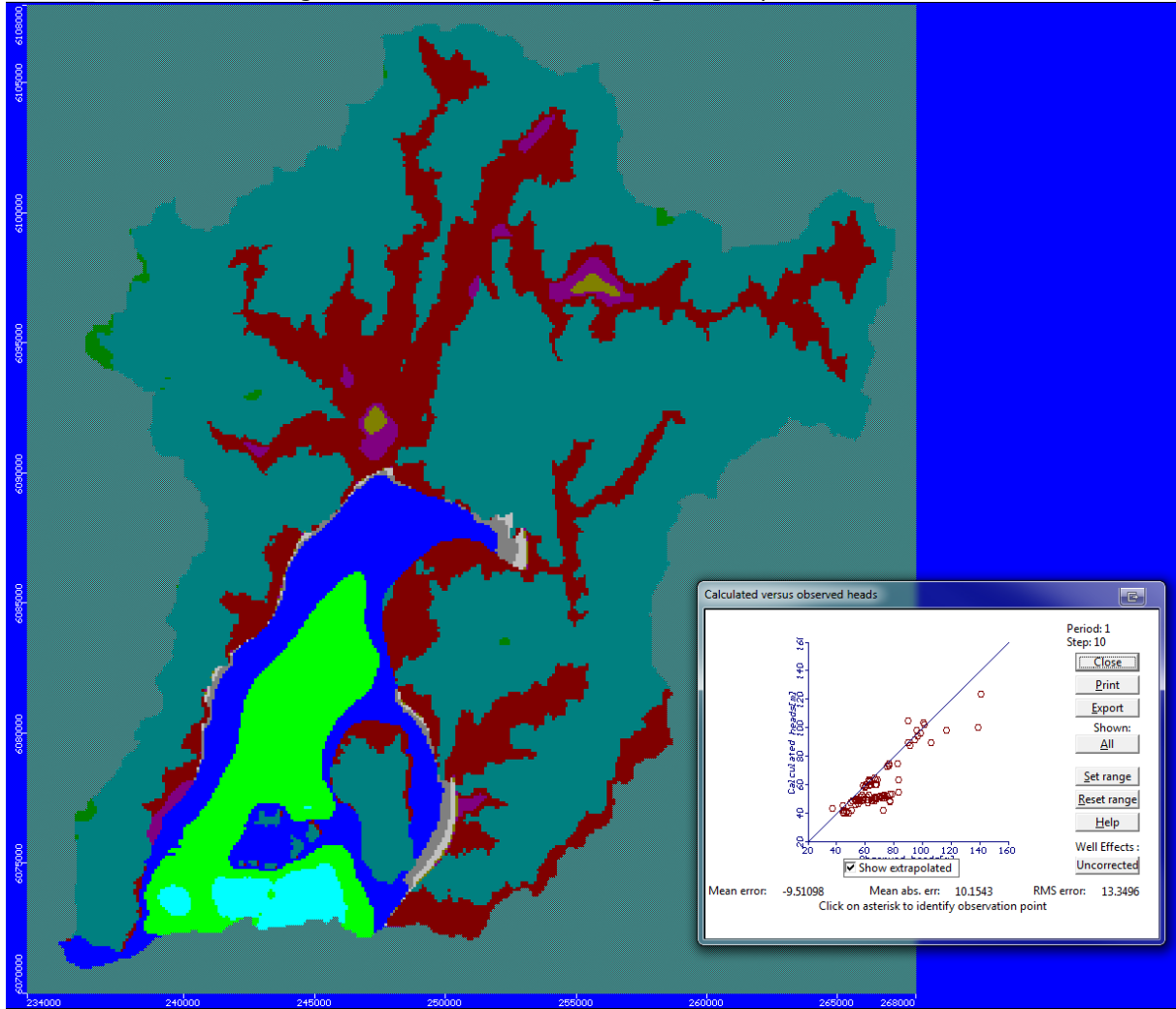
Figura VII-23. Calibración en régimen impermanente
