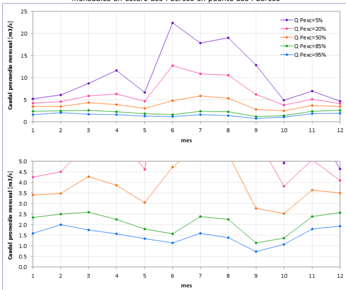
Figura III-7. Curva de variación estacional de caudales promedios mensuales en estero Los Puercos en puente Los Puercos
