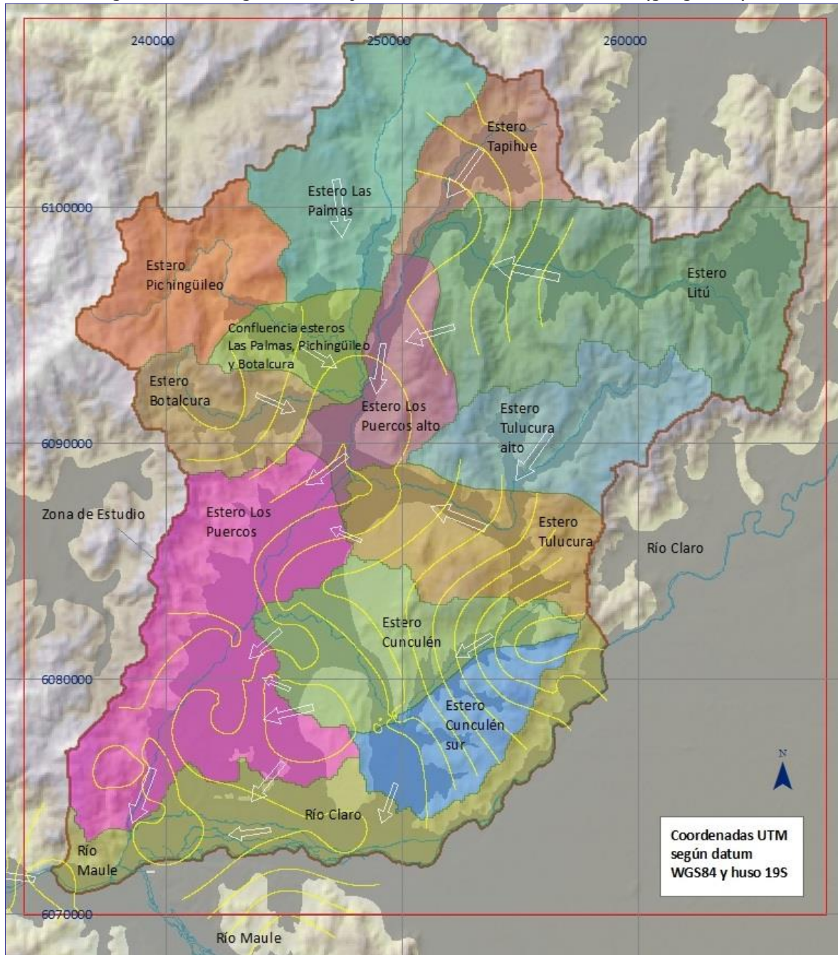
Figura VII-1. Diagrama de flujo subterráneo sistema Pencahue (geográfico)
