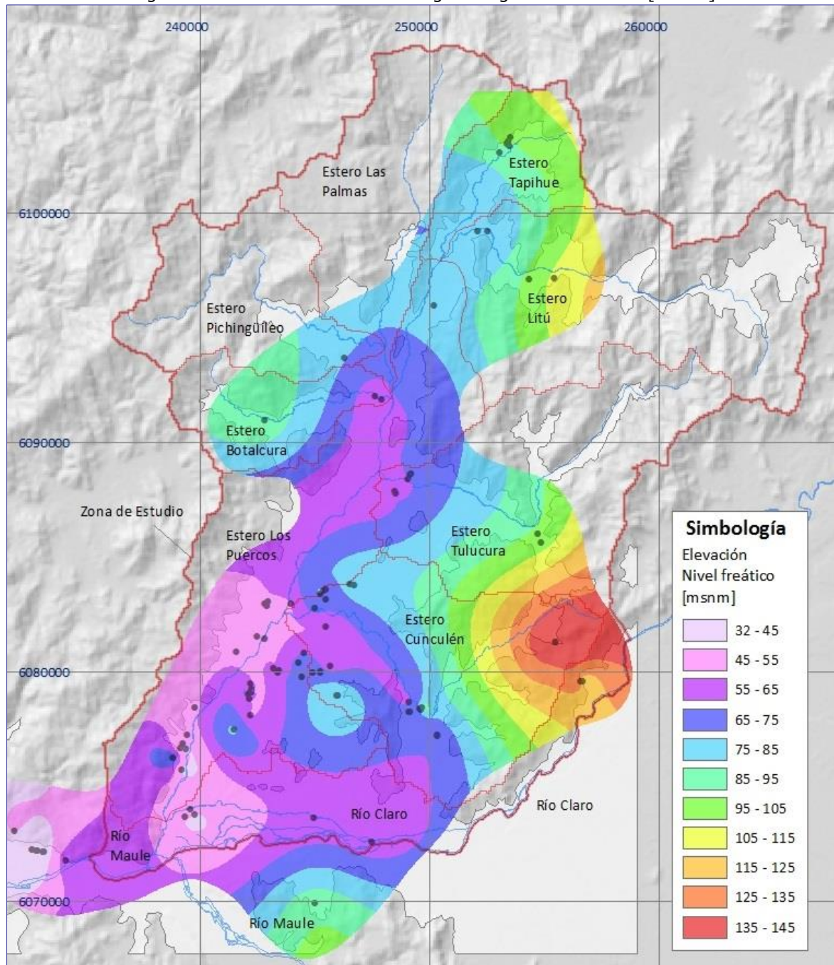
Figura V-11. Curvas isofreáticas según rangos de elevación [msnm]
