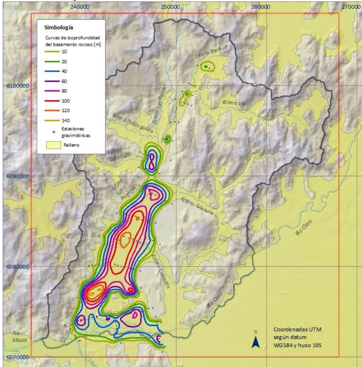
Figura VII-13. Curvas de isoprofundidad del basamento rocoso
