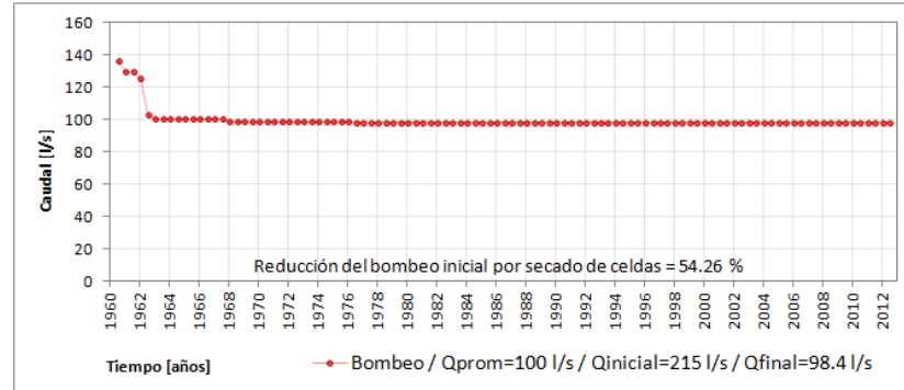
Gráfico VII-9. Flujos principales simulados en escenario 5
