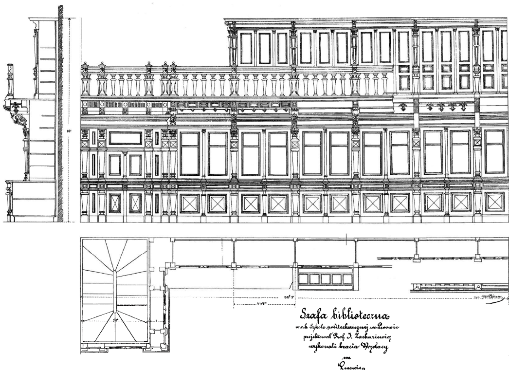
Проект бібліотечної шафи Політехнічної школи у Львові Ю. Захарієвича
