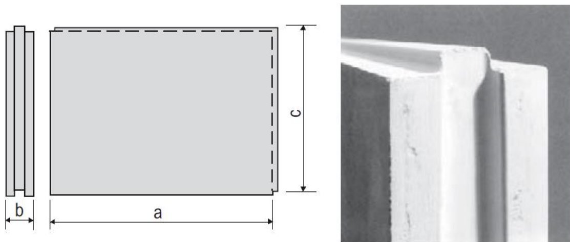
Рис. 1. Паз і гребінь у ГПП
