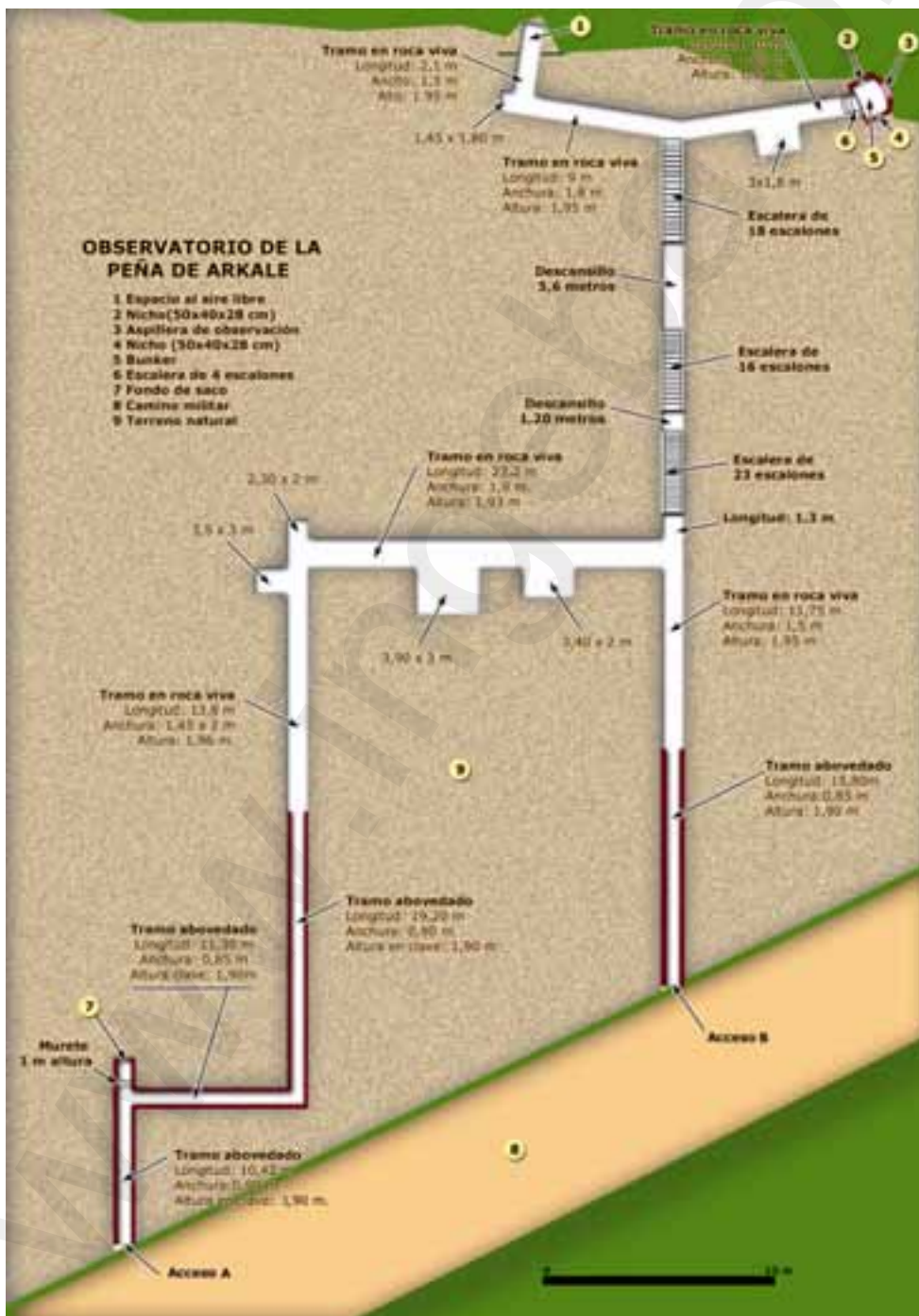
Fig. 77: Observatorio de Arkale. Planta del estado actual.
