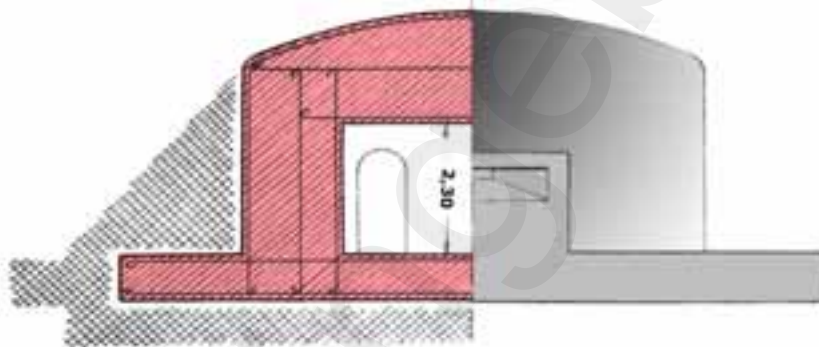
ALZADO
