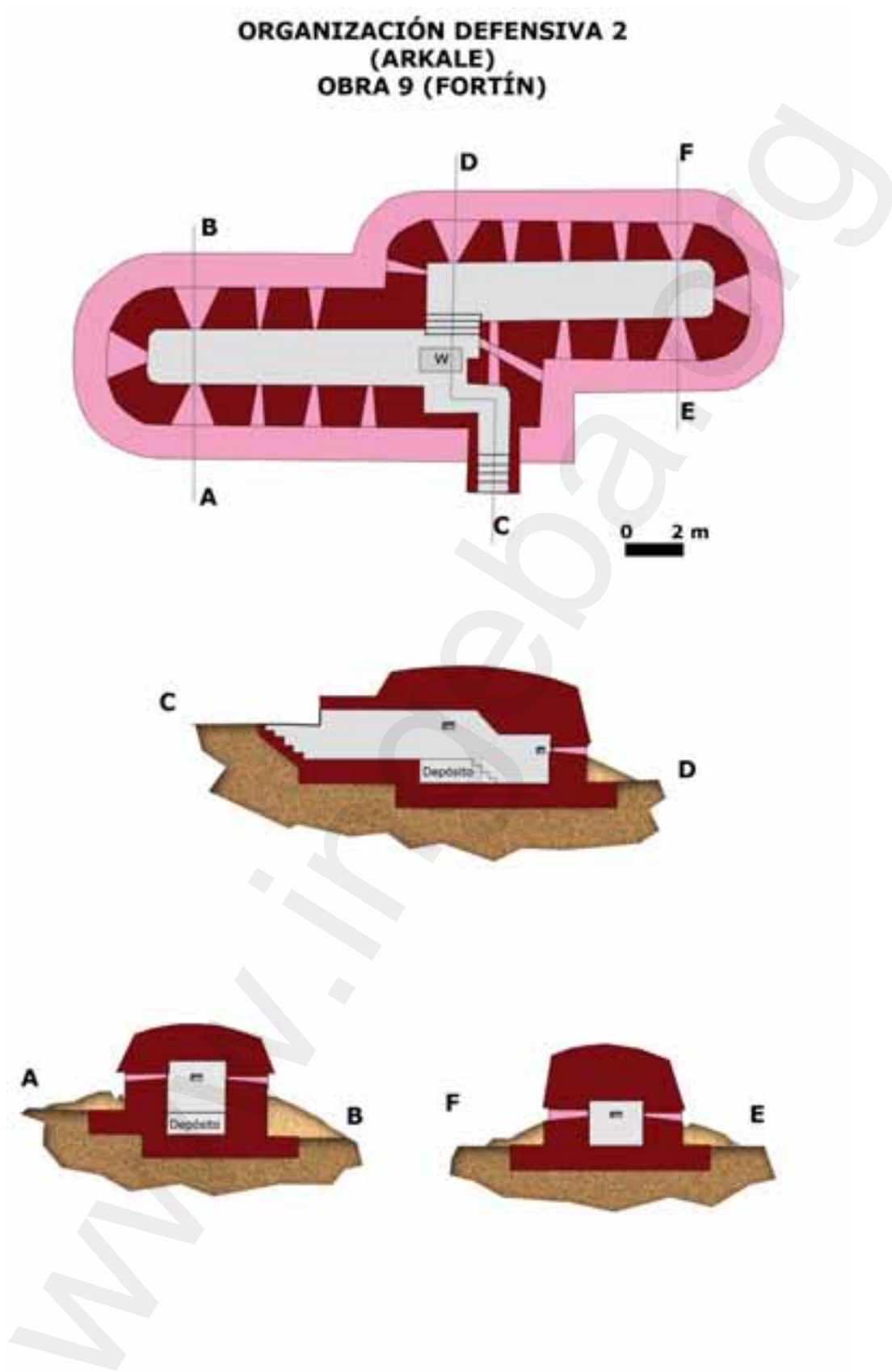
Fig. 58: Organización defensiva n. 2 (Arkale) obra n. 9. Planta y secciones.
