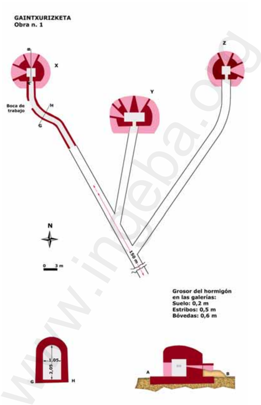
Fig. 31: Organización defensiva n. 1 (Gaintxurizketa) : Obra n. 1
