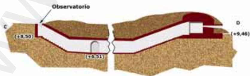
Fig. 24: Organización defensiva n. 1 (Gaintxurizketa) : Obra n. 7 (Secciones)
