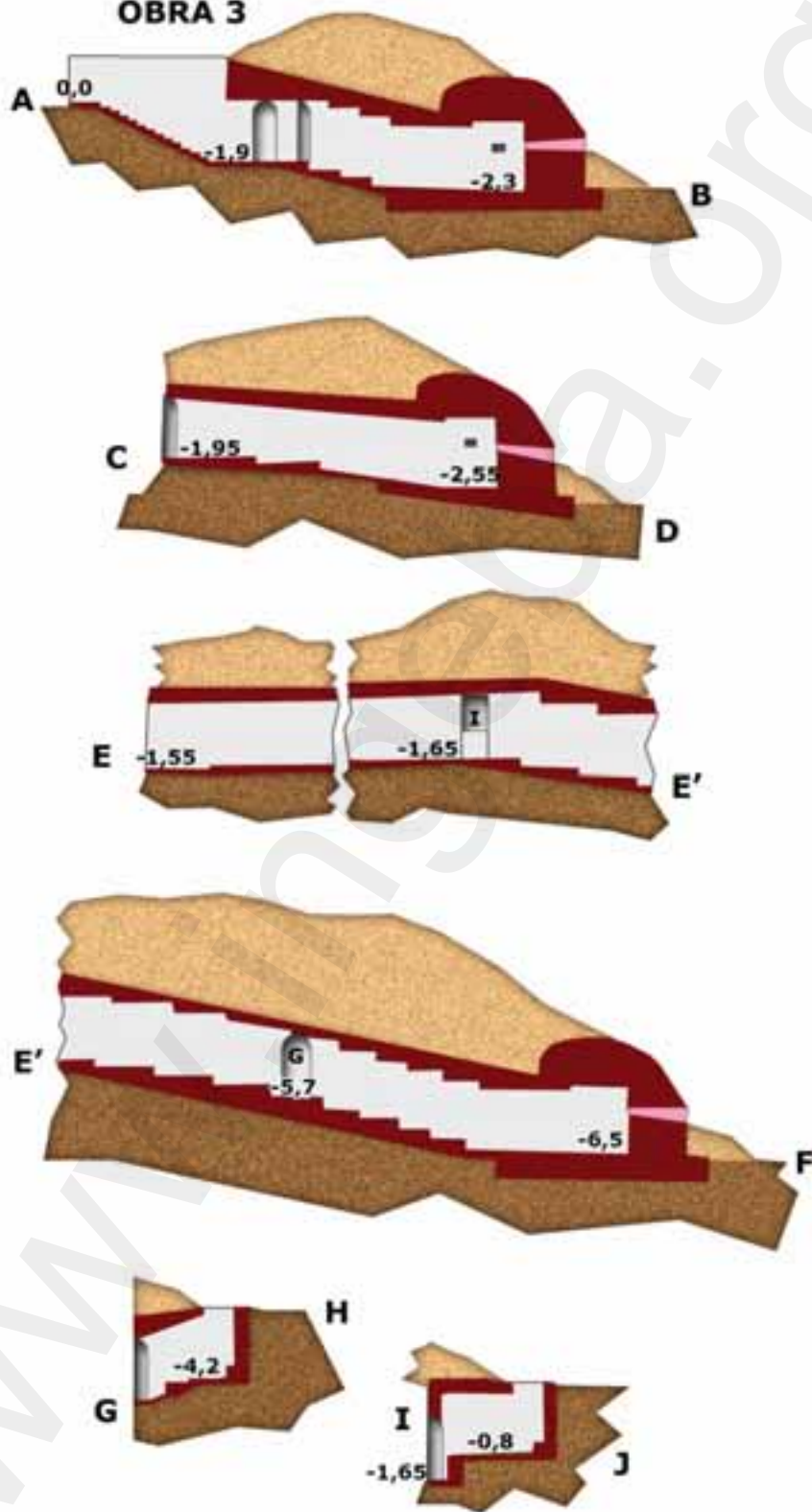
Fig. 45: Organización defensiva n. 2 (Arkale) obra n. 3. Secciones.
