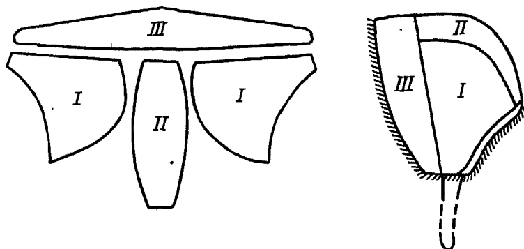
Раскрой мужского мехового капора (с. Ковран, 1963 г.): I — х'вавъм; II — ч'зих'ч; III — ир'ярич, мухта.
