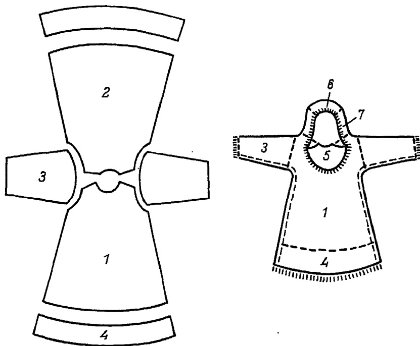
Раскрой современной ительменской меховой курлянки: 1 — увык, к?л'фьян'чран; 2 — сал'ган, краач; 3 — спльн'; 4 — темп-темп; 5 — пыхихэч; 6 — кзихч; 7 — х'вавъм.
