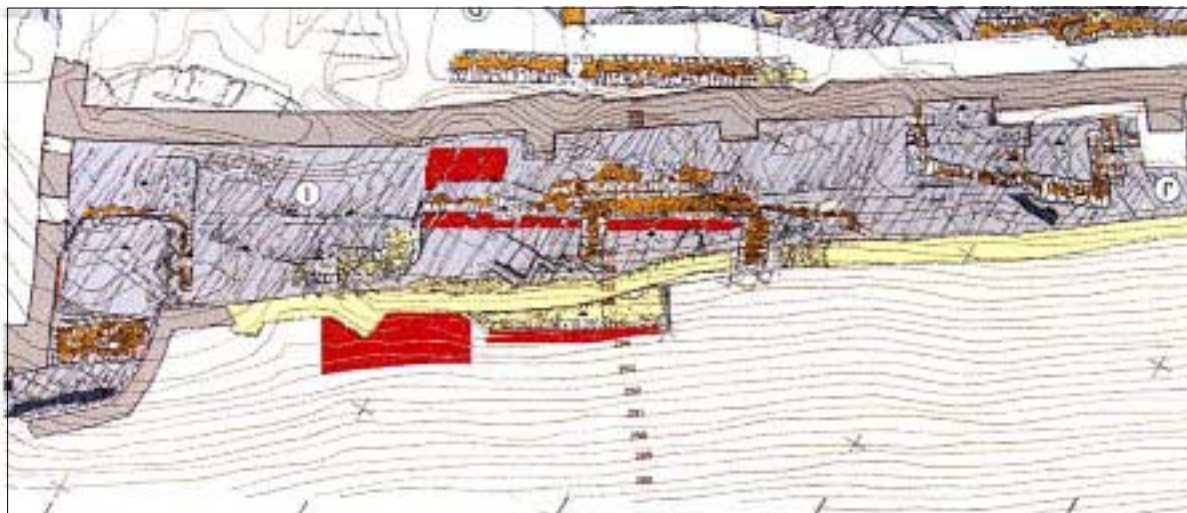
Zones fortement déstabilisées et nécessitant des renforts en béton armé
