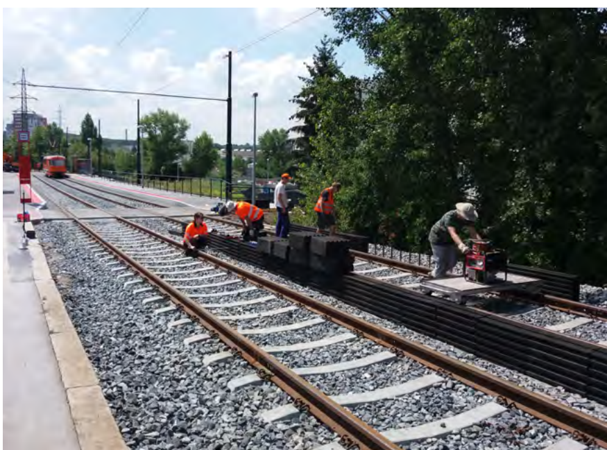
V ÚSEKU KOLEM VOZOVNY HLOUBĚTÍN SE ZA PROVOZU TESTUJE NOVÁ PROTIHLUKOVÁ CLONA Z GUMOVÝCH KVÁDRŮ, JEJÍŽ VÝSTAVBA JE NA SNÍMKU ZACHYCENA
