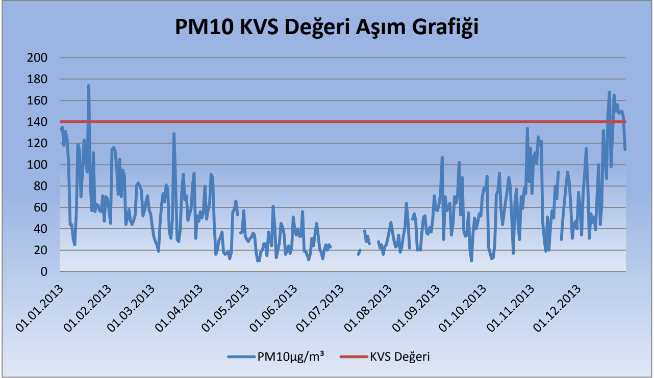
Grafik A.1- İlimizde Hava Kalitesi ölçüm İstasyonu PM10 Parametresi Günlük Ortalama Deęer Grafięi (Kars ÇŞİM, 2013)
