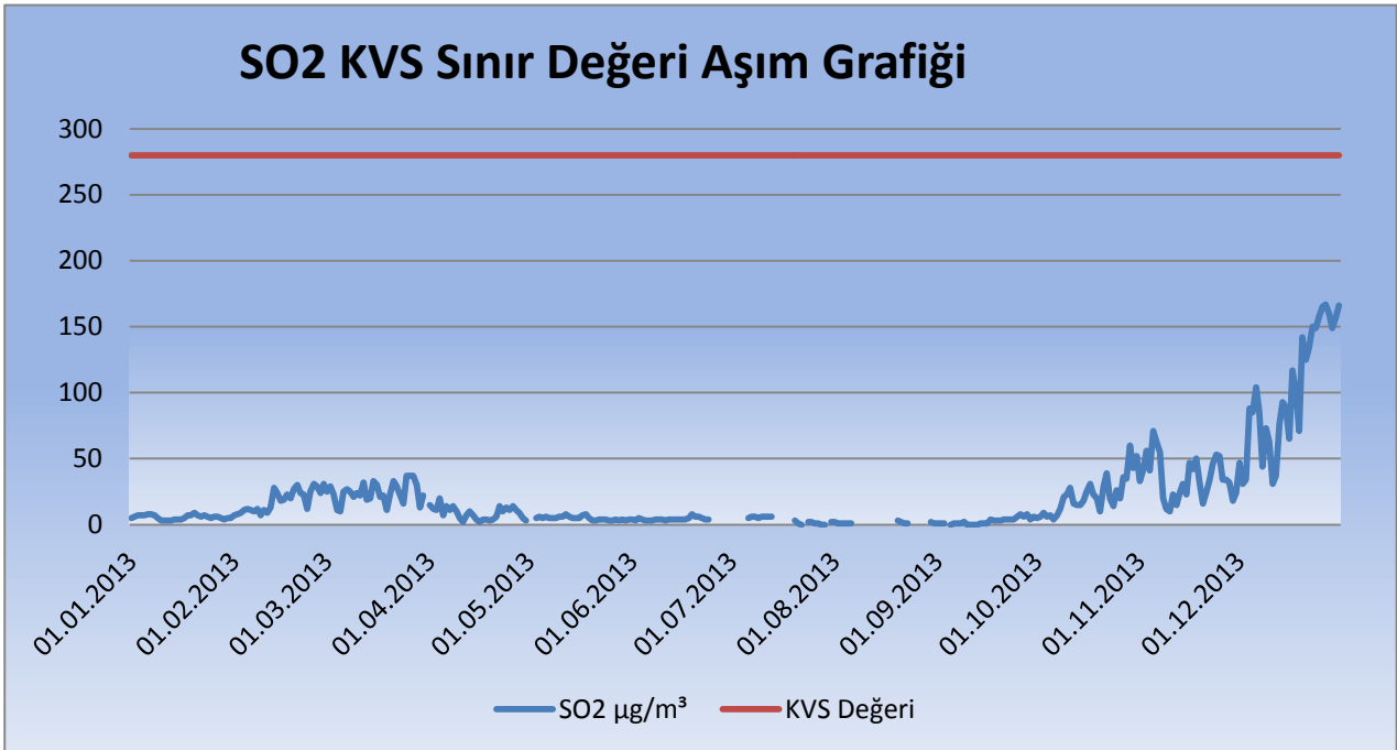
Grafik A.2- İlimizde Hava Kalitesi ölçüm İstasyonu SO2 Parametresi Günlük Ortalama Deęer Grafięi (Kars ÇŞİM, 2013)
