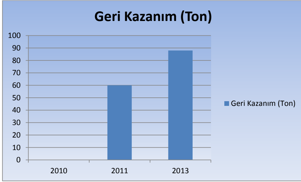
Grafik C.4 – İlimizde Yıllar İtibariyle Atık Akü Toplama ve Geri Kazanım Miktarı (Ton) (Kars Ç.Ş.İ.M., 2014)
