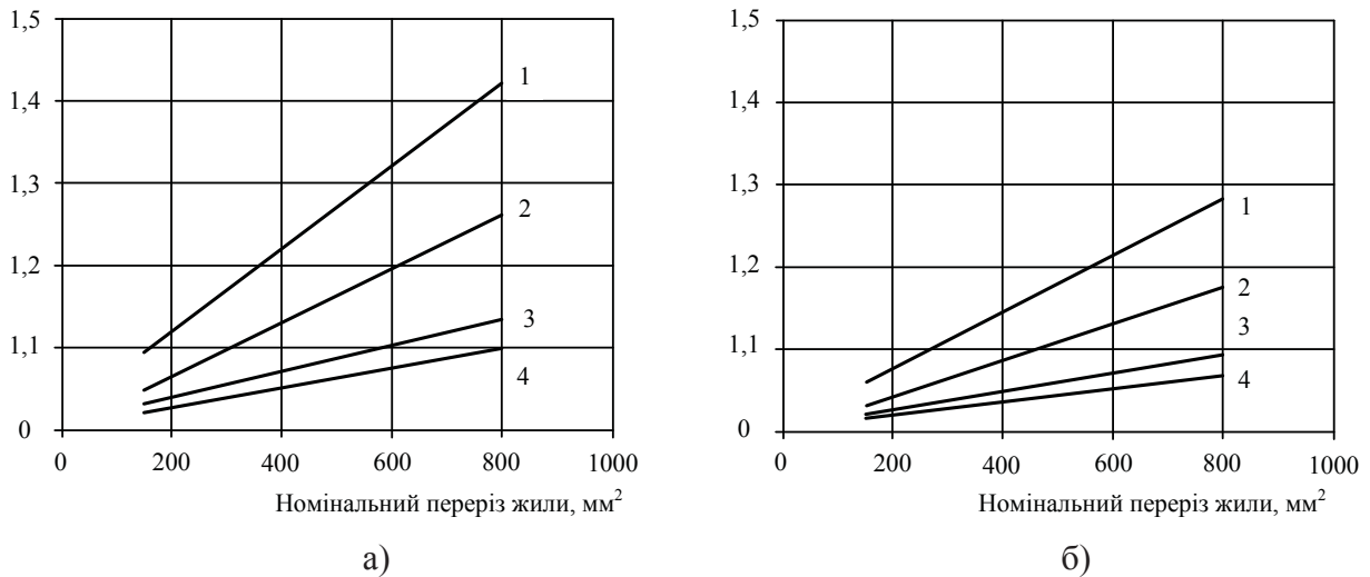
а – для кабелів з мідною жилою; б – для кабелів з алюмінієвою жилою; 1 – кабелі прокладено в землі за схемою «у площині»; 2 – кабелі прокладено в повітрі за схемою «у площині»; 3 – кабелі прокладено в землі за схемою «у трикутник»; 4 – кабелі прокладено в повітрі за схемою «у трикутник»
