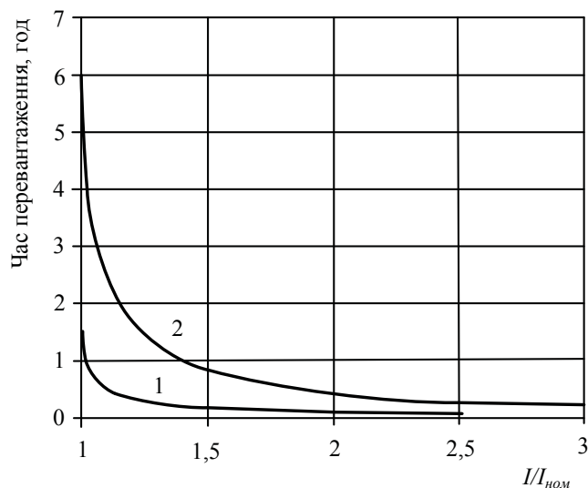
1 – для жили перерізом 35 мм 2 ; 2 – для жили перерізом 800 мм 2
