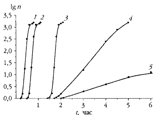
Рис. 3. Изменение концентрации частиц никеля в объеме борогидридного раствора в отсутствие (1) и в присутствии: 2 – окись алкилдиметиламина, 3 – 5-нитробензимидазол, 4 – 6-метилдитиоурацил, 5 – 2,4-дитио-1,2,3,4-тетрагидропиримидин
