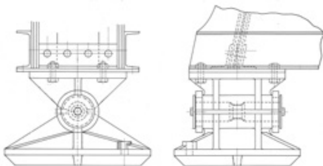
Pendelpilarprinsippet bygger på at pilarene har bevegelige ledd ved topp og fot og dermed kan bevege seg fritt i viaduktens lengderetning. En detalj av Smålensbanens tegning nr. 332 gjengir pilarfotens bevegelige ledd, en horisontal valse som er omsluttet av to lagetskåler. (Foto: Jernbaneverket, bearbeidet av Rolf Tore Arnesen).
