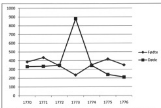
Fig. 3. Fødte og døde i Øvre Borgarsyssel prosti 1770-1776
