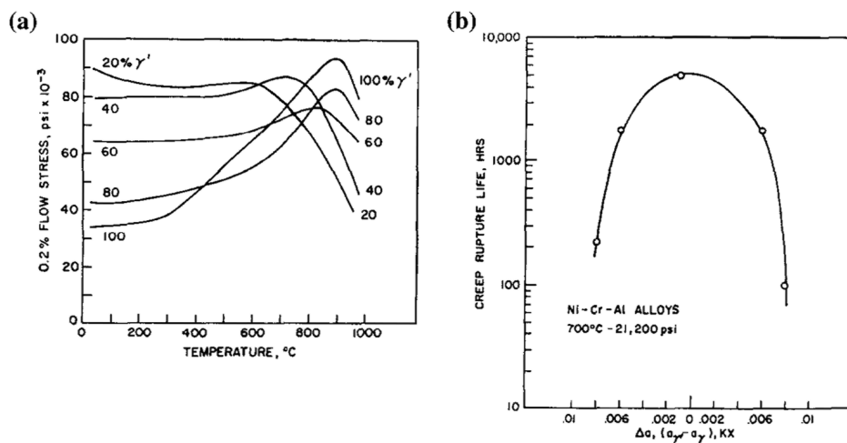
Рис. 9.6. (а) температурная зависимость напряжения течения специального сплава Ni-Cr-Al с различным объемным содержанием фазы гамма-штрих (по Beardmore et al. 1969). (б) Влияние рассогласования параметра решетки в КХ (эквивалентно \text{\AA} ) на значение времени, требуемое для разрушения сплава деформацией ползучести (по Mirkin and Kancheev 1967)
