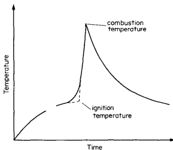
Рис. 11.2. Схематическое изображение эпюры изменения температуры при синтезе TiC_x
