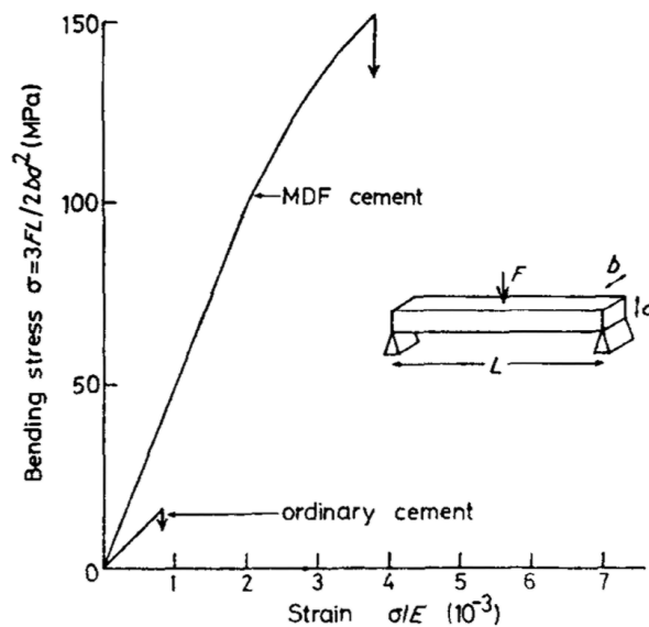
Рис. 9.12. Прочность при изгибе обычного цемента и цемента, свободного от макродефектов (по Birchall et al. 1982)
