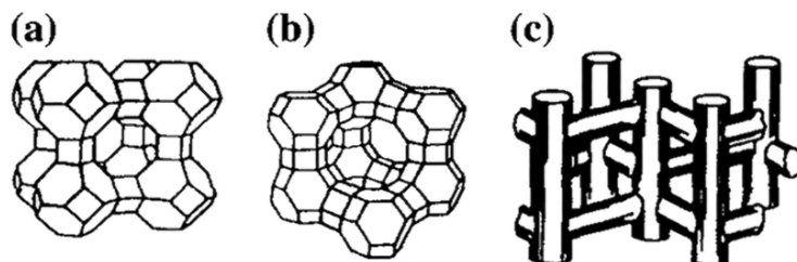
Рис. 10.4. Схемы структур (а) цеолита А, (b) гомологичного ему фожасита, (с) схема «трубчатого» цеолита ZSM-5
