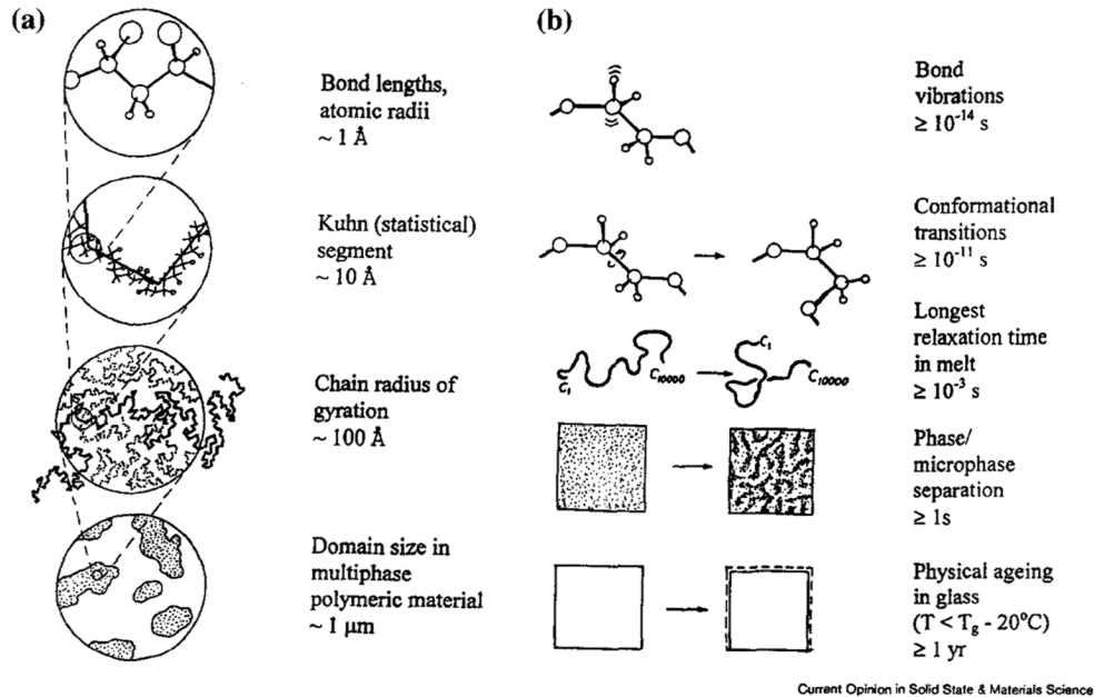
Рис. 12.4. Иерархия масштабов размеров структур и временных масштабов движения в полимерах. T_g – температура стеклования (по Uhlherr and Theodorou 1998) (изображение предоставлено издательством Elsevier Science)
