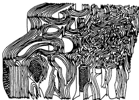
Рис. 11.5. Модель структуры углеродного волокна на основе полиакрилонитрила (по Johnson 1994)
