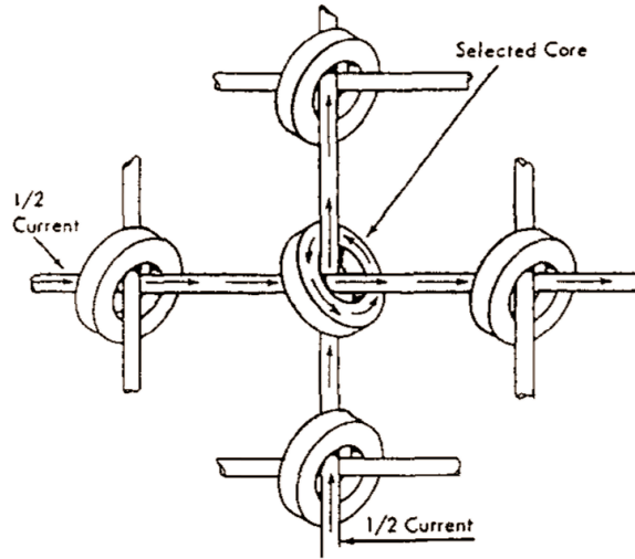
Рис. 7.9. Фрагмент памяти на магнитном сердечнике (по IBM News, 1967)
