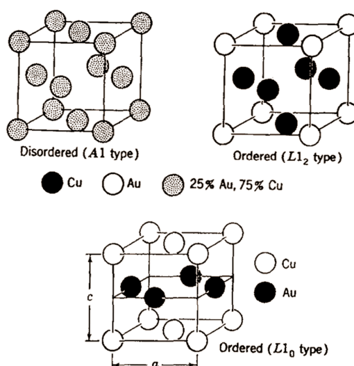
Рис. 3.17. Расположение атомов в сплавах Cu-Au
