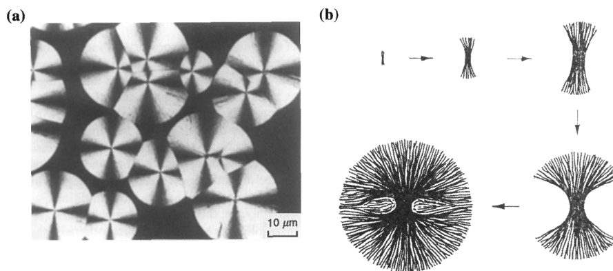
Рис. 8.1. (а) Сферолиты, растущие в тонкой пленке изотактического полистирола, увиденные с помощью оптического микроскопа с пересекающимися полярами (из Bassett, 1981, по Keith, 1963). (б) Схема роста сферолитов (по Bassett 1981). Волокна состоят из зигзагообразных цепей полимеров
