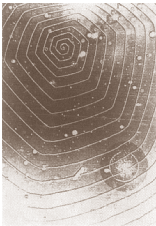
Рис. 3.23. Рост по спирали кристалла карбида кремния, начинающийся в точке возникновения винтовой дислокации (изображение предоставлено профессором С. Амелингом)
