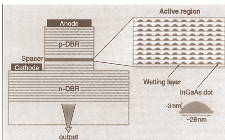
Рис. 7.5. Полупроводниковый плоскостной лазер с вертикальным резонатором на квантовых точках, активный слой которого состоит из самоупорядоченных квантовых точек \text{In}_{0,5}\text{GaAs}_{0,5} (Fasor, 1997)
