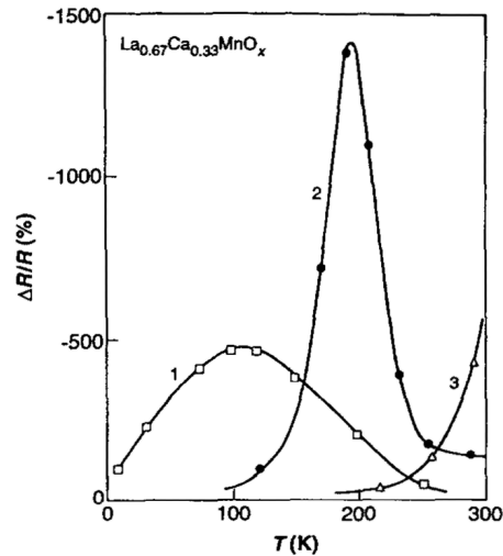
Рис. 11.4. Три графика кривых отношения \Delta R к R для пленки La-Ca-Mn-O: (1) осажденной, (2) выдержанной в течение получаса при температуре 700^\circ\text{C} в кислороде; (3) выдержанной в течение трех часов при 900^\circ\text{C} в кислороде (по Jin et al. 1993, рис. предоставлен журналом «Science»)
