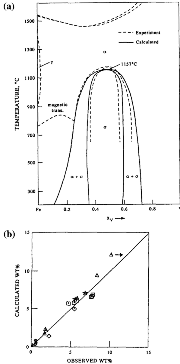
Рис. 12.6. (a) Рассчитанные и полученные в результате эксперимента графики границы ( \alpha+\sigma ) фазы Fe-V (по Spenser and Putland 1973). (b) Сравнение между рассчитанными и экспериментальными величинами концентрации Al, V и Fe в двух фазах в сплаве Ti-6Al-4V (по Saunders and Miodownik 1998)
