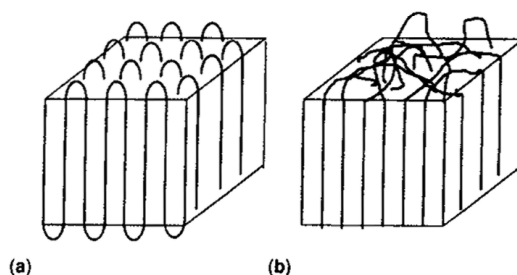
Рис. 8.4. Схема расположения перегибов цепей в монокристалле полимера. (a) упорядоченная модель; (b) неупорядоченная модель
