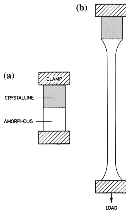
Рис. 8.10. Образец каучука, подвергнутый обработке с тем расчетом, чтобы одна его половина сделалась кристаллической, а другая аморфной. При нагружении заметному растяжению подвергается только аморфная часть (по Treloar 1970)
