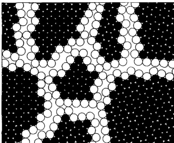
Рис. 10.2. Схема микроструктуры наноструктурного монофазного материала (по Gleiter 1996)
