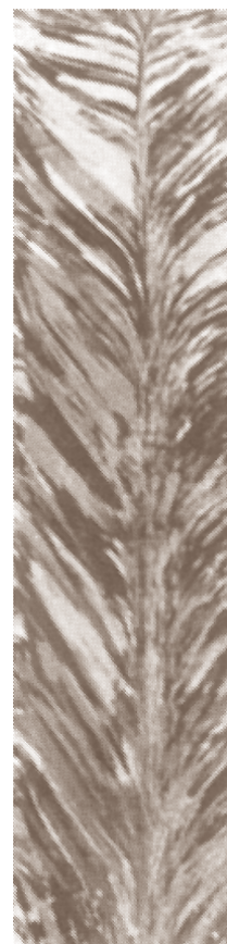
Рис. 3.9. Макроструктура слитка
