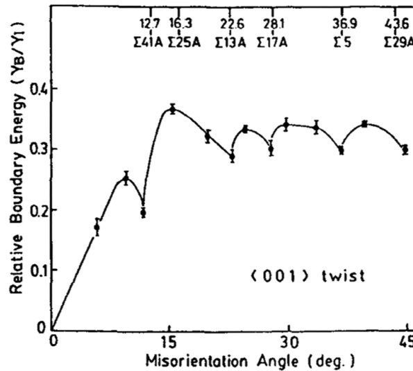
Рис. 9.9. Зависимость энергии зеренных границ в меди от угла их разориентировки (по Miura et al. 1990)
