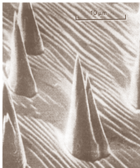
Рис. 6.6. Полученное с помощью сканирующего электронного микроскопа изображение поверхности кристаллов олова, подвергшихся бомбардировке ионами аргона с энергией 5 кэВ (Stewart and Thompson, 1969).
