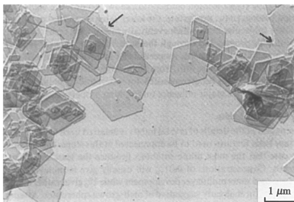
Рис. 8.2. Ромбовидные монокристаллы полиэтилена, выращенные из раствора с помощью метода для выращивания монослойных кристаллов. Снимок получен с помощью электронного микроскопа (по Bassett 1981)
