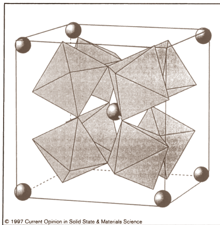
Рис. 7.6. Структура кристалла антимонида скуттерудита. Атом переходного металла (Fe или Co), расположенный в центре каждого октаэдра, связан с атомами сурьмы, находящимися в его вершинах. Редкоземельные атомы (малые сферы) расположены в «ячейках», образованных восемью октаэдрами. По-видимому, именно большая амплитуда колебаний редкоземельных атомов в их ячейках является причиной удивительно низкой теплопроводности этого материала (Sales, 1997)
