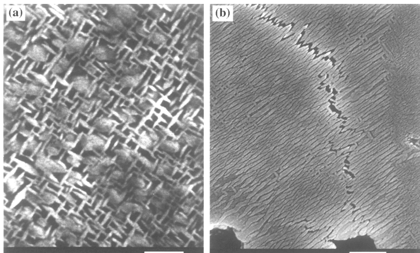
Рис. 9.13. (а) Полученный с помощью просвечивающего электронного микроскопа снимок ZrO_2 с примесью MgO , посредством старения доведенного до максимальной прочности. Видны тетрагональные частицы на гранях куба; кубическая матрица протравлена плавиковой кислотой. Масштаб 0,5 \mu m . (б) Полученный с помощью сканирующего электронного микроскопа снимок перестаренного и подвергнутого нагружению образца ZrO_2 с примесью MgO с крупными частицами. На снимке видны сильное отклонение направления трещины и образование перемычек. Масштаб 2,5 \mu m (снимки предоставлены доктором Р. Г. Дж. Ханнинком)
