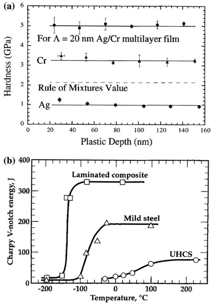
Рис. 10.6. (а) Нанотвердость на вдавливание мультислоев серебро/хром и отдельных пленок этих металлов как функция от глубины ямки, полученной в результате пластической деформации. (б) Ударная вязкость по Шарпи, температурная зависимость трещиностойкости трех материалов: малоуглеродистой стали, высокоуглеродистой стали и многослойного композита из этих двух видов стали (графики предоставлены доктором Дж. Водсвортом) (рис. 10.6 (б) взят из книги [Kum et al. 1983])
