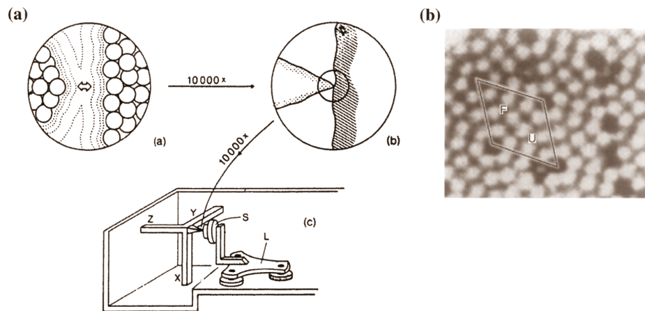
Рис. 6.9. (а) – Схема изобретенного Биннигом и Рорером сканирующего туннельного микроскопа. (б) – Изображение «7x7» поверхностной структуры в плоскости {111} кремния, полученное Хамерсом и другими с помощью сканирующего туннельного микроскопа (Hamers et al., 1986)
