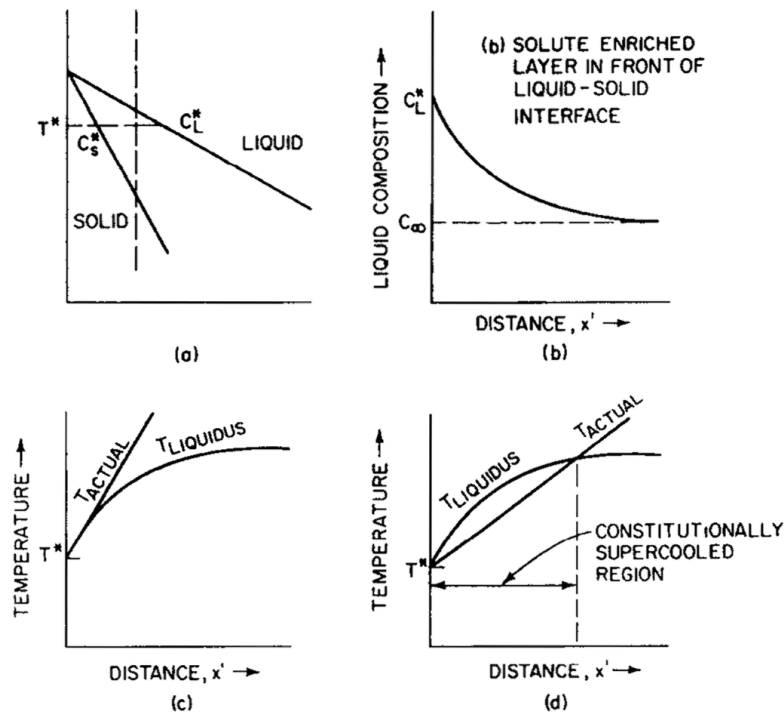
Рис. 9.2. Переохлаждение в ходе затвердевания сплава: (а) фазовая диаграмма; (б) слой с повышенным содержанием растворенного вещества на границе твердое тело – жидкость; (с) условия, при которых граница устойчива; (д) условия, при которых граница неустойчива
