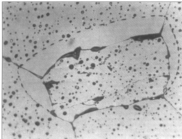
Рис. 9.10. Выполненный с помощью оптического микроскопа снимок уплотненного порошка глинозема на поздней стадии процесса спекания. На нем видны перемещения пор вдоль линии движения зеренной границы. (Большие неупорядочно расположенные поры возникли в результате подготовки образца). Зеренные границы выявлены травлением. Этот снимок выполнен в компании General Electric в конце 1950-х годов и приведен в книге (Burke 1996) (с согласия компании General Electric)
