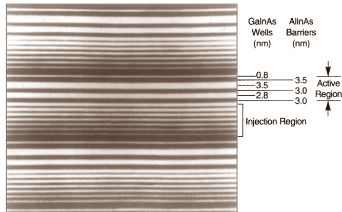
Рис. 7.4. Электронный снимок поперечного разреза квантового каскадного полупроводникового лазера (по Cho 1995)
