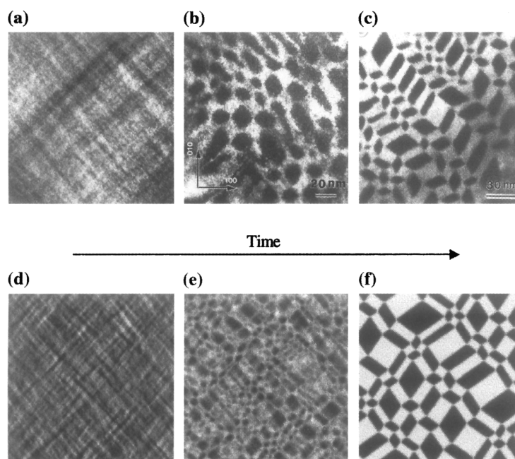
Рис. 12.3. Сравнение между полученными в результате эксперимента (а – с) и численного моделирования (d – f) изображениями «шахматной» микроструктуры, формирующейся в сплаве \text{Co}_{39,5}\text{Pt}_{60,5} , медленно охлажденном от температуры 1023 К до температуры (а) 963 К, (b) 923 К и (с) 873 К. В последнем случае образец был выдержан при температуре 873 К, чтобы изображение стало совершенно четким (по Le Vouar et al. 2000) (фотографии были предоставлены Й. Ле Буаром)
