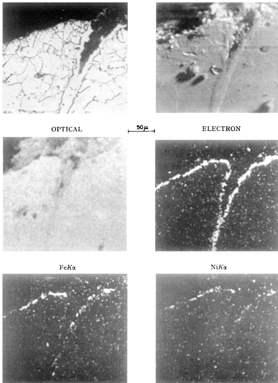
Рис. 6.8. Снимок, сделанный с помощью первой модели сканирующего электронного микроскопа. На фото показаны поверхностные сегрегации примесей Ni, Cu и Sn, растворенных в стали в очень малых концентрациях. Две последние примеси, сегрегирующие на внутренних поверхностях, становятся причиной появления горячих трещин (хрупкости при высоких температурах) и эти исследования прямо продемонстрировали причину этого явления.
