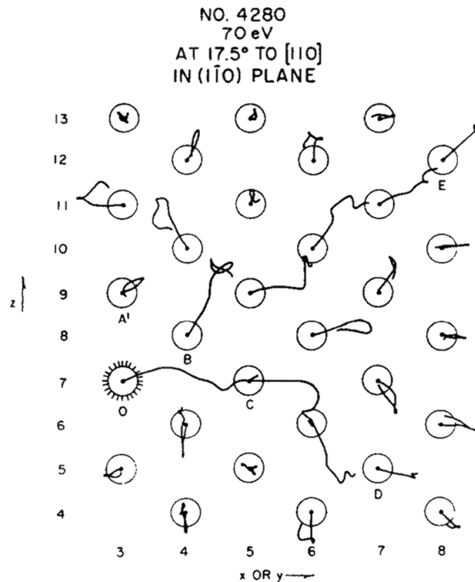
Рис. 12.1. Модель траекторий в каскаде радиационных повреждений в железе (рис. взят из книги Erginsoy et al. 1964)
