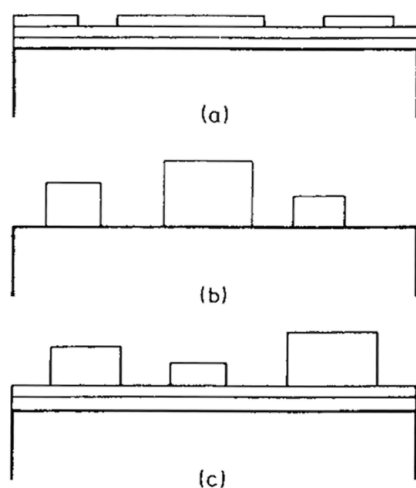
Рис. 10.5. Три модели роста пленок: (а) монослой Франка и Ван-дер-Мерве (двумерный); (б) трехмерный рост Фольмера-Вебера; (с) модель Странски-Крастанова, сочетающая двумерный и трехмерный рост
