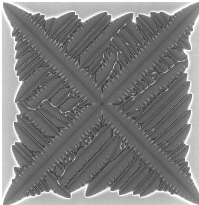
Рис. 9.3. Компьютерная численная модель дендритов, возникающих в сплаве Ni-Cu с содержанием 41 at.% Cu. Локальный состав дендрита можно определить по оттенкам цвета изображения (рис. предоставлен В.Дж. Боэттингером и Дж.А. Уорреном)
