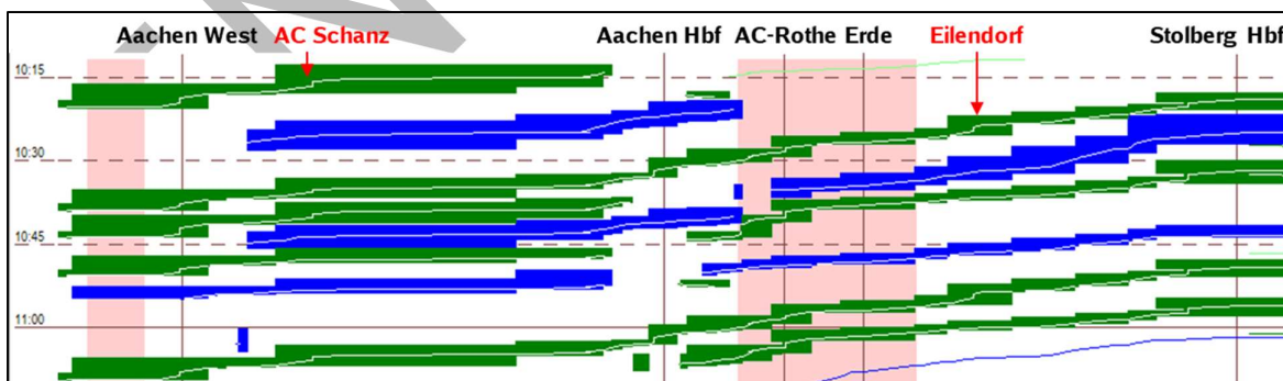
Abbildung 35: Halte von Zügen in Aachen Schanz und Eilendorf verursachen einen erhöhten Kapazitätsverbrauch
