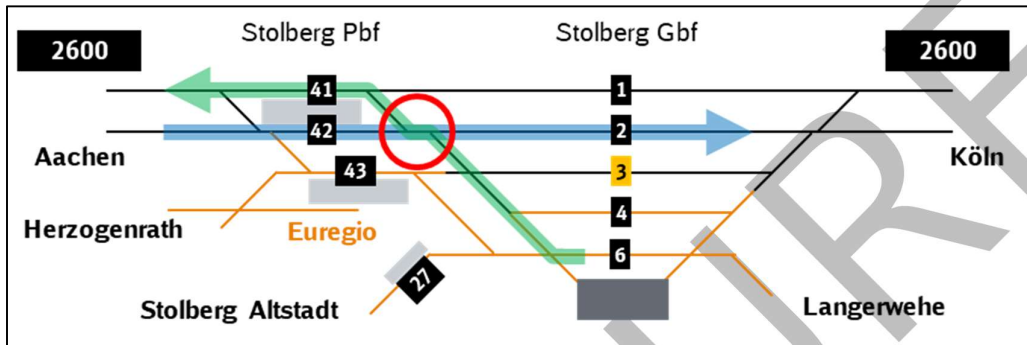
Abbildung 17: Gleisplan von Stolberg Hbf und niveaugleich einfädelnde RB 20
