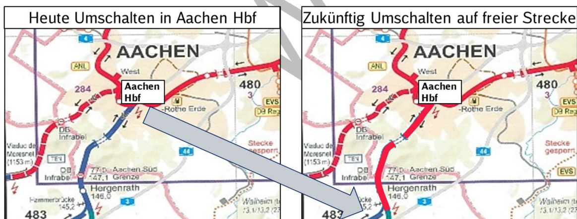
Abbildung 21: Verlegung der Systemtrennstelle von Aachen Hbf auf die Strecke Richtung Liège
