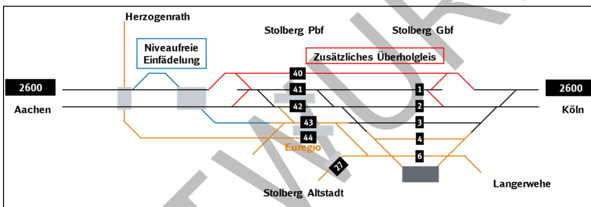
Abbildung 32: Zusätzliches Überholungsgleis und niveaufreie Einfädung für die RB 20 in Stolberg Hbf
