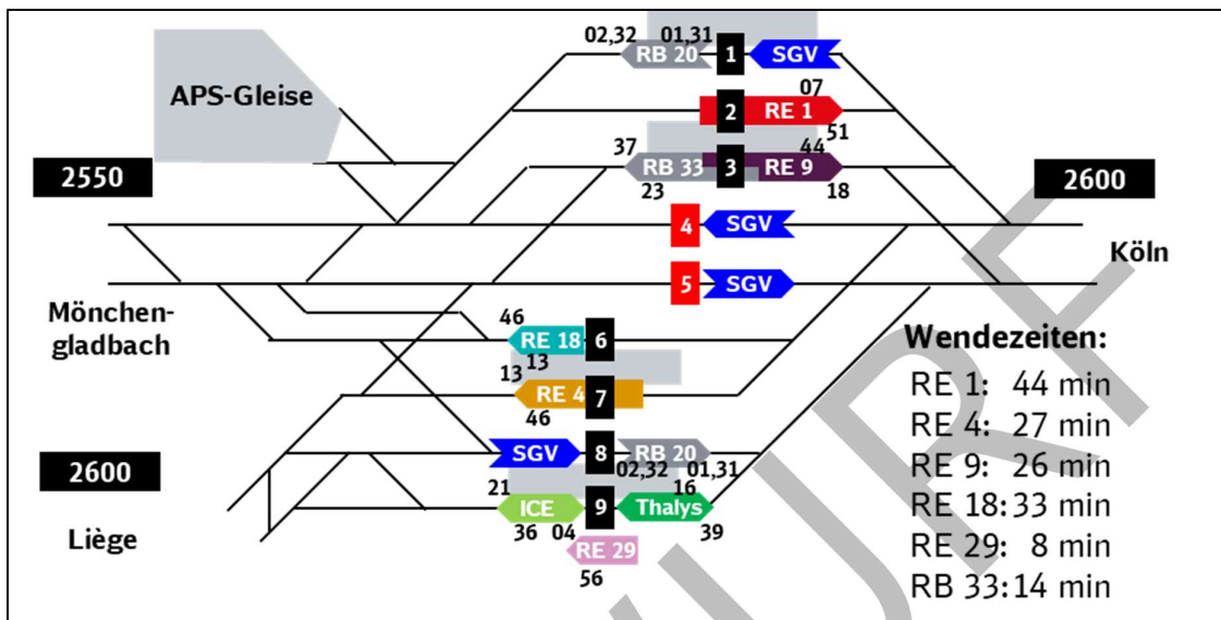
Abbildung 13: exemplarische Gleisbelegung in Aachen Hbf (vormittags)
