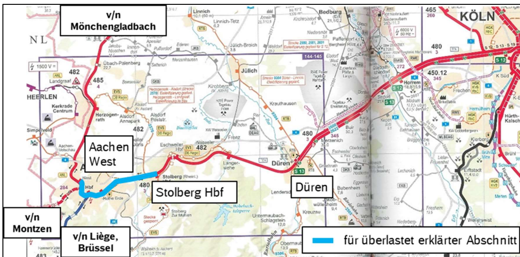
Abbildung 2: Lage des als überlastet erklärten Schienenweges im Streckennetz
