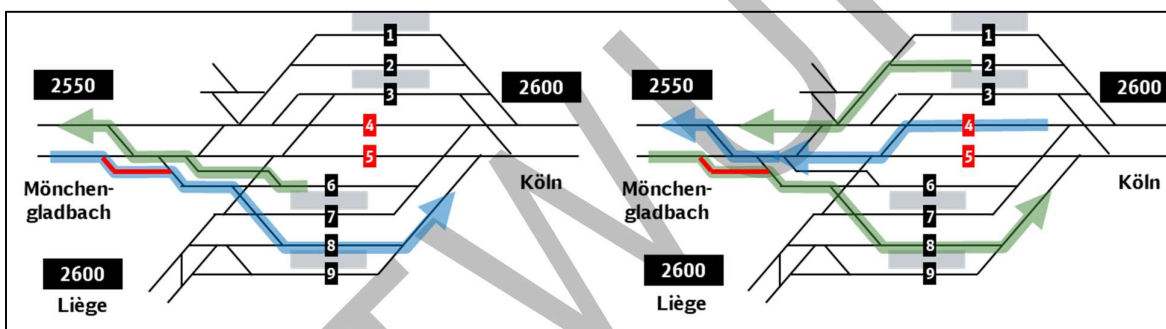
Abbildung 22: Zusätzliche Weichen ermöglichen parallele Fahrmöglichkeiten zwischen den Gleisen 6 und 7 bzw. 8
