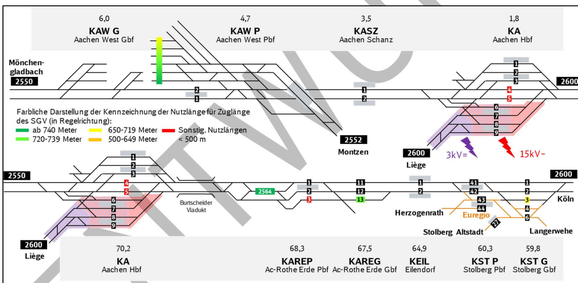
Abbildung 3: Infrastrukturübersicht des Abschnittes Stolberg Hbf - Aachen West
