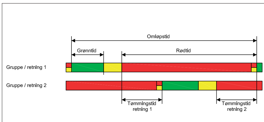
Figur 3-4: Omløpstid, grønntid og rødtid og tømmingstid i skyttelsignalanlegg.
