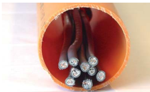
Figur 2-57: 9 detektorkabler (PFSP 2 \times 2,5 \text{ mm}^2 ) i 110 mm rør.
