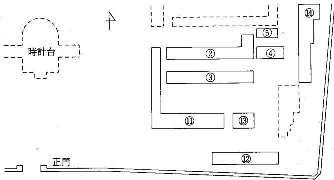
図9-5 機械系建物配置図(平成6年)
