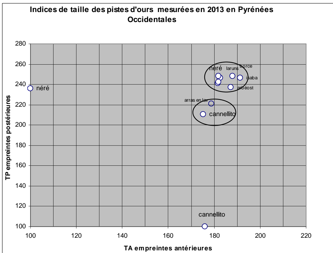
Graph 7. Indices de taille calculés à partir des mesures des empreintes d'ours récoltés dans les Pyrénées Occidentales en 2013.
