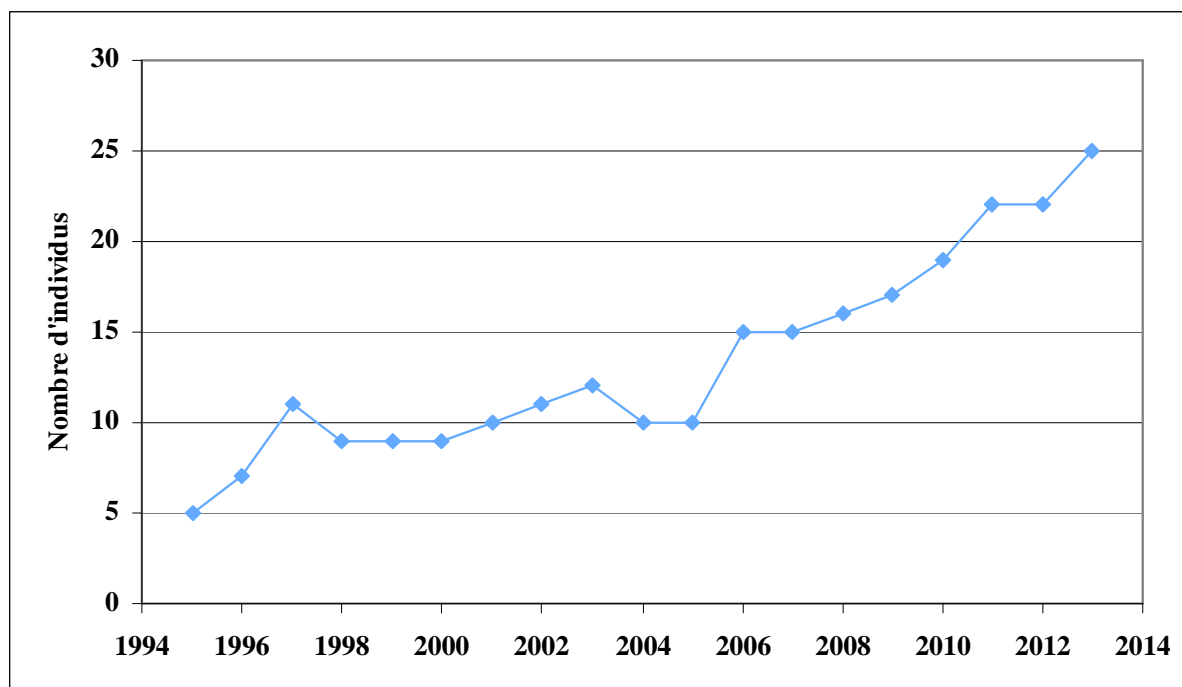
Graphique n° 8. Evolution des effectifs minimums détectés dans les Pyrénées depuis 1995.
