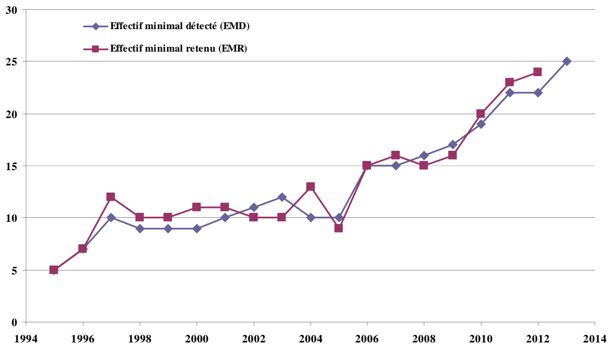
Graph n° 10 : Courbes des effectifs minimums détectés et des effectifs minimums retenus.
