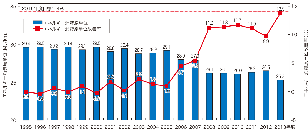
エネルギー消費原単位とエネルギー消費原単位改善率の推移
