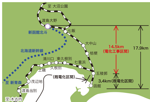
電化工事区間概要図
