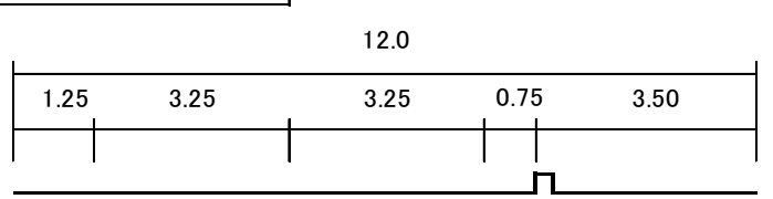
標準断面図
