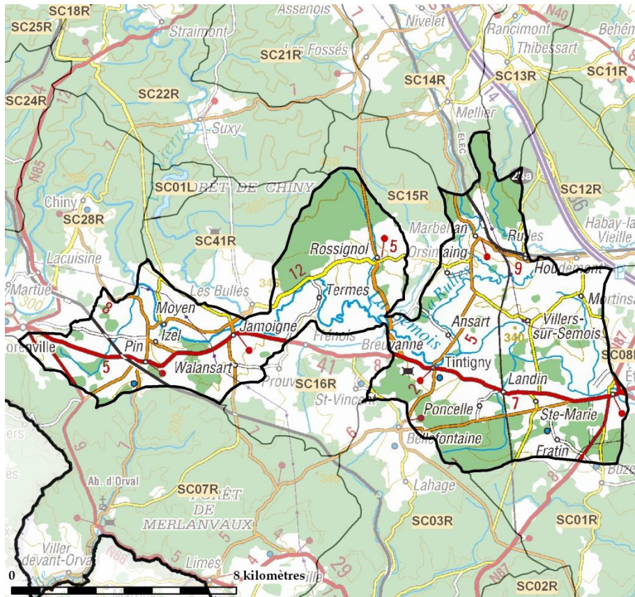
Bassin versant de la masse d'eau de surface (2009) SC23R
