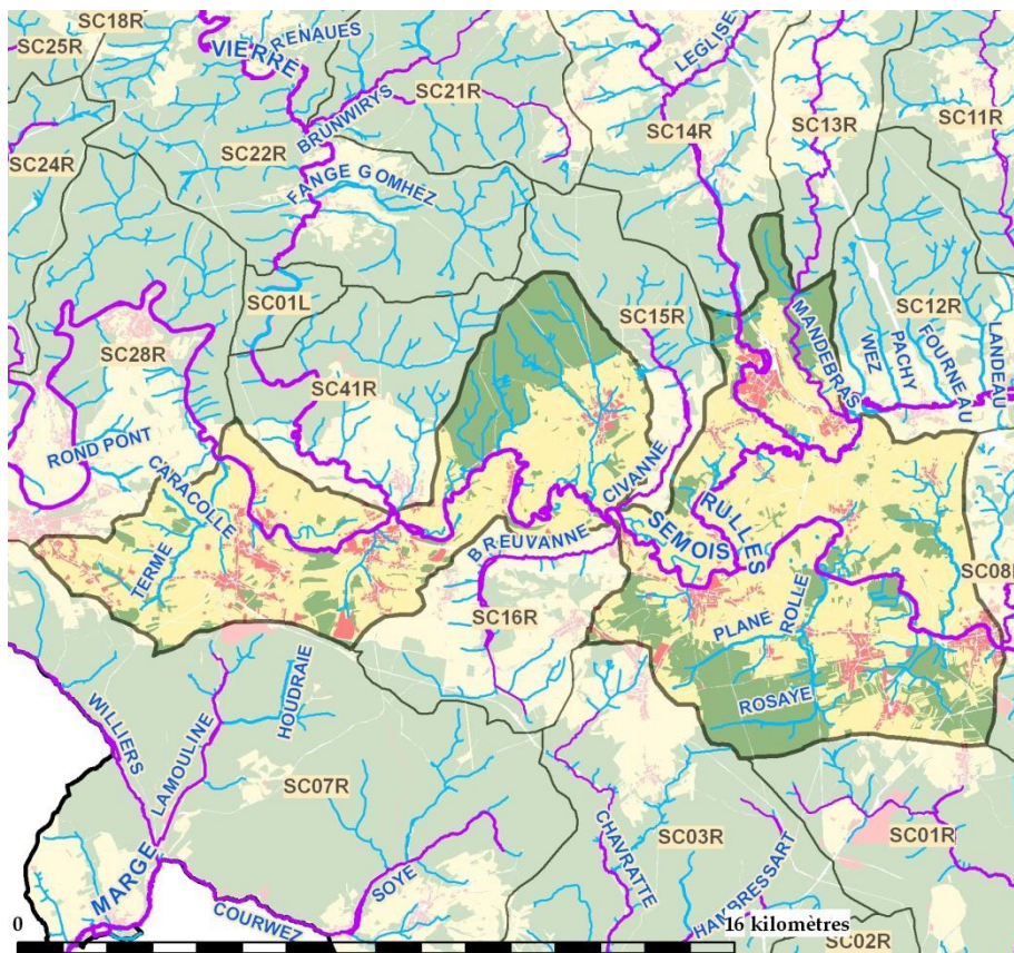
Masses d'eau de surface et principaux cours d'eau (2009) SC23R
