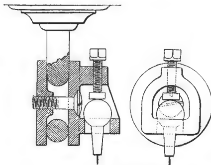
Рис. 2. Способъ прикрѣпленія нити маятника.
