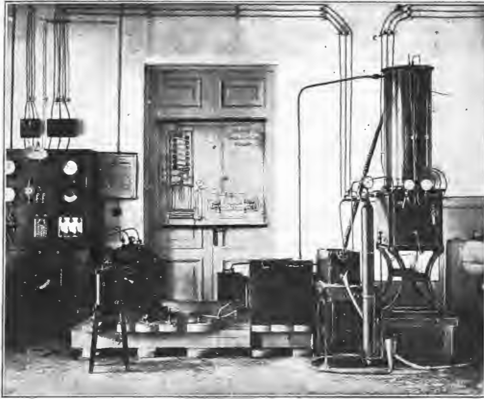
Палата мѣръ и вѣсовъ въ Петербургѣ. Приборъ проф. Линде для превращенія атмосфернаго воздуха въ жидкость. По фот. К. Булла авт. «Нивы».
