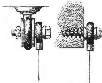
Рис. 1. Прикрѣпленіе маятника къ потолку или балкѣ.
