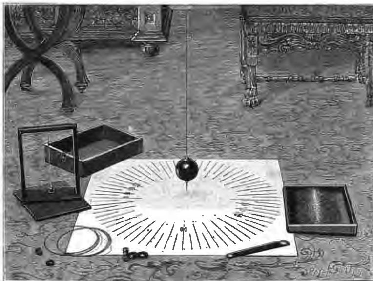
Рис. 3. Аппаратъ, наглядно показывающій вращательное движеніе земли.
