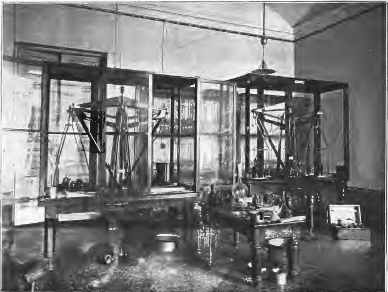
Палата мѣръ и вѣсовъ въ Петербургѣ. Отдѣленіе съ чувствительными вѣсами для точнаго взвѣшиванія. По фот. К. Булла авт. «Нивы».
