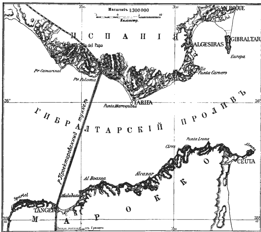
Проект туннеля под Гибралтарским проливом.
