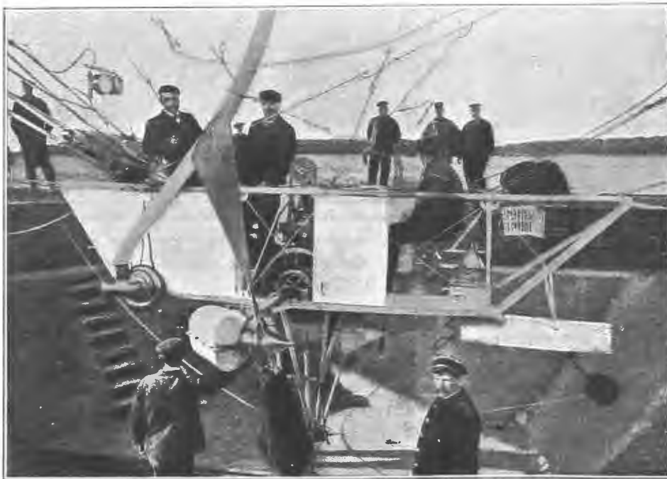
„Воздушный корабль“ Лебоди. Гондола воздушнаго корабля.
