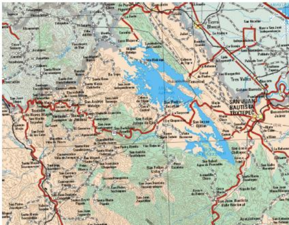
FIGURA 1.1. Esquema del sistema de presas Temascal-Cerro de Oro (De Luna 2010, p. 49).
