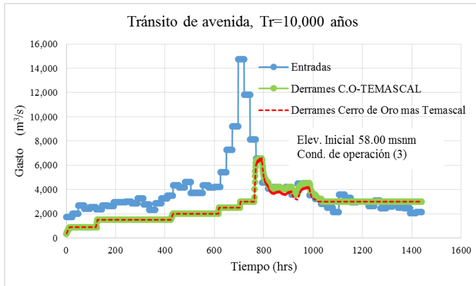
FIGURA 5.7. Tránsito de avenidas, Tr = 10,000 años, elevación inicia 58.00 msnm y condición de operación 3
