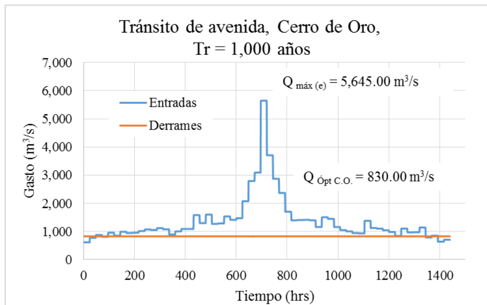
FIGURA 5.44. Tránsito de avenidas en Cerro de Oro, Tr = 1,000 años y política óptima
