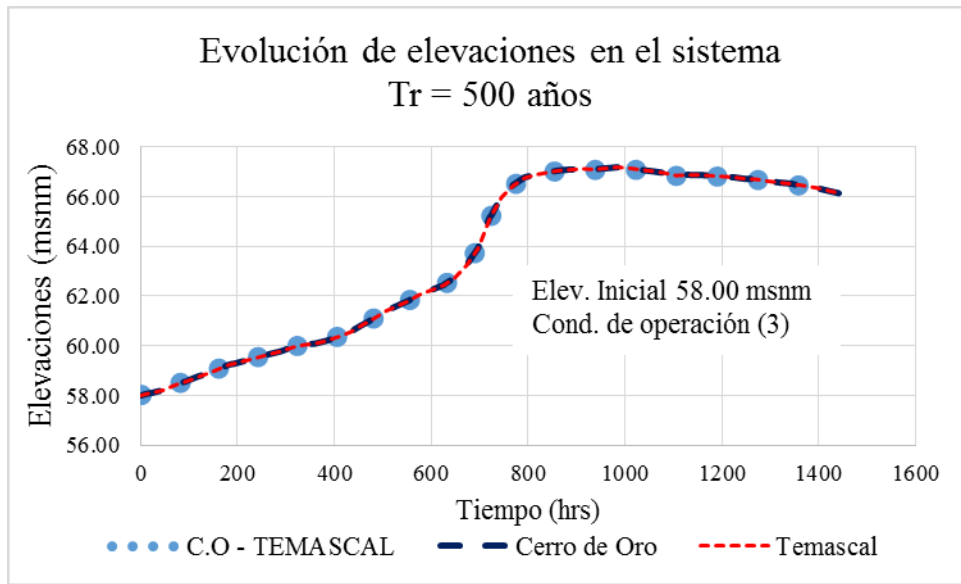
FIGURA 5.15. Evolución de elevaciones, Tr = 500 años, elevación inicia 58.00 msnm y condición de operación 3
