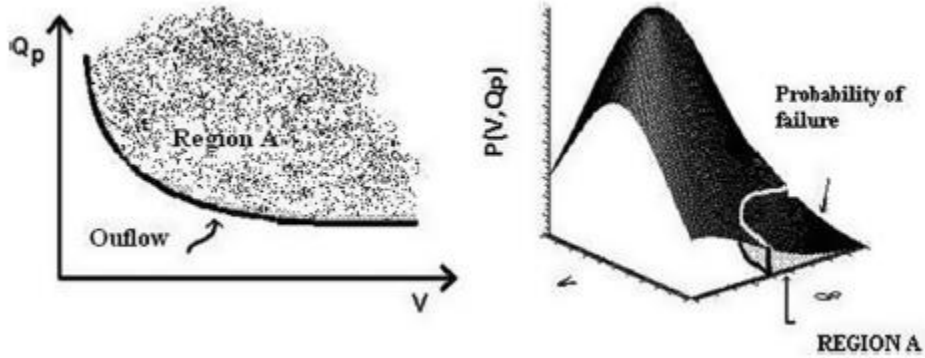
FIGURA 2.3. Definición de la zona de falla para un gasto máximo de descarga
