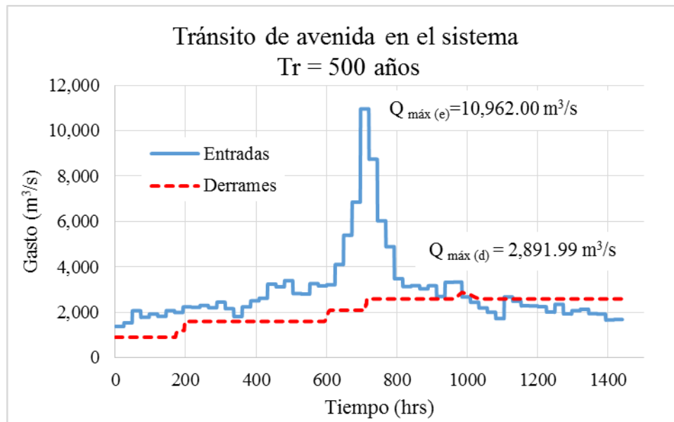
FIGURA 5.33. Tránsito de avenidas en sistemas de embalses, Tr = 500 años y política de operación en Cerro de Oro y Temascal
