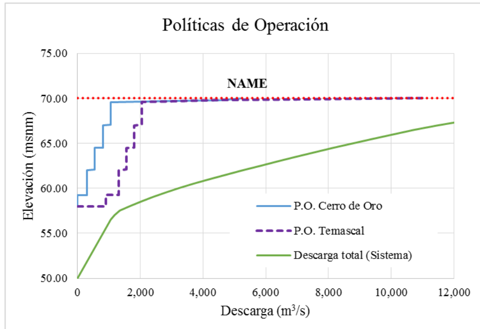
FIGURA 5.29. Políticas de operación, Cerro de Oro y Temascal
