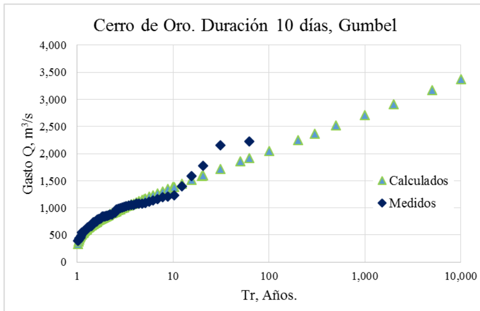
FIGURA 4.3. Ajuste de la serie de gastos con duración de 10 días, Cerro de Oro
