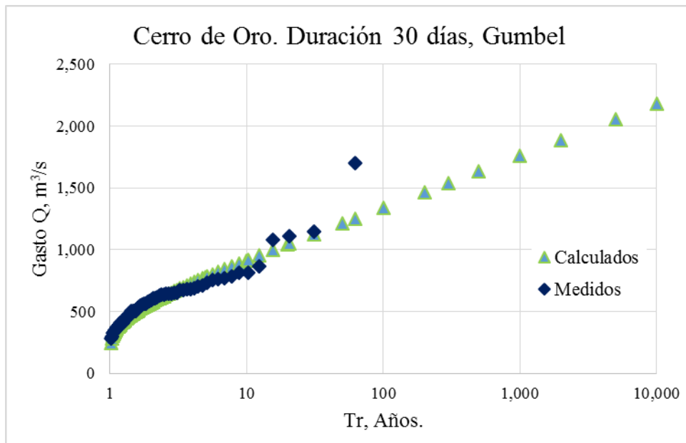
FIGURA 4.5. Ajuste de la serie de gastos con duración de 30 días, Cerro de Oro
