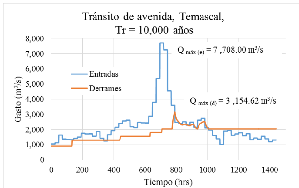
FIGURA 5.32. Tránsito de avenidas en Temascal, Tr = 10,000 años y política de operación en Cerro de Oro y Temascal
