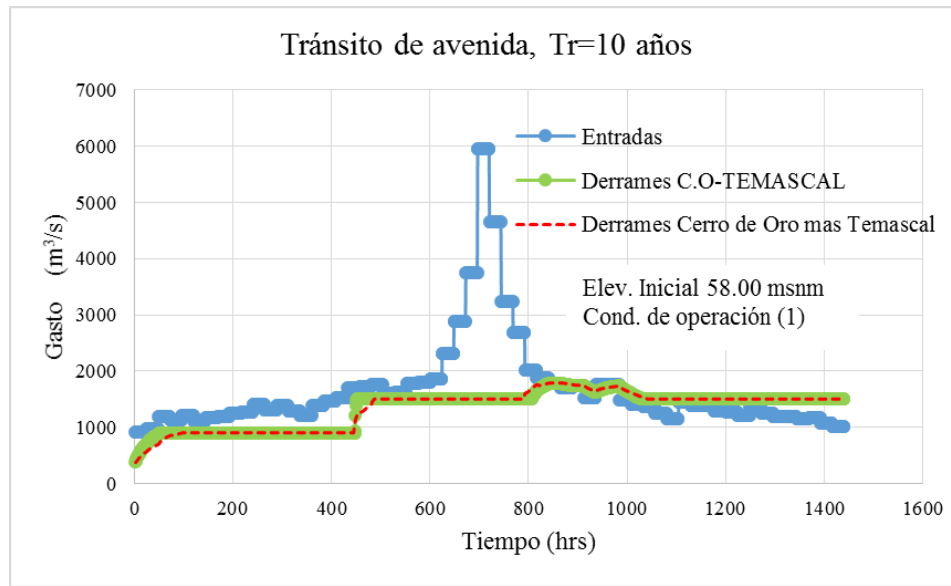
FIGURA 5.21. Tránsito de avenidas, Tr = 10 años, elevación inicia 58.00 msnm y condición de operación 1
