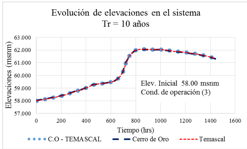
FIGURA 5.24. Evolución de elevaciones, Tr = 10 años, elevación inicial 58.00 msnm y condición de operación 3
