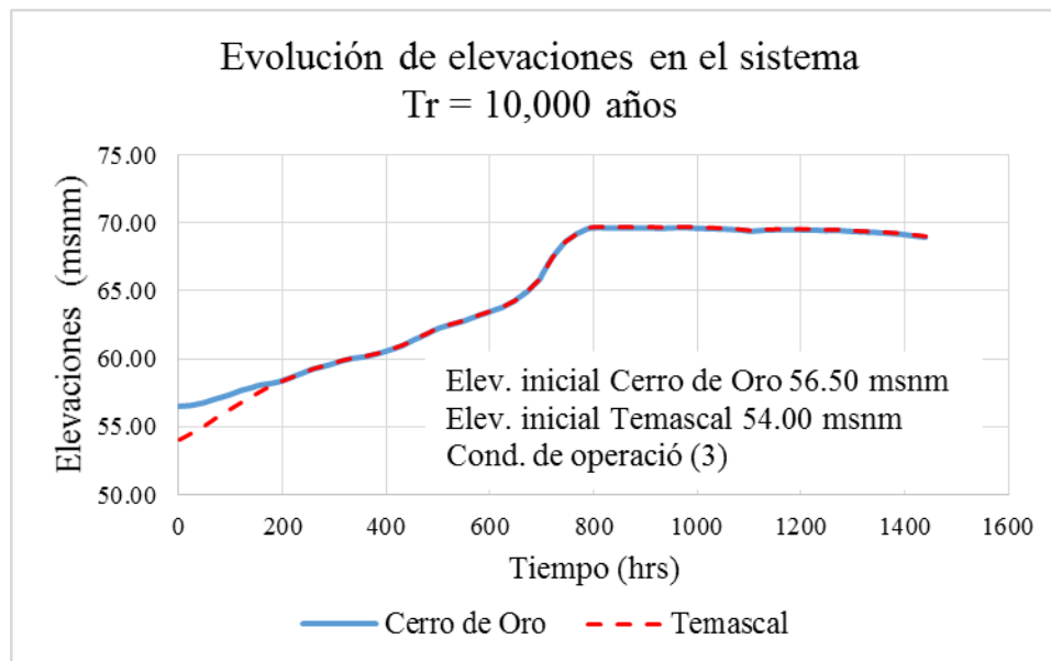
FIGURA 5.10. Evolución de elevaciones, Tr = 10,000 años, elevaciones iniciales, Cerro de Oro 56.50 msnm y Temascal 54.00 msnm, y condición de operación 3
