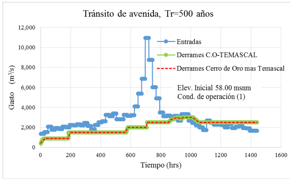
FIGURA 5.12. Tránsito de avenidas, Tr = 500 años, elevación inicia 58.00 msnm y condición de operación 1
