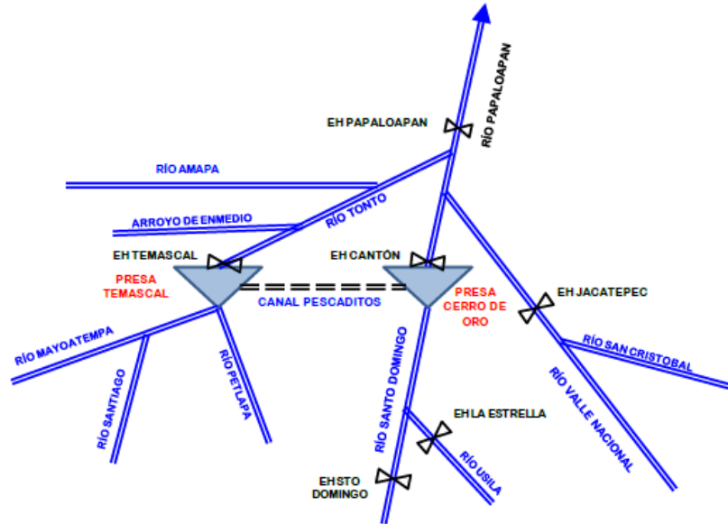
FIGURA 3.1. Esquema del sistema de presas Temascal-Cerro de Oro, De Luna (2010, p. 49)
