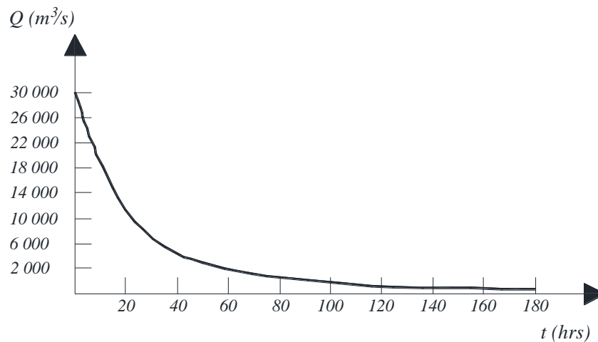
FIGURA 2.14. Curva tipo de descenso de avenidas
