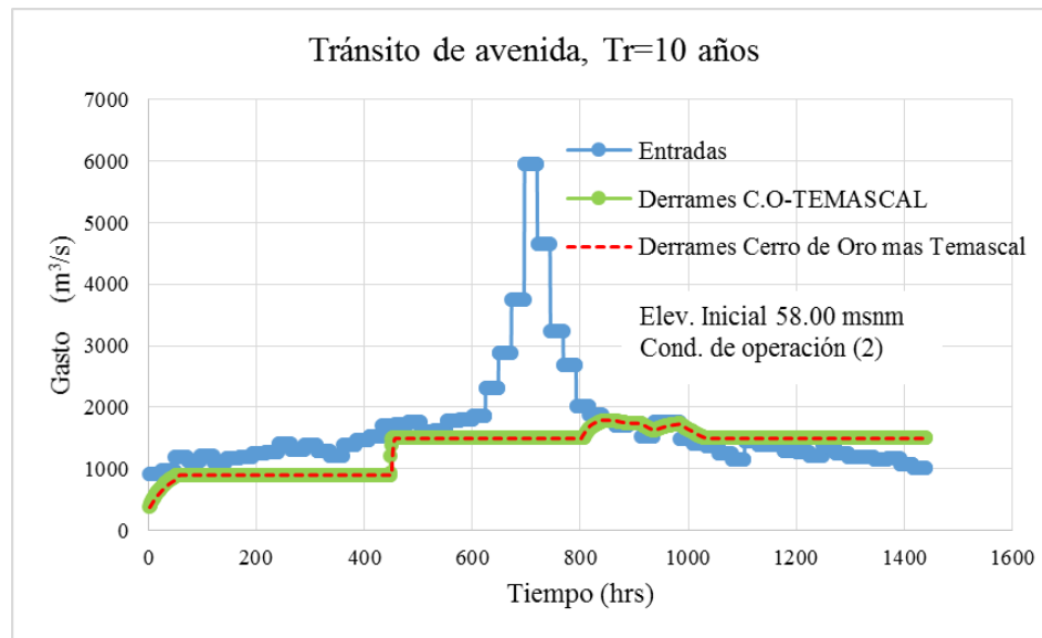
FIGURA 5.23. Tránsito de avenidas, Tr = 10 años, elevación inicia 58.00 msnm y condición de operación 2
