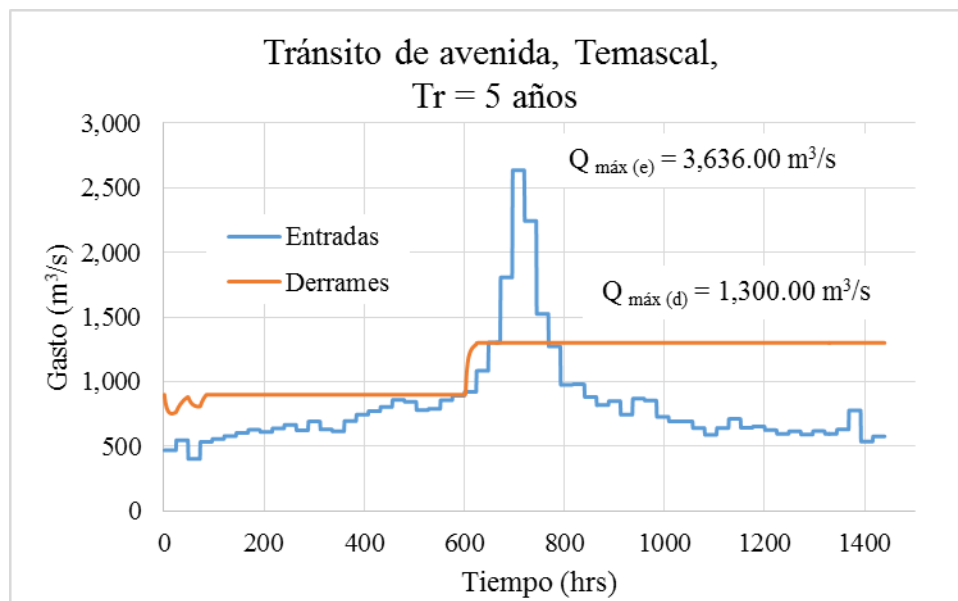
FIGURA 5.38. Tránsito de avenidas en Temascal, Tr = 5 años y política de operación en Cerro de Oro y Temascal
