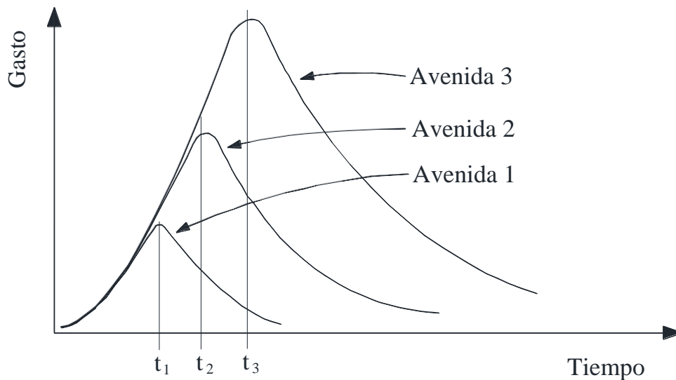
FIGURA 2.9. Hidrogramas para avenidas de periodos de retorno Tr_1, Tr_2 y Tr_3 .
