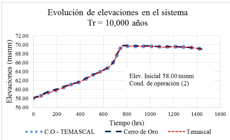
FIGURA 5.4. Evolución de elevaciones, Tr = 10,000 años, elevación inicia 58.00 msnm y condición de operación 2
