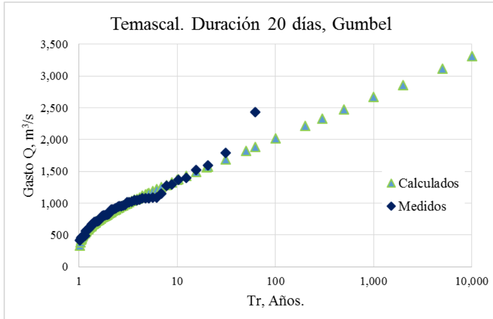
FIGURA 4.10. Ajuste de la serie de gastos con duración de 20 días, Temascal
