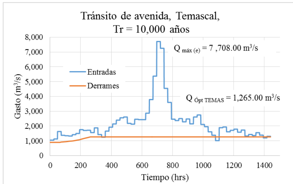
FIGURA 5.41. Tránsito de avenidas en Temascal, Tr = 10,000 años y política óptima
