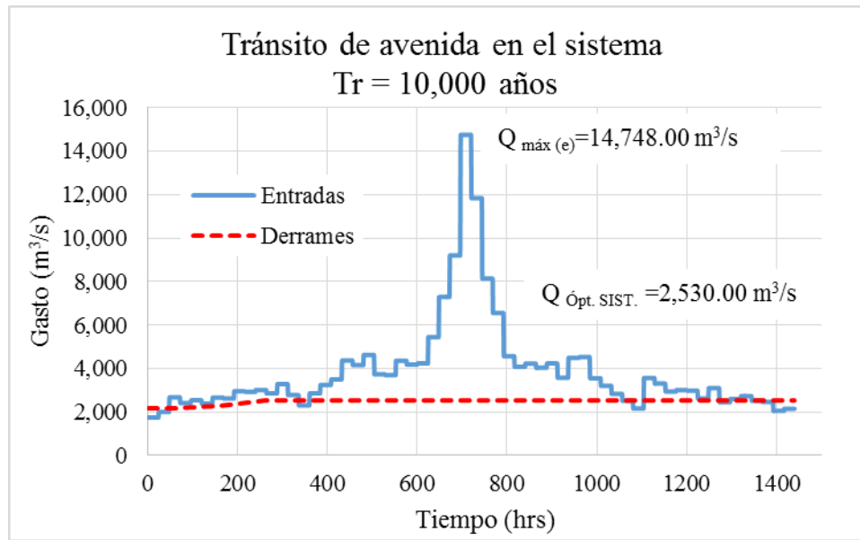
FIGURA 5.39. Tránsito de avenidas en el sistema, Tr = 10,000 años y política óptima
