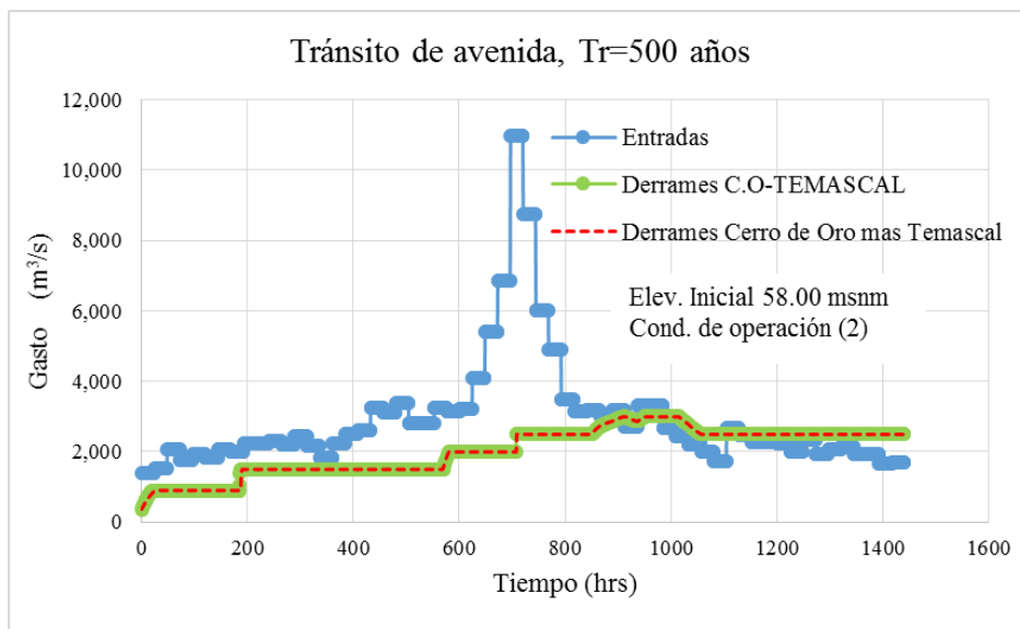
FIGURA 5.14. Tránsito de avenidas, Tr = 500 años, elevación inicia 58.00 msnm y condición de operación 2
