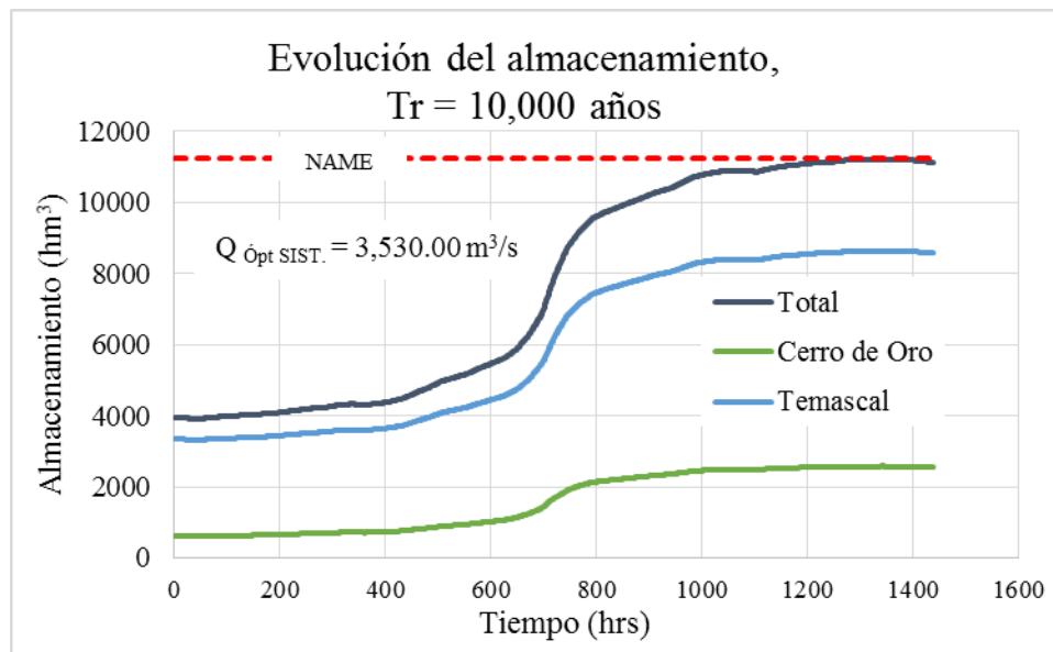
FIGURA 5.42. Evolución del almacenamiento, Tr = 10,000 años y política óptima
