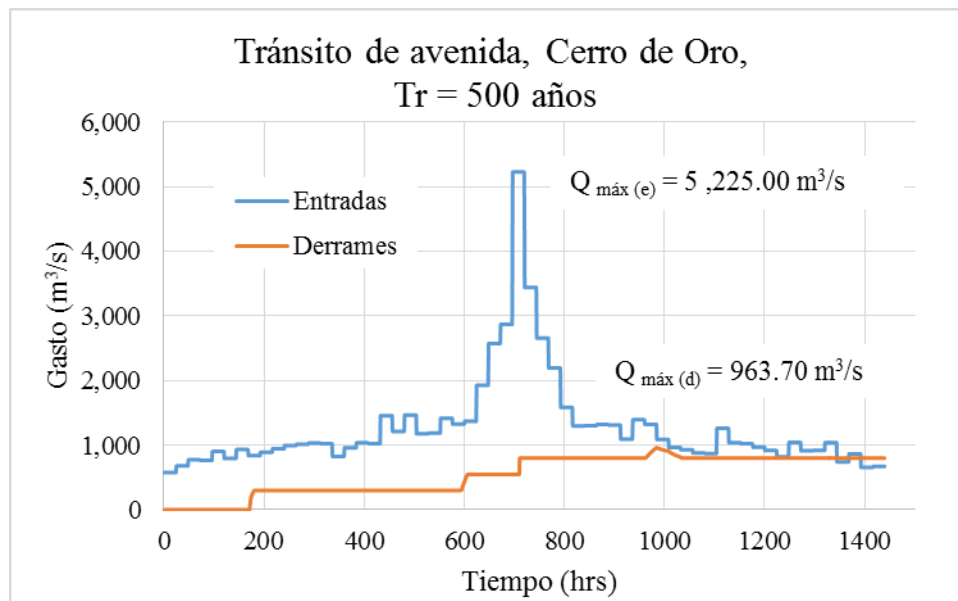
FIGURA 5.34. Tránsito de avenidas en Cerro de Oro, Tr = 500 años y política de operación en Cerro de Oro y Temascal
