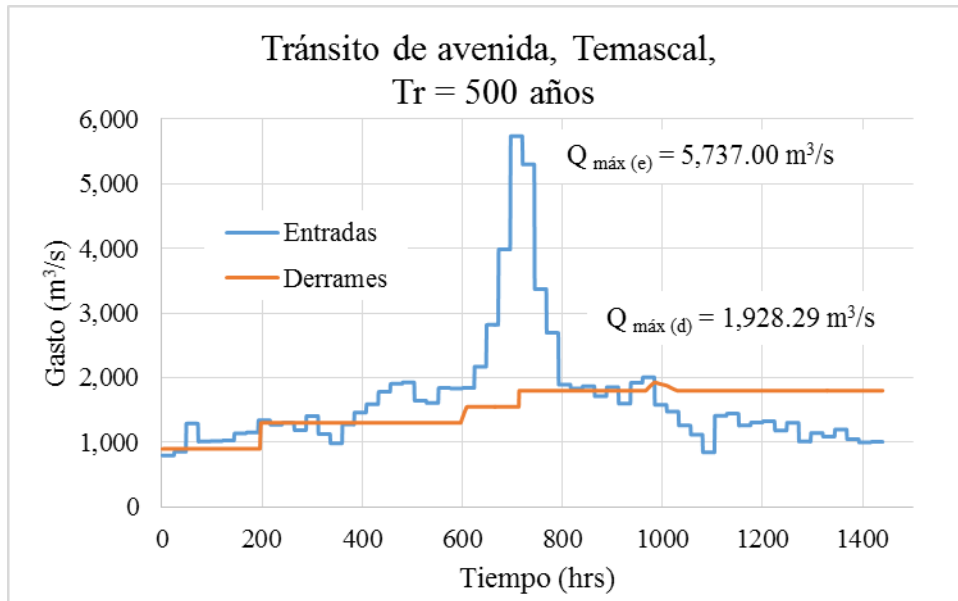
FIGURA 5.35. Tránsito de avenidas en Temascal, Tr = 500 años y política de operación en Cerro de Oro y Temascal
