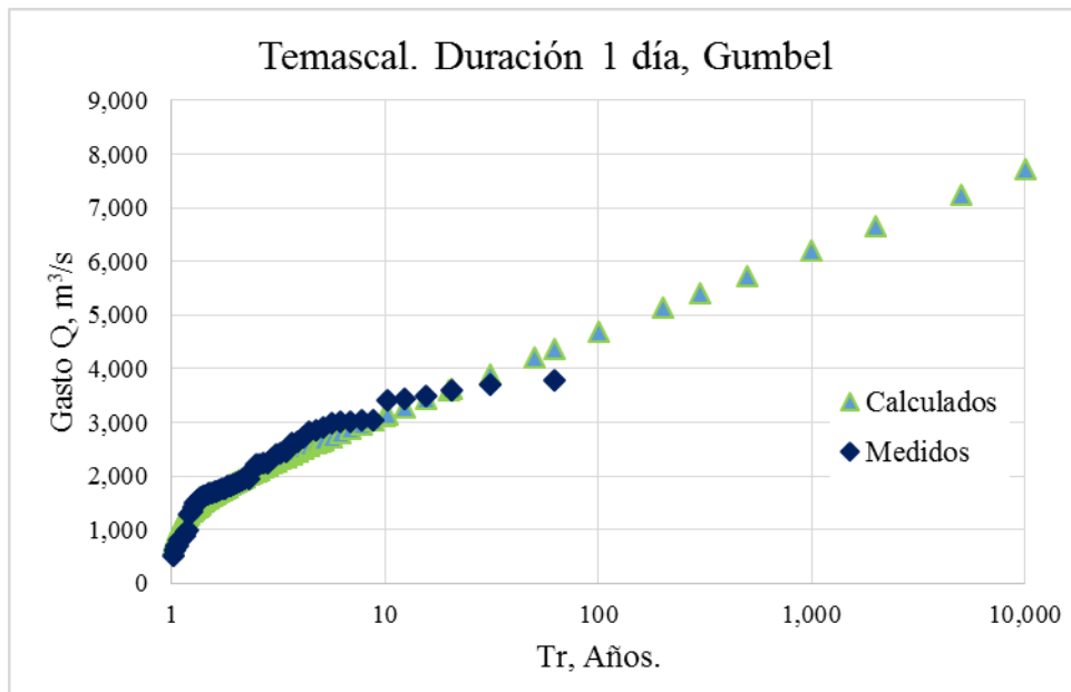
FIGURA 4.7. Ajuste de la serie de gastos con duración de 1 día, Temascal
