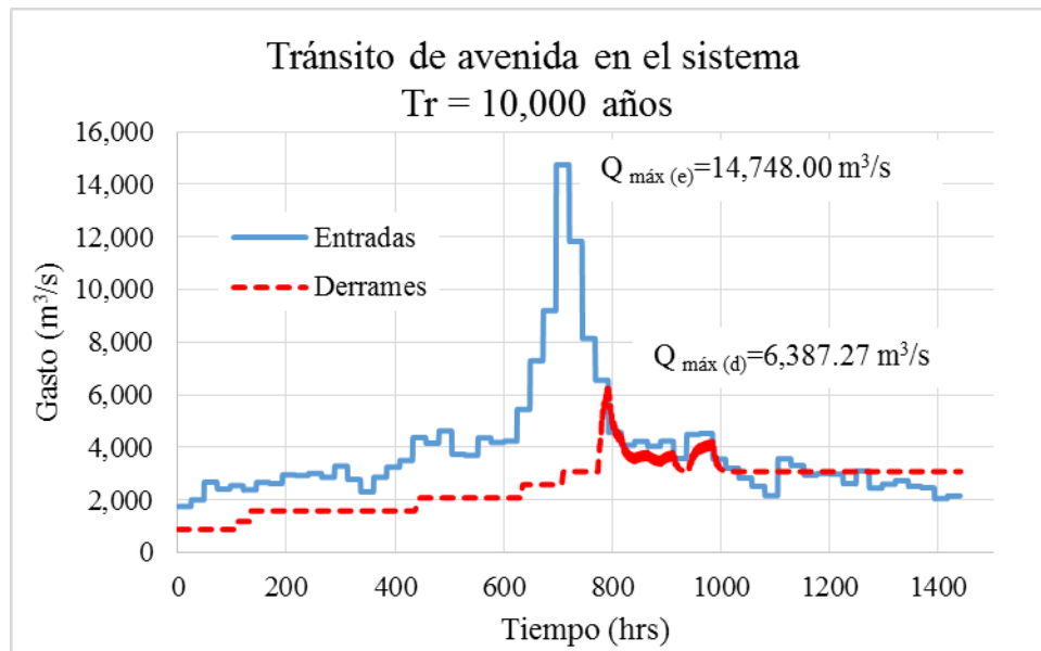
FIGURA 5.30. Tránsito de avenidas en el sistema de embalses, Tr = 10,000 años y política de operación en Cerro de Oro y Temascal
