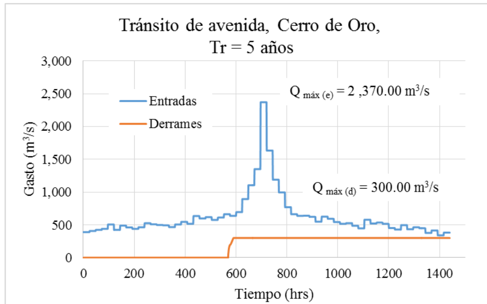
FIGURA 5.37. Tránsito de avenidas en Cerro de Oro, Tr = 5 años y política de operación en Cerro de Oro y Temascal
