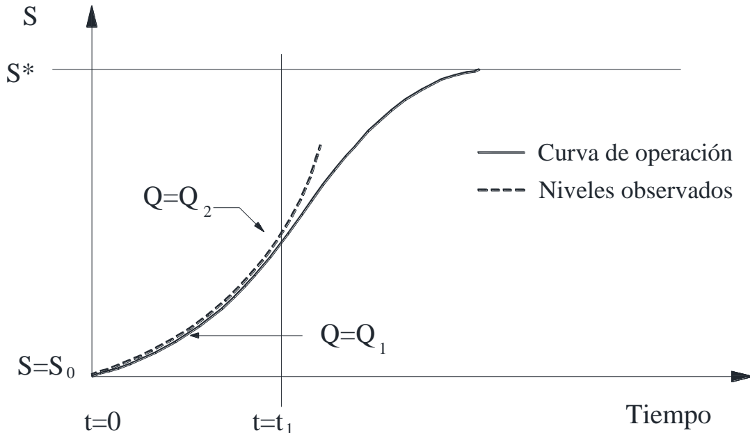
FIGURA 2.10. Operación de acuerdo con la política obtenida para la avenida con periodo de retorno Tr .
