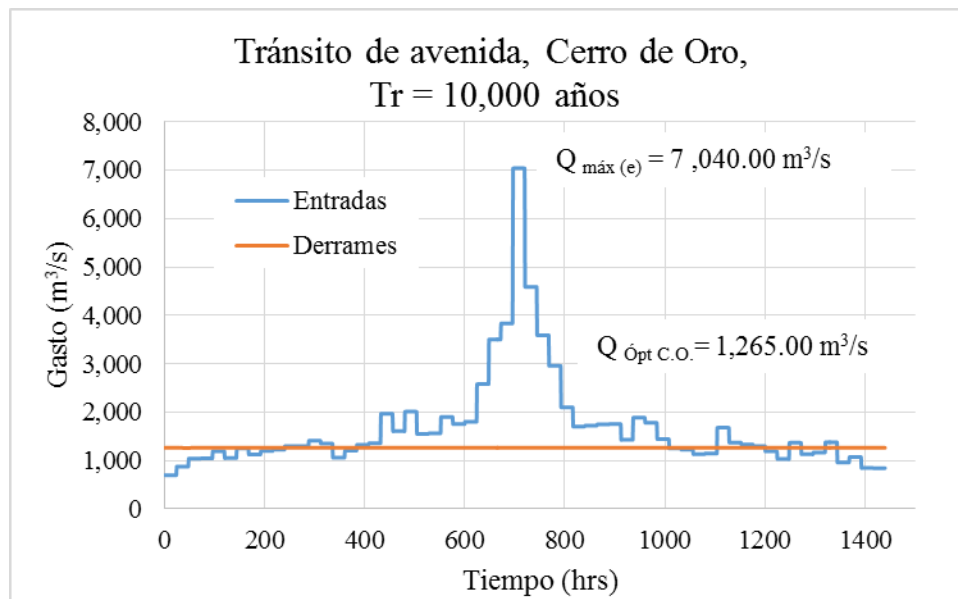
FIGURA 5.40. Tránsito de avenidas en Cerro de Oro, Tr = 10,000 años y política óptima
