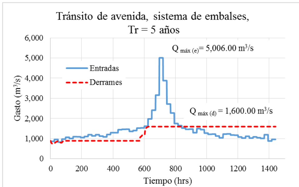
FIGURA 5.36. Tránsito de avenidas en el sistema de embalses, Tr = 5 años y política de operación en Cerro de Oro y Temascal
