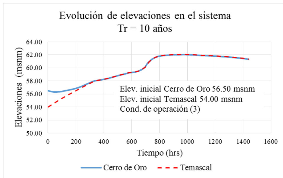
FIGURA 5.28. Evolución de elevaciones, Tr = 10 años, elevaciones iniciales, Cerro de Oro 56.50 msnm y Temascal 54.00 msnm, y condición de operación 3
