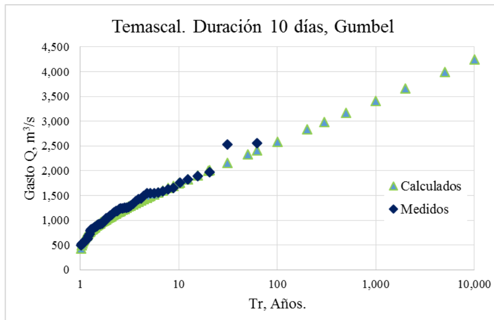
FIGURA 4.9. Ajuste de la serie de gastos con duración de 10 días, Temascal
