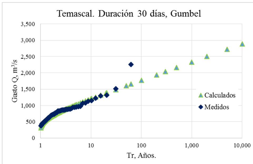
FIGURA 4.11. Ajuste de la serie de gastos con duración de 30 días, Temascal
