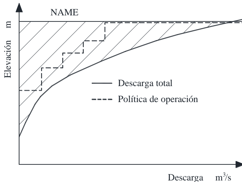
FIGURA 2.15. Nomograma de la política de operación
