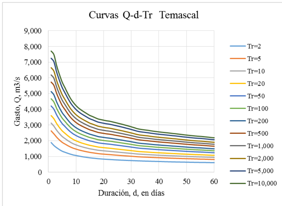
FIGURA 4.14. Curvas gasto duración periodo de retorno, Temascal
