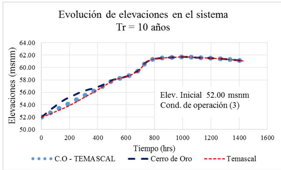
FIGURA 5.26. Evolución de elevaciones, Tr = 10 años, elevación inicial 52.00 msnm y condición de operación 3
