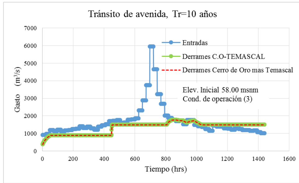
FIGURA 5.25. Tránsito de avenidas, Tr = 10 años, elevación inicial 58.00 msnm y condición de operación 3
