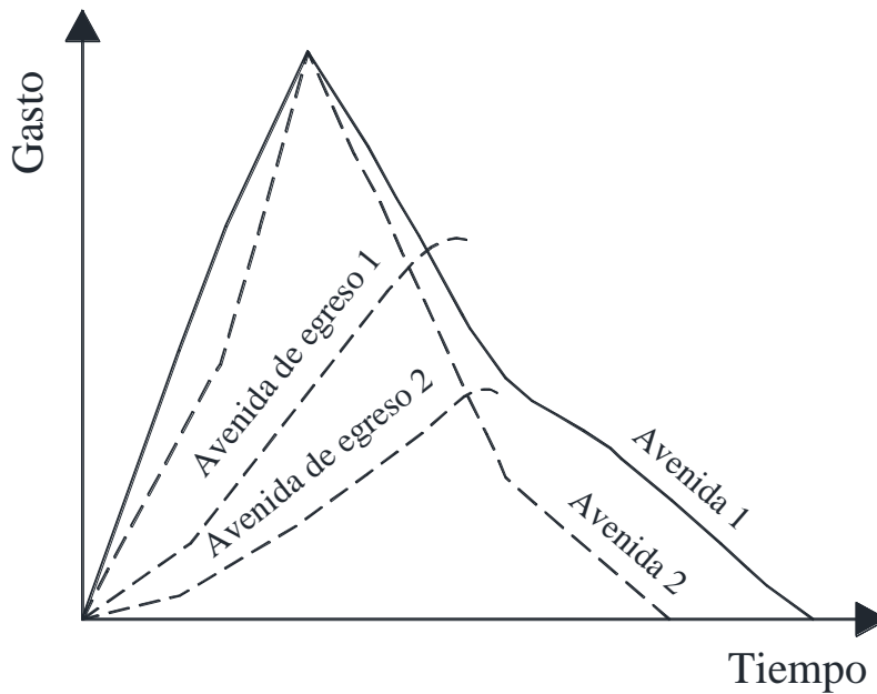
FIGURA 2.1. Tránsito de avenidas con mismo gasto pico, pero diferente volumen
