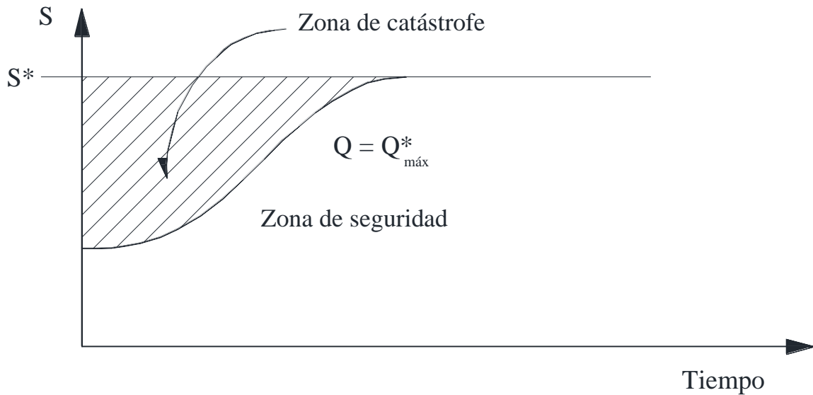
FIGURA 2.11. Política de operación para la avenida de diseño
