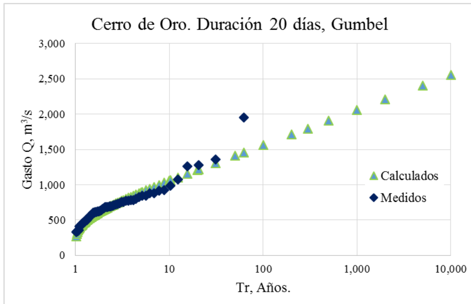
FIGURA 4.4. Ajuste de la serie de gastos con duración de 20 días, Cerro de Oro
