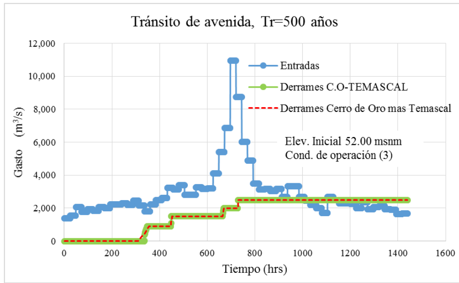
FIGURA 5.18. Tránsito de avenidas, Tr = 500 años, elevación inicia 52.00 msnm y condición de operación 3
