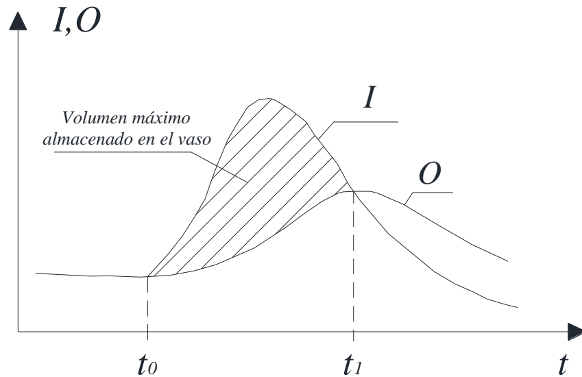
FIGURA 2.4. Hidrograma de entrada ( I ) y salida ( O )
