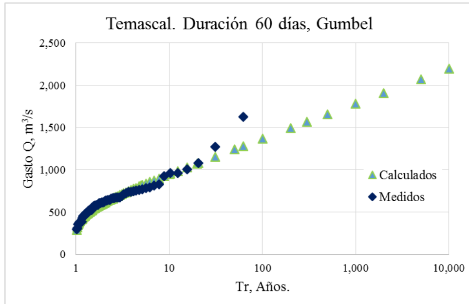
FIGURA 4.12. Ajuste de la serie de gastos con duración de 60 días, Temascal
