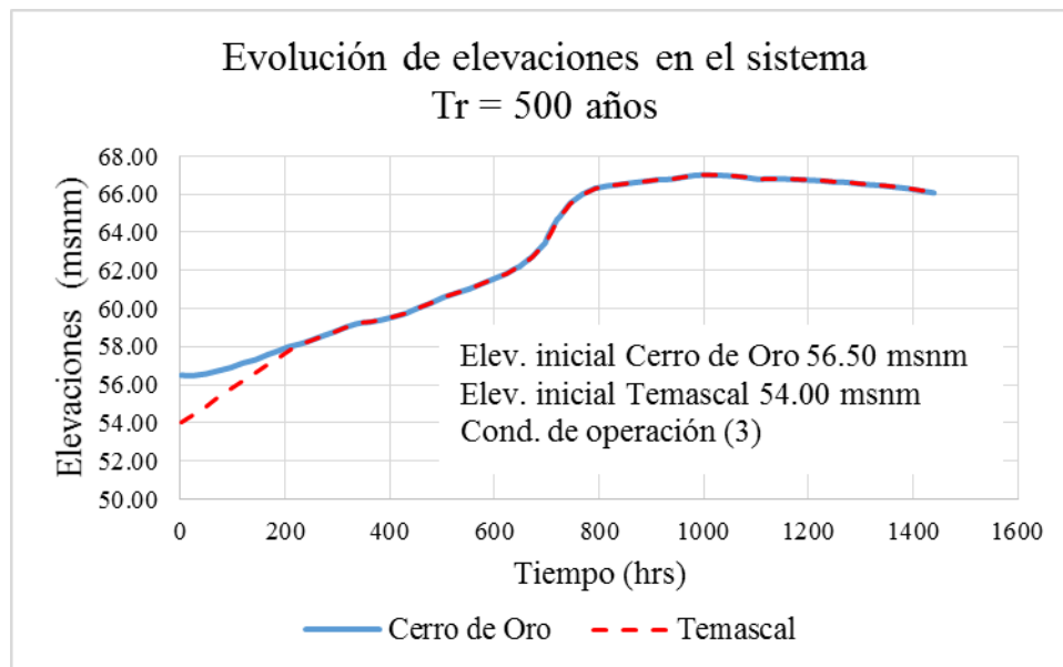
FIGURA 5.19. Evolución de elevaciones, Tr = 500 años, elevaciones iniciales, cerro de Oro 56.50 msnm y Temascal 54.00 msnm, y condición de operación 3
