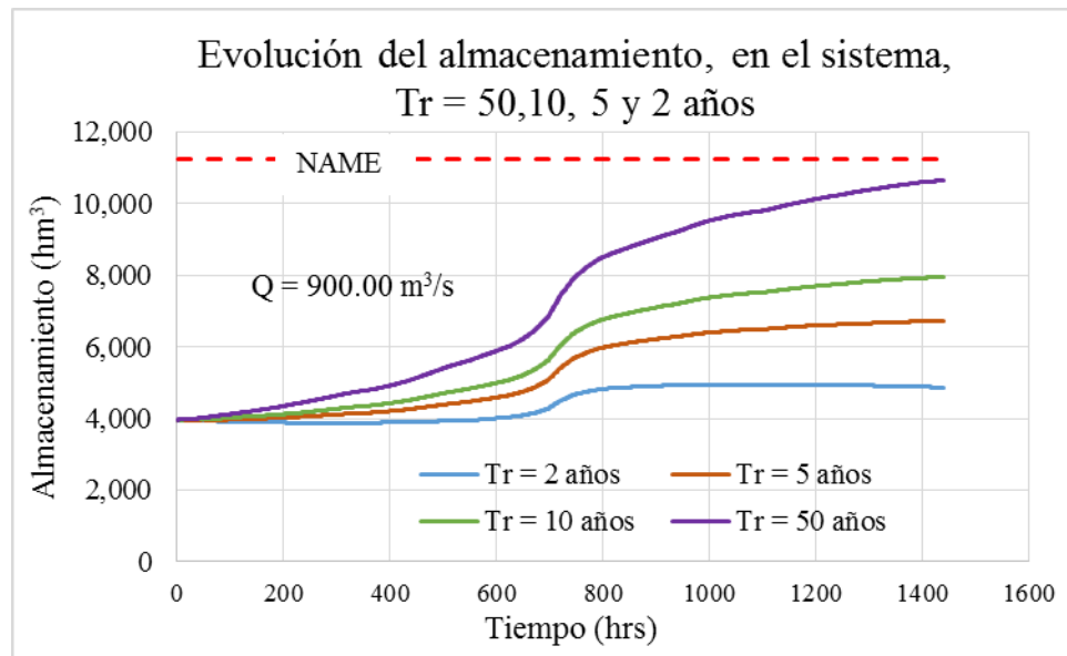
FIGURA 5.47. Evolución del almacenamiento, Tr = 50, 10, 5 y 2 años y gasto de operación
