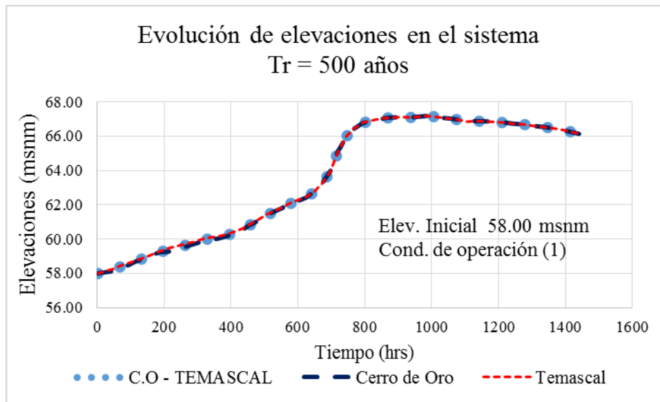
FIGURA 5.11. Evolución de elevaciones, Tr = 500 años, elevación inicial 58.00 msnm y condición de operación 1
