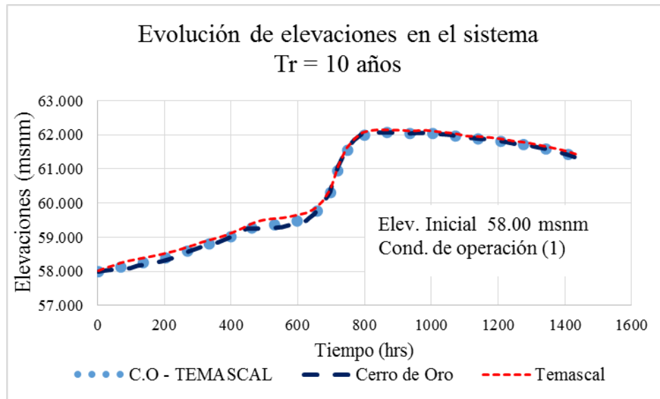
FIGURA 5.20. Evolución de elevaciones, Tr = 10 años, elevación inicia 58.00 msnm y condición de operación 1
