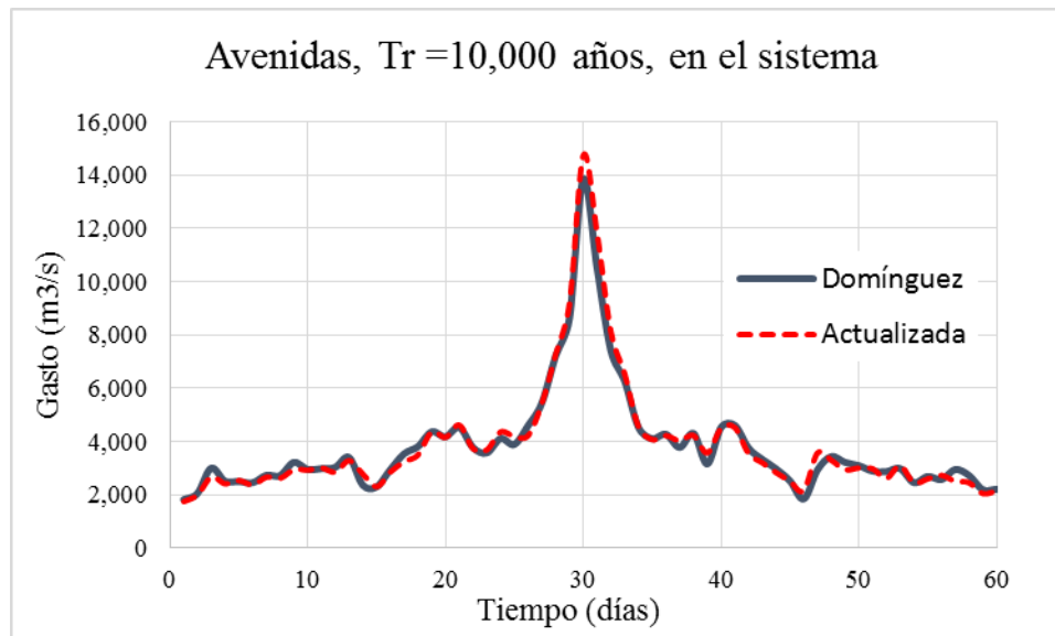
FIGURA 6.1. Avenida de diseño con Tr = 10,000 años, en el sistema, actualizada y obtenida por Domínguez.
