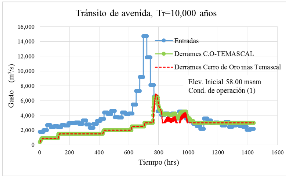
FIGURA 5.3. Tránsito de avenidas, Tr = 10,000 años, elevación inicia 58.00 msnm y condición de operación 1
