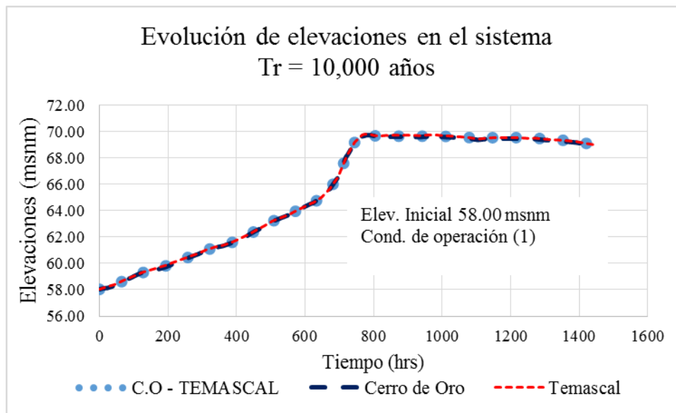
FIGURA 5.2. Evolución de elevaciones, Tr = 10,000 años, elevación inicial 58.00 msnm y condición de operación 1
