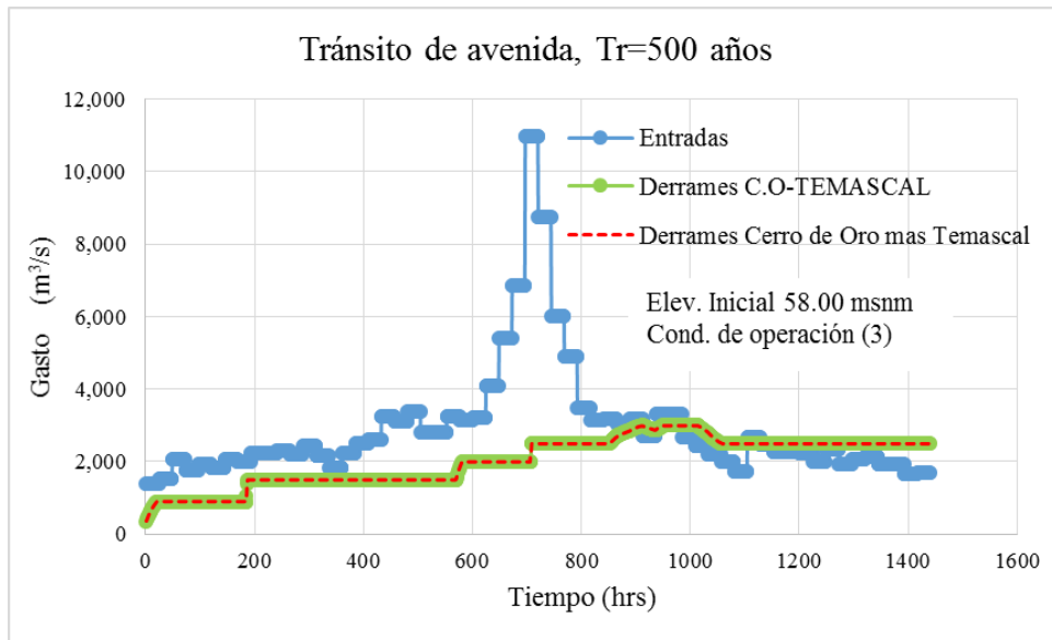
FIGURA 5.16. Tránsito de avenidas, Tr = 500 años, elevación inicia 58.00 msnm y condición de operación 3
