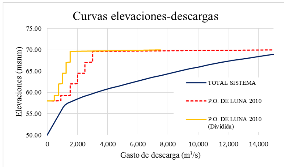
FIGURA 5.1. Política de operación escalonada (De Luna, 2010)
