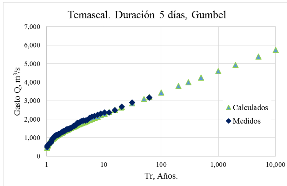
FIGURA 4.8. Ajuste de la serie de gastos con duración de 5 días, Temascal
