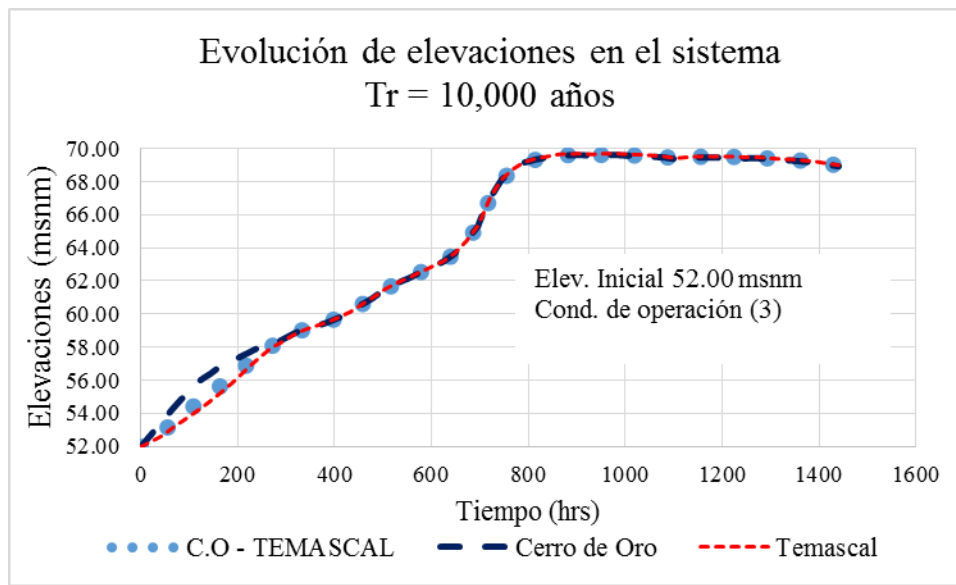
FIGURA 5.8. Evolución de elevaciones, Tr = 10,000 años, elevación inicial 52.00 msnm y condición de operación 3
