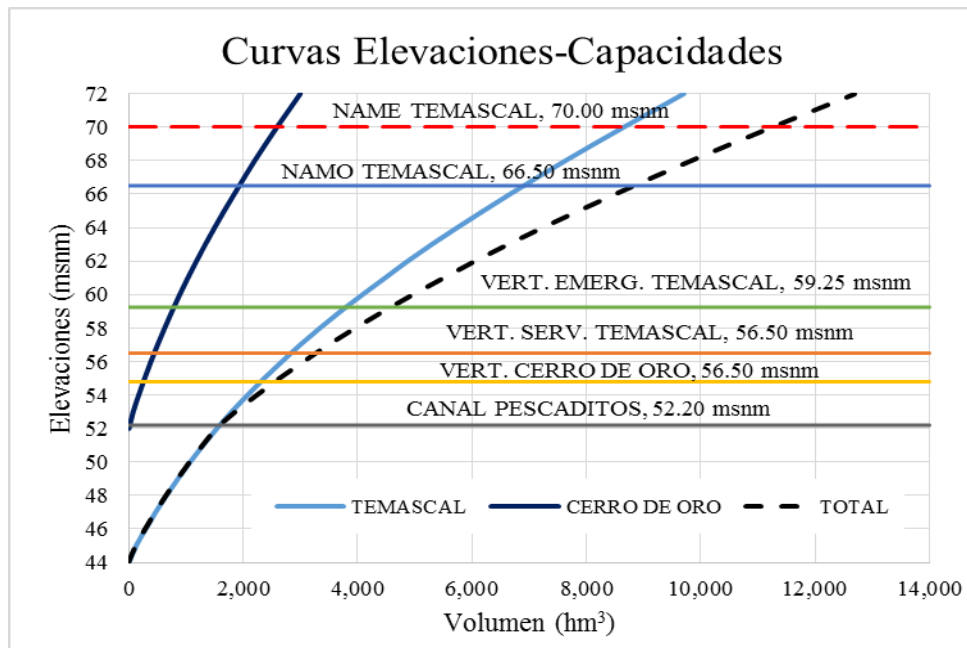
FIGURA 3.2. Curva Elevaciones-capacidades del sistema de presas, De Luna (2010)
