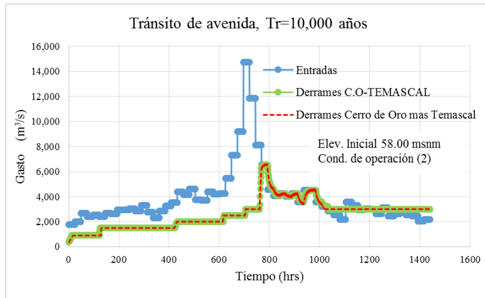
FIGURA 5.5. Tránsito de avenidas, Tr = 10,000 años, elevación inicia 58.00 msnm y condición de operación 2
