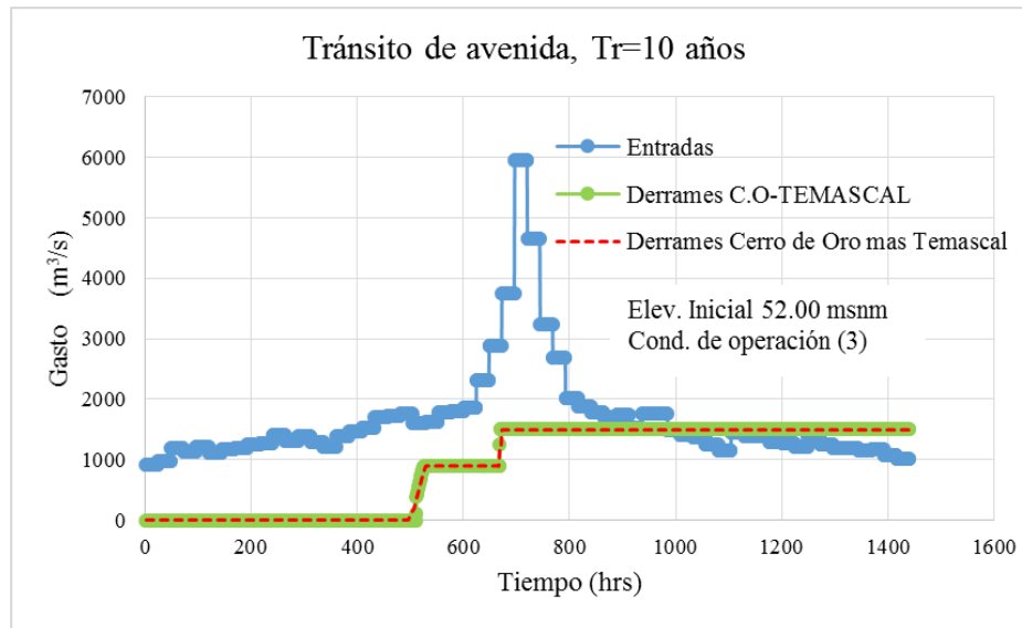
FIGURA 5.27. Tránsito de avenidas, Tr = 10 años, elevación inicia 52.00 msnm y condición de operación 3
