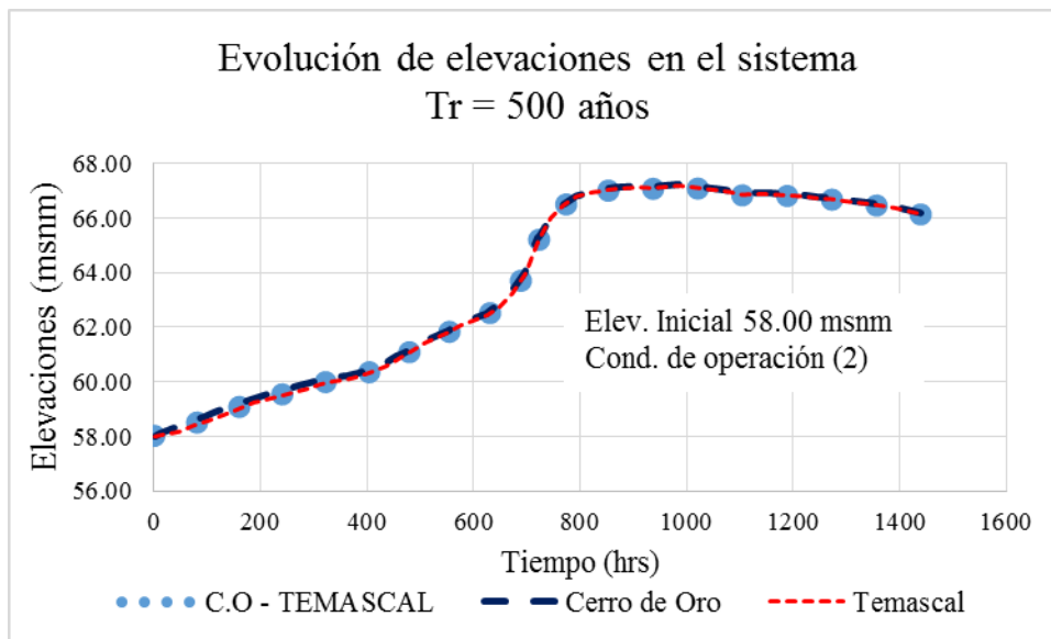
FIGURA 5.13. Evolución de elevaciones, Tr = 500 años, elevación inicia 58.00 msnm y condición de operación 2
