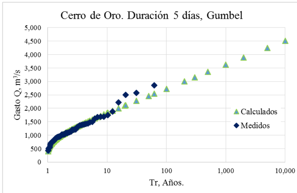
FIGURA 4.2. Ajuste de la serie de gastos con duración de 5 días, Cerro de Oro
