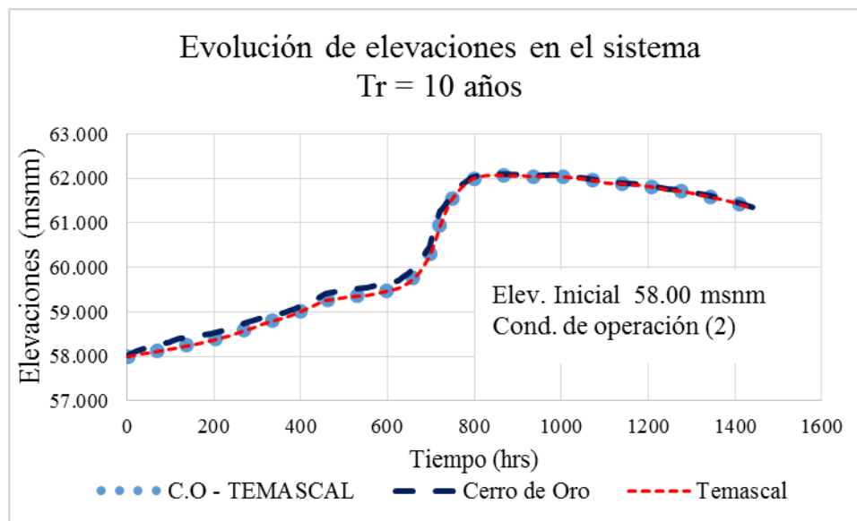
FIGURA 5.22. Evolución de elevaciones, Tr = 10 años, elevación inicia 58.00 msnm y condición de operación 2
