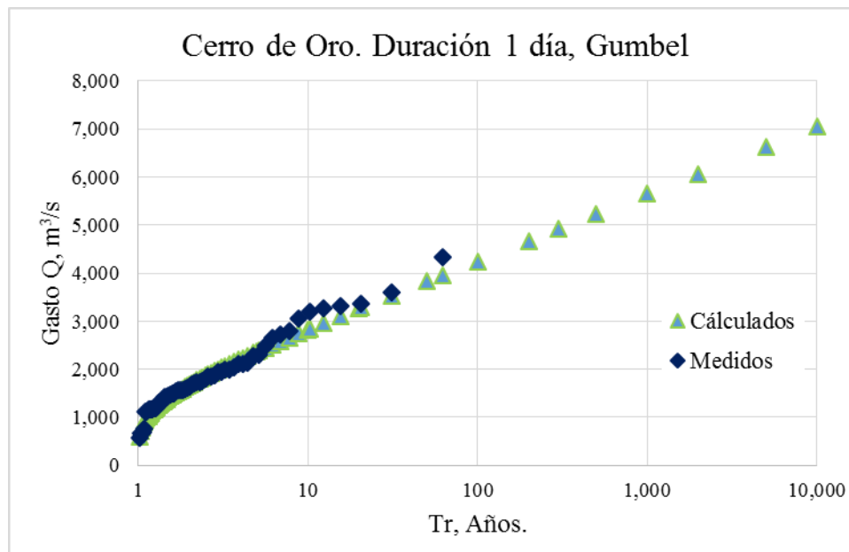
FIGURA 4.1. Ajuste de la serie de gastos con duración de 1 día, Cerro de Oro
