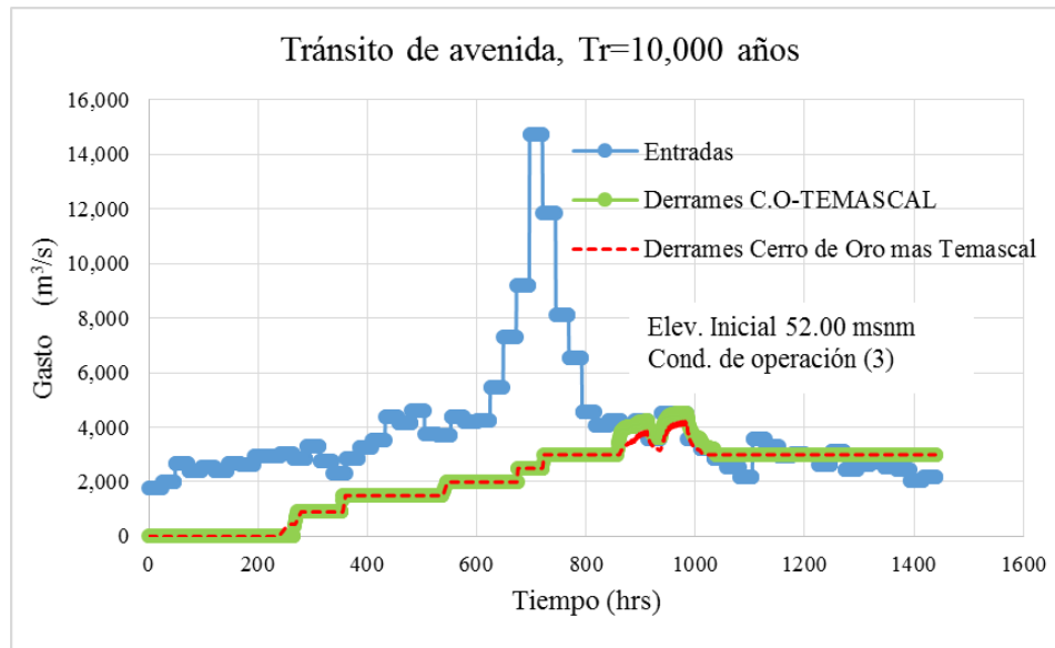
FIGURA 5.9. Tránsito de avenidas, Tr = 10,000 años, elevación inicia 52.00 msnm y condición de operación 3
