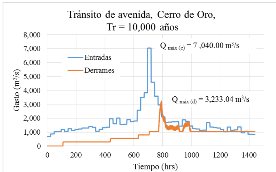
FIGURA 5.31. Tránsito de avenidas en Cerro de Oro, Tr = 10,000 años y política de operación en Cerro de Oro y Temascal
