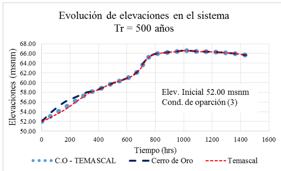
FIGURA 5.17. Evolución de elevaciones, Tr = 500 años, elevación inicial 52.00 msnm y condición de operación 3
