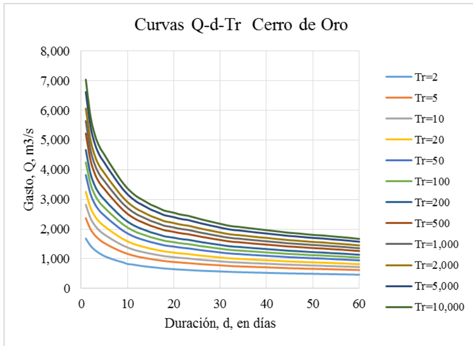
FIGURA 4.13. Curvas gasto duración periodo de retorno, Cerro de Oro
