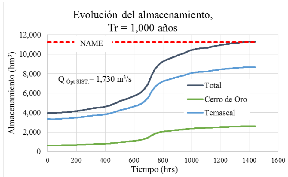
FIGURA 5.46. Evolución del almacenamiento, Tr = 1,000 años y política óptima
