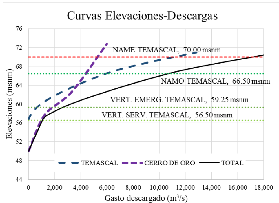
FIGURA 3.3. Curva Elevaciones-descargas del sistema de presas, De Luna (2010)
