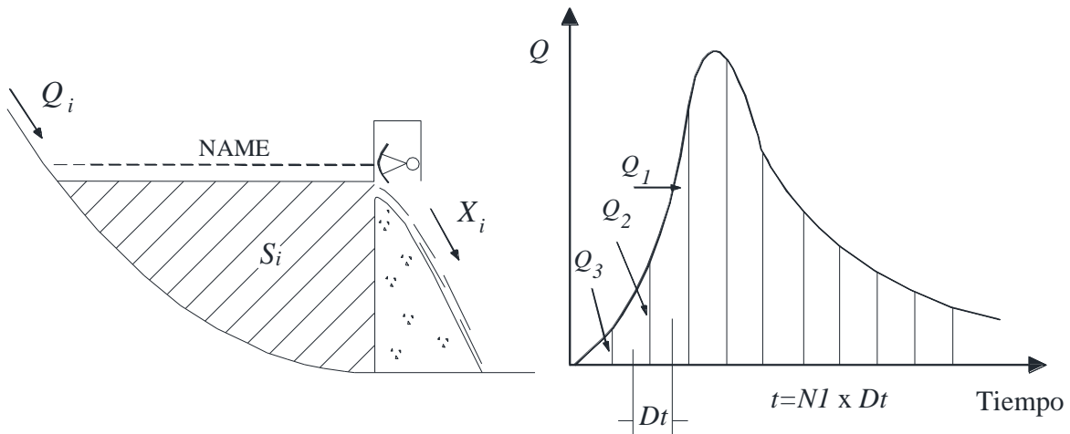
FIGURA 2.7. Esquema de la presa y vertedor
