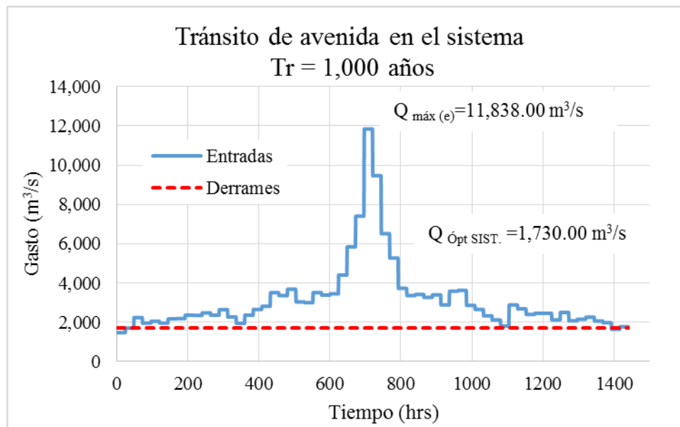
FIGURA 5.43. Tránsito de avenidas en el sistema, Tr = 1,000 años y política óptima
