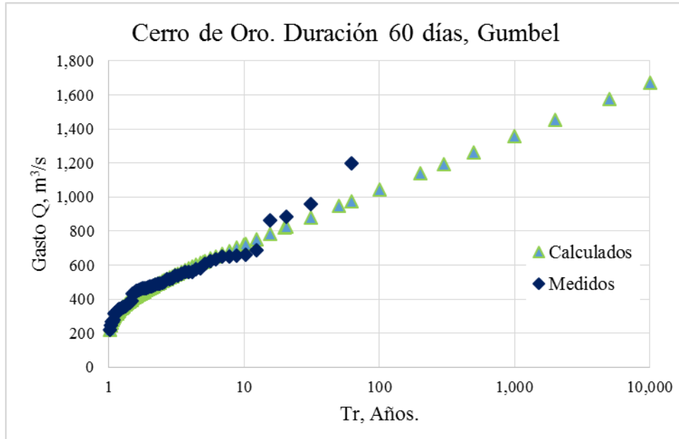
FIGURA 4.6. Ajuste de la serie de gastos con duración de 60 días, Cerro de Oro
