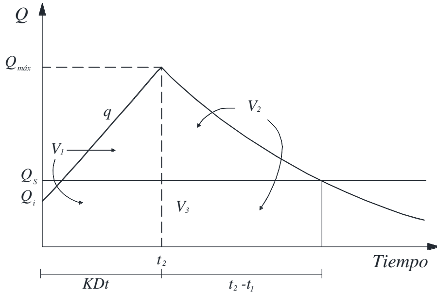
FIGURA 2.13. Hidrograma representativo de una avenida
