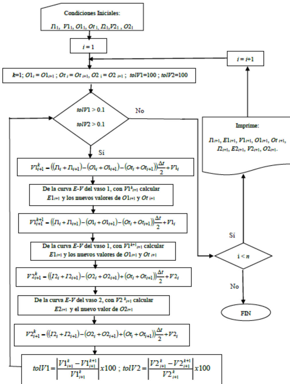
FIGURA 2.6. Diagrama de bloques, método numérico modificado
