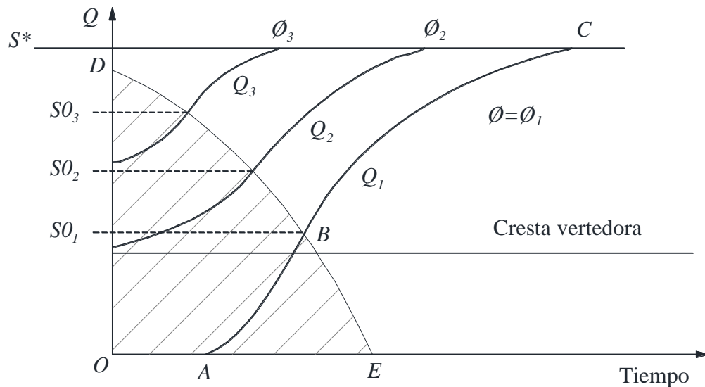
FIGURA 2.8. Evolución de los almacenamientos en el tiempo para las políticas óptimas dada una avenida de periodo de retorno Tr y considerando diferentes niveles iniciales
