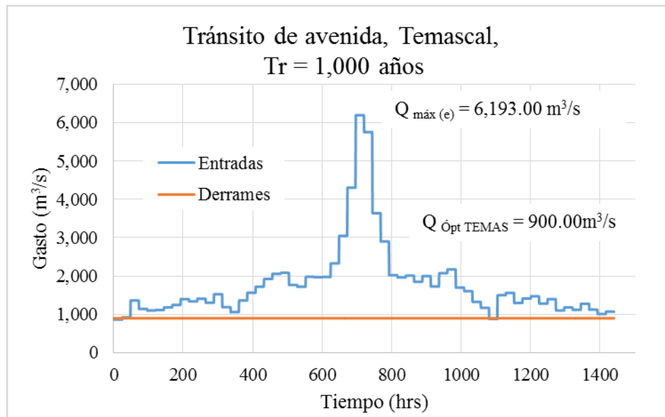
FIGURA 5.45. Tránsito de avenidas en Temascal, Tr = 1,000 años y política óptima
