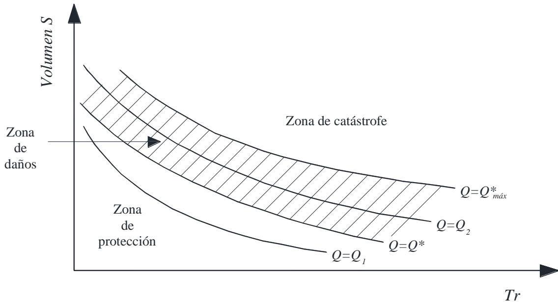
FIGURA 2.12. Gastos máximos para diferentes para diferentes almacenamientos iniciales y periodos de retorno
