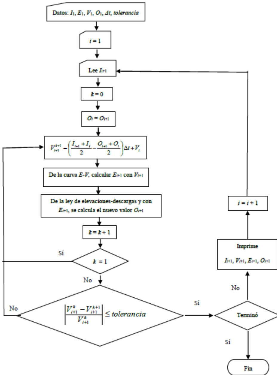
FIGURA 2.5. Diagrama de bloques, método numérico
