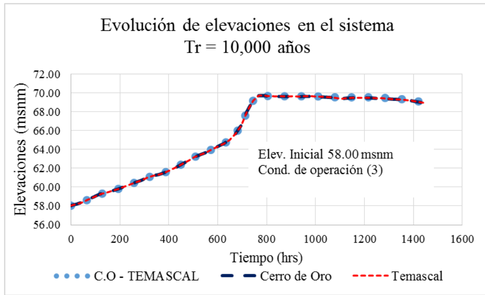
FIGURA 5.6. Evolución de elevaciones, Tr = 10,000 años, elevación inicia 58.00 msnm y condición de operación 3
