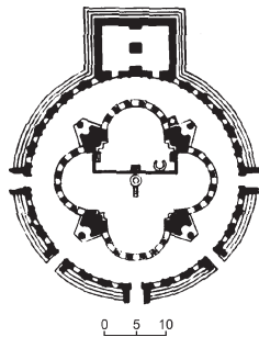
Զվարթնոց տաճարի հատակագիծը
