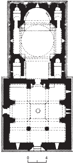
Գանձասարի վանքի հատա-կազի՞րը
