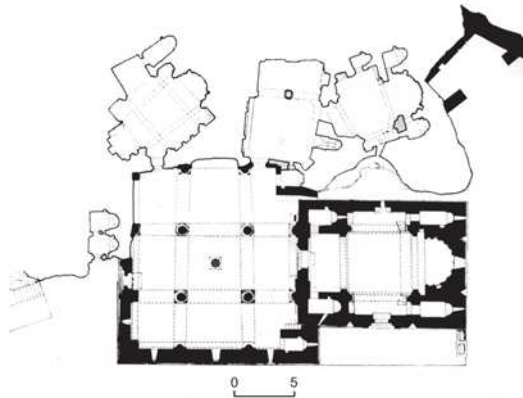
Գեղարզավանքի հատակագիծը
