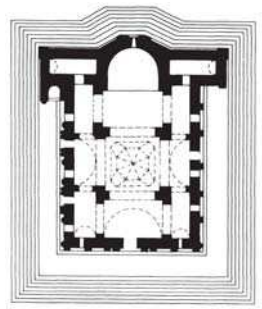
Տեկորի Ս. Երրորդութիւն վանքի Ս. Սարգիս վկայարանի հատակագիծը
