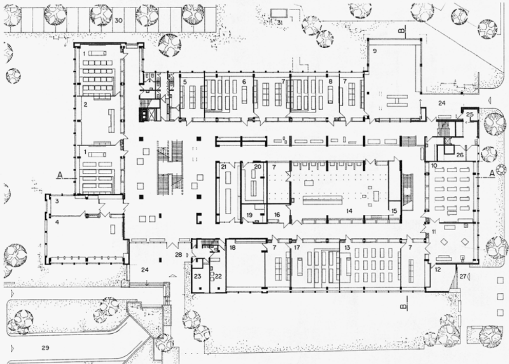
Sockelgeschoss 1:600. Legende: 1 Mechaniker, 2 Demonstrations- und Materialraum, 3 Prüfmaschine, 4 mech. Werkstatt, 5 Werkstattlehrer, 6 Bauschlosser, 7 Material, 8 Automechaniker, 9 Autolehrraum, 10 Schreiner-Werkstatt, 11 Maschinenraum Schreiner, 12 Spänerraum, 13 Schreiner, 14 Werkstatt für Spengler, Bauschlosser, Installateure, 15 Garderobe, 16 Vorbereitung, 17 Installateure, Heizungsmonteur, 18 Demonstrationsraum Heizung, Sanitär, 19 Sanitätsraum, 20 Patentschriften, 21 Verteilraum, 22 Waschküche Abwartwohnung, 23 Arbeitszimmer, 24 gedeckte Pausenhalle, 25 Abfälle, 26 Lager, 27 Aufgang zu Pausenplatz (Haupteingang), 28 Eingang Abwartwohnung, 29 Rampe zu Garage (Zivilschutzanlage), 30 Parkplatz Gewerbeschule, 31 Aussenzugang Schul-Luftschutz
