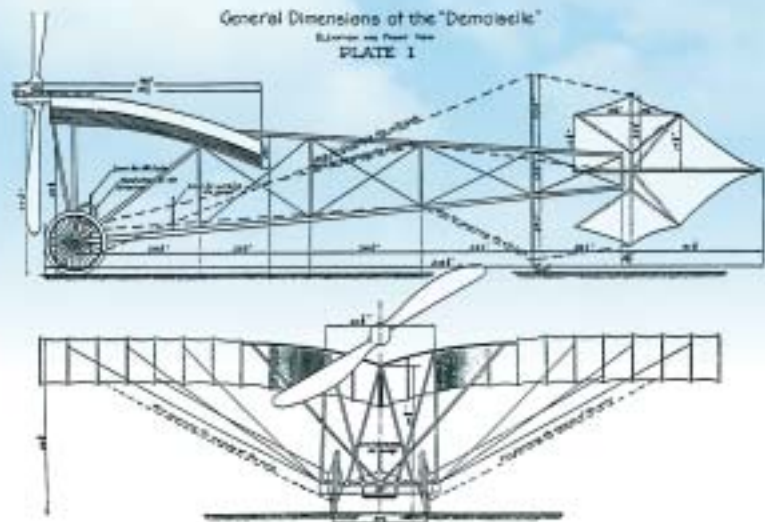
Plano do último Demoiselle, de Santos Dumont, publicado na revista Popular Mechanics de 1910.
