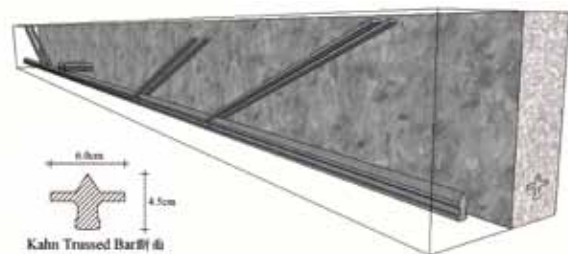
圖3 於大成館修復工程中所記錄的 Kahn Truss Bar 構造。
