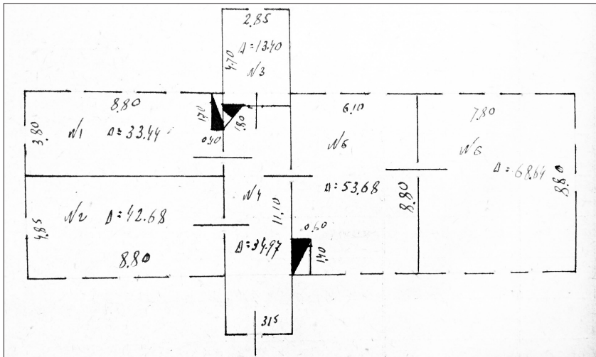
План здания бывшей немецкой церкви (1931 г.).
