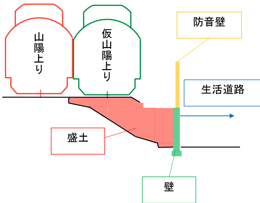
広島方を向いた断面図
