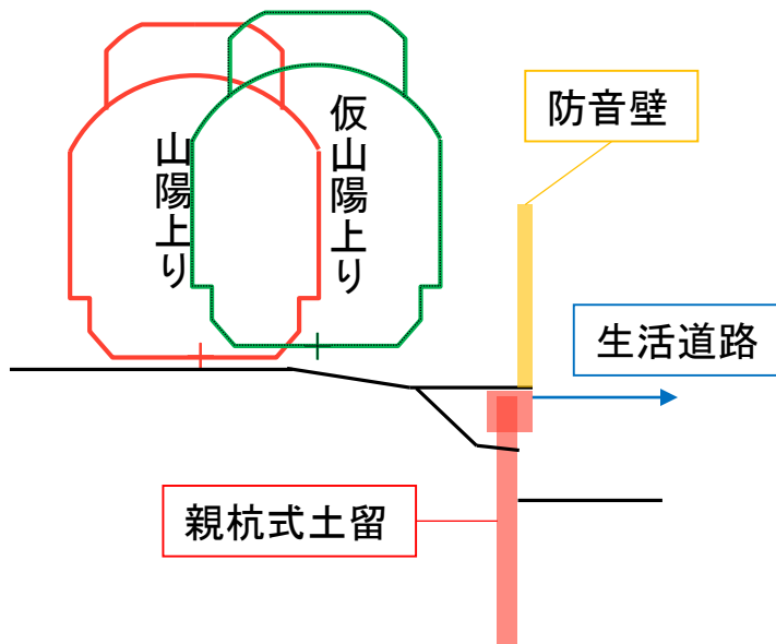
広島方を向いた断面図
