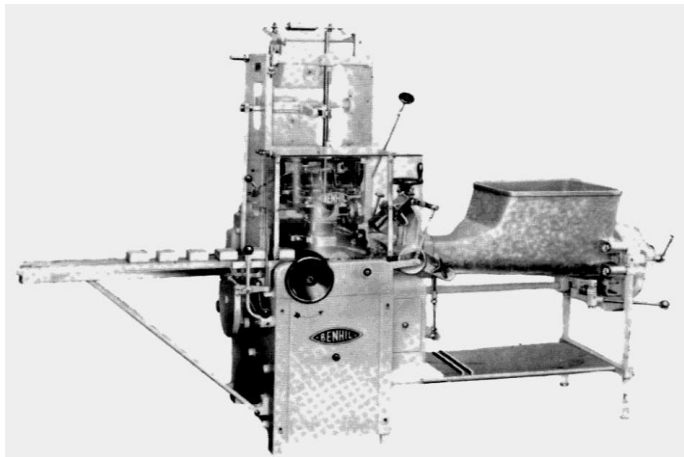
Smørpakkemaskinen "Benhil"
