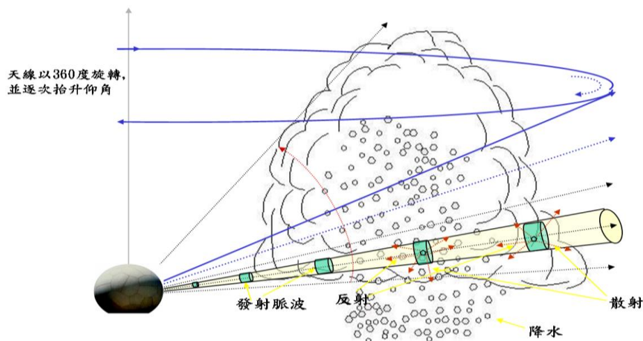
圖 16 雷達掃描觀測示意圖
