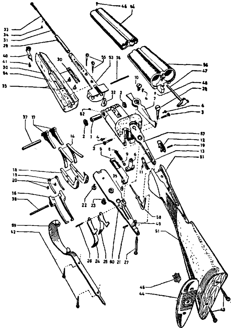
ŞEKİL — 2a Av tüfeklerinin parçaları
