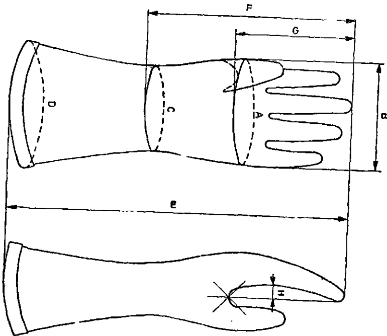
Şekil - 1 Alçak gerilim için yalıtkan lastik eldiven
