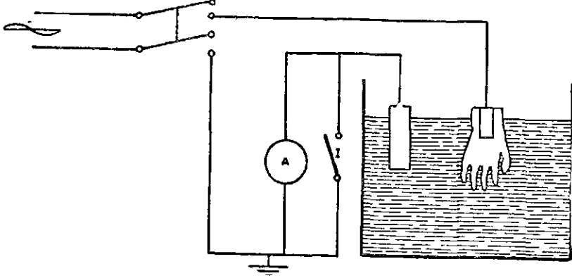
Şekil - 2 Yüksek gerilim deneyi devre şeması
