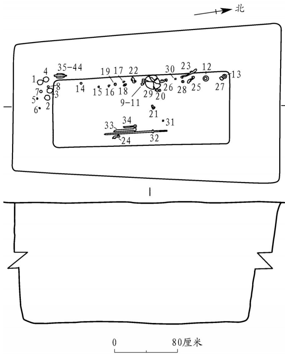
图二// M1平、剖面图
