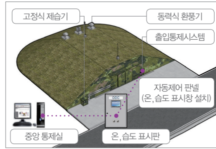
스마트탄약고(이글루형)
