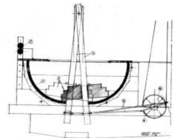
Подужни пресек ваљаре у Новом Милошеву
