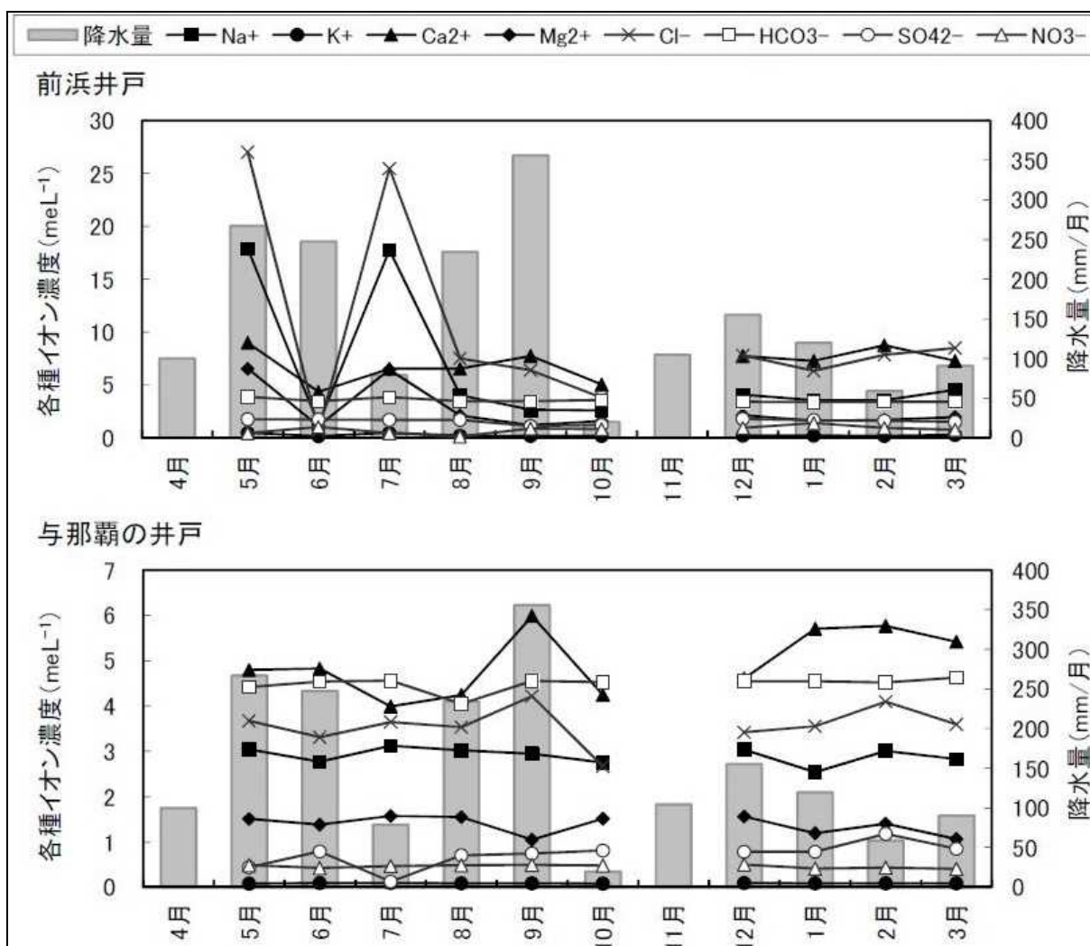
図 3.2.2-4(1) 事業実施想定区域周辺の宮古島市地下水水質保全調査結果グラフ
