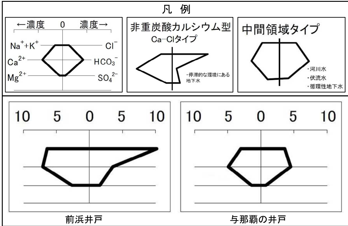
図 3. 2. 2-4(2) 事業実施想定区域周辺の宮古島市地下水水質保全調査結果ヘキサダイアグラム
