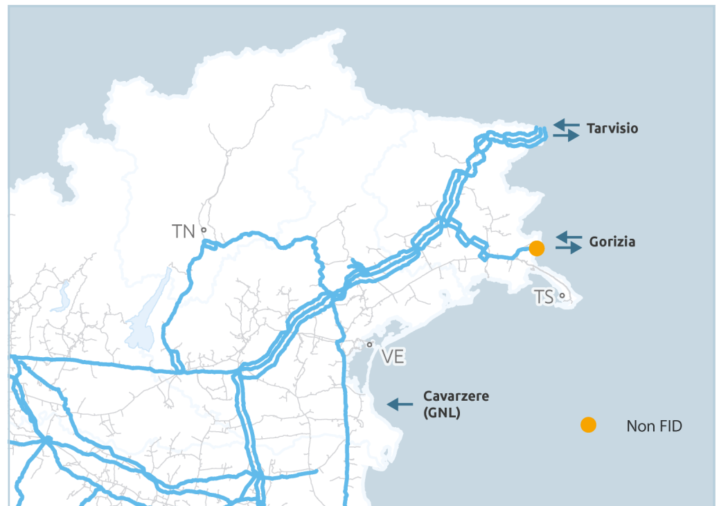
Figura 9: Potenziamento Impianto di Gorizia
