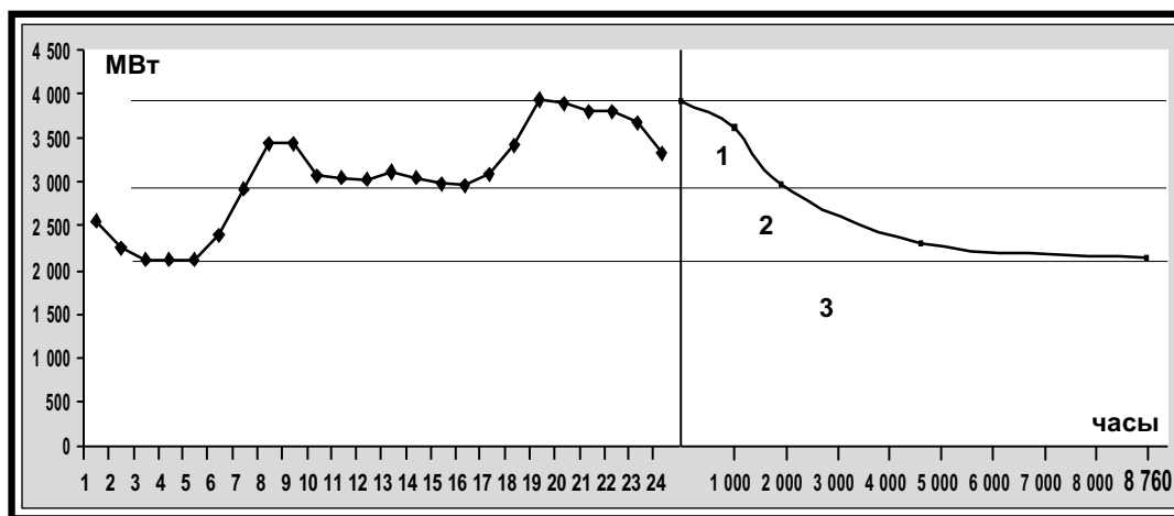
Схема перехода суточного графика нагрузки к годовому
